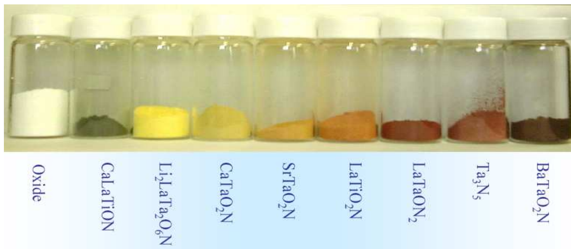
Figure 1.4. Poudres oxynitrides colorées en comparaison d'un oxyde blanc [Domen].
