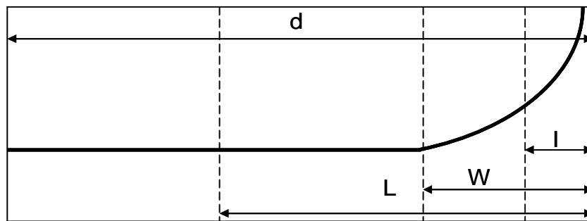
Figure 5.11. Profondeur de pénétration de la lumière l=1/\alpha , épaisseur de la zone de charge espace W , longueur de diffusion des porteurs minoritaires L et d l'épaisseur du grain [Mills].
