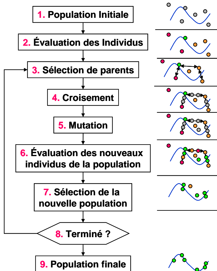
Figure 19: schéma des algorithmes génétiques
