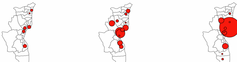
Nord et Sud Kivu, 2001, semaines 30 à 33
