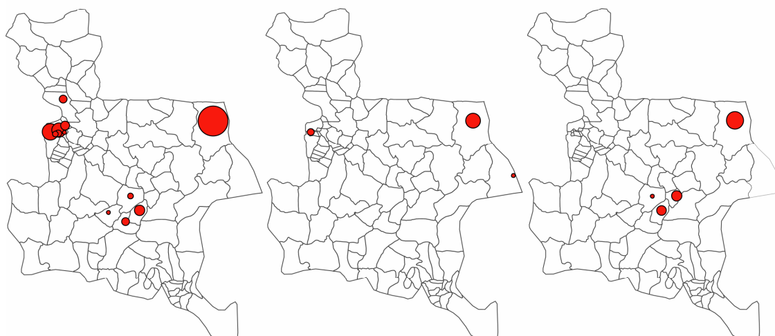
Nord et Sud Kivu, 2001, semaines 30 à 33
