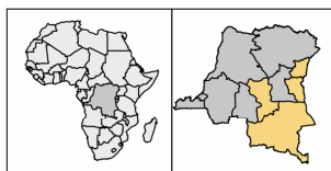
Katanga et Kasai Oriental, 2005, semaines 29 à 32
