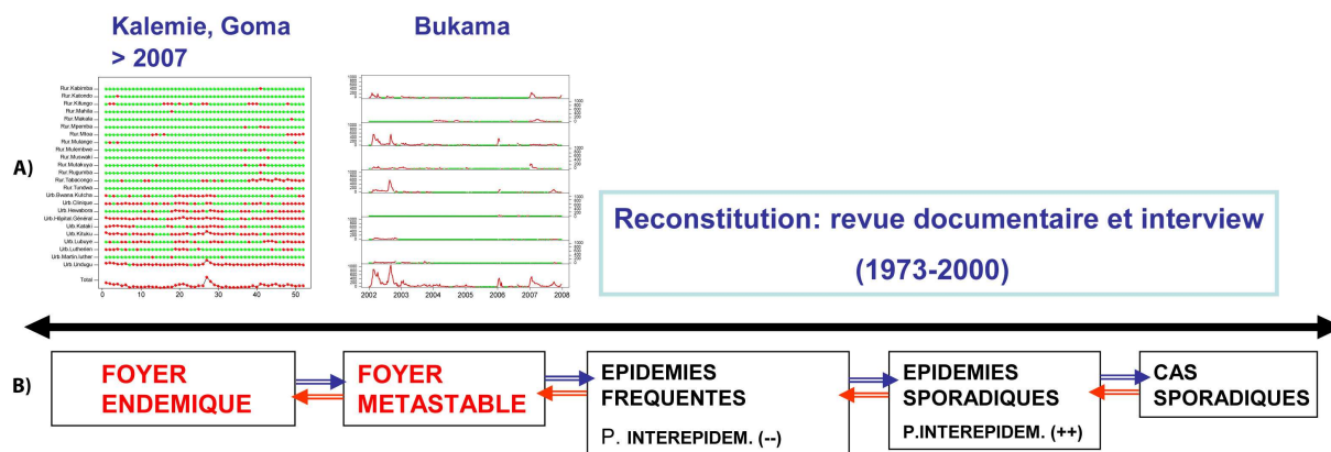
Figure 45 : (A) Evolution de la situation du choléra par foyer. (B) : Cycle des changements d'état du choléra au niveau environnemental dans la région des Grands Lacs africains.
