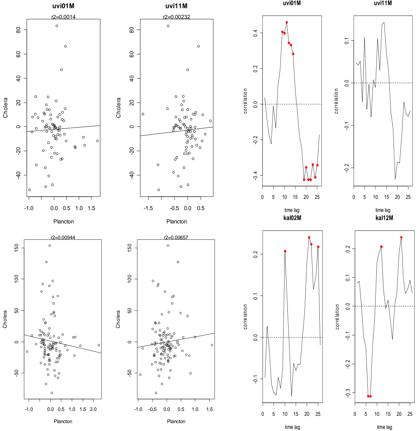
Figure 40 : Corrélations croisées entre résidus de séries de plançon (dégagés de la tendance inter-annuelle) et nombre de cas de choléra observés à Uvira (haut) et Kalemie (bas), étude sans décalage (A) et avec décalage (B)
