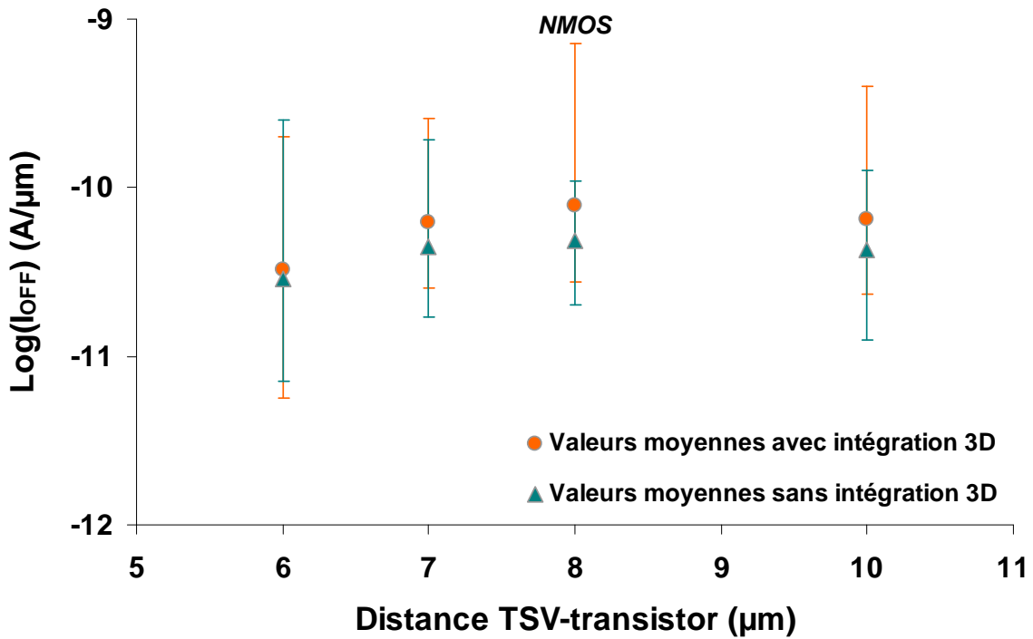
Figure 4.10. Courants de fuite moyens et dispersions associées pour les transistors NMOS de largeur de grille 0,15 μm implémentés à différentes distances du TSV. La ligne horizontale est la valeur moyenne de référence pour le courant de fuite avant intégration 3D.
