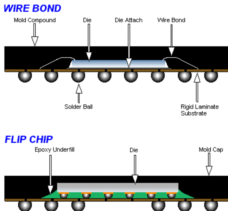
Figure 1.4. Principe de connexion par câblage ( wire bonding ) et par report ( flip chip ). (© 2001 Amkor Technology, Inc.)
