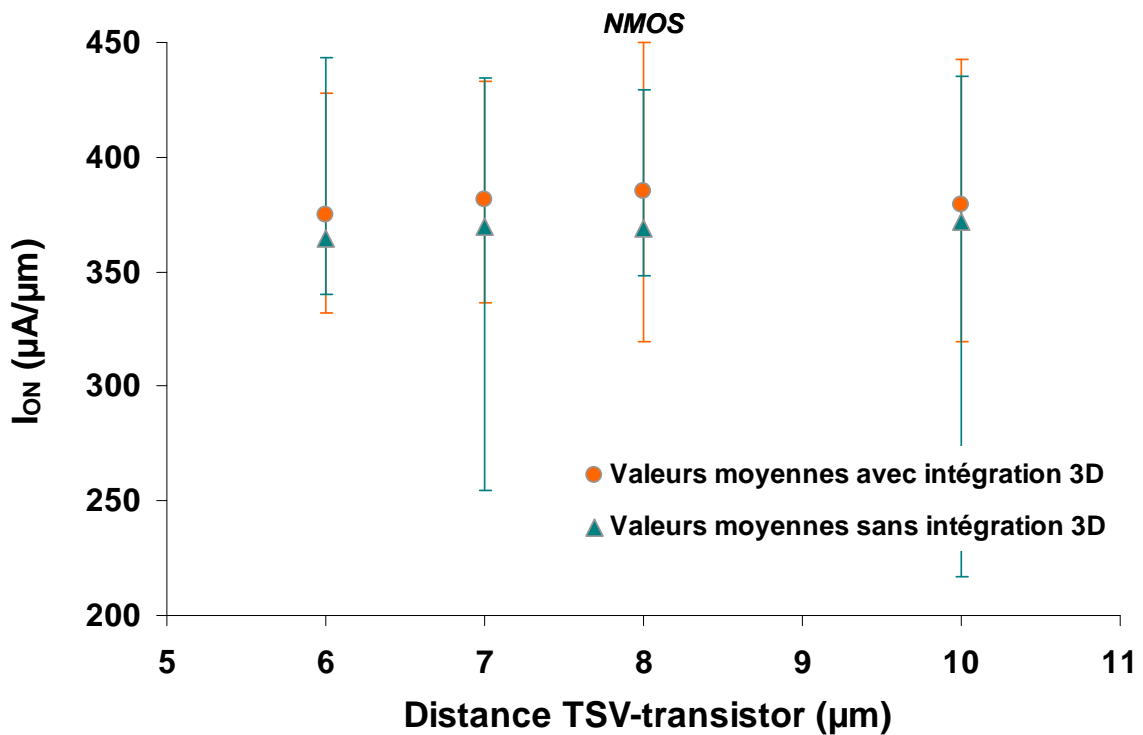
Figure 4.11. Courants de saturation moyens et dispersions associées pour les transistors NMOS de largeur de grille 0,15 μm implémentés à différentes distances du TSV. La ligne horizontale est la valeur moyenne de référence pour le courant de saturation avant intégration 3D.
