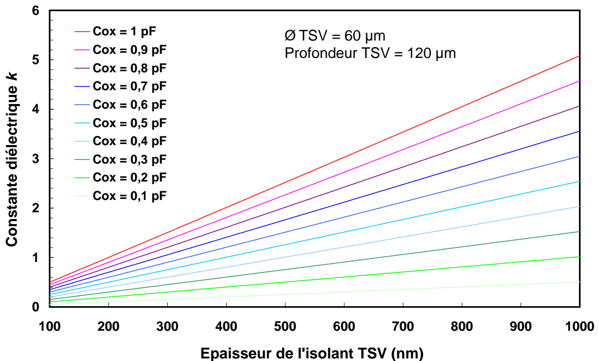
Figure B.2. Courbes iso-capacités pour un facteur de forme de 1:2 ( \varnothing 60\ \mu\text{m} ) en fonction de la constante diélectrique k de l'isolant et de son épaisseur de dépôt.
