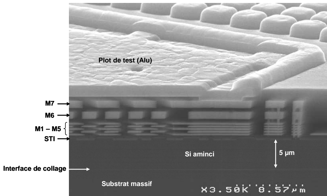
Figure 4.3. Coupe MEB de la plaque amincie à 5 μm avec visualisation de tous les niveaux BEOL et du silicium aminci sur son substrat support.
