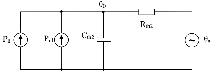
Figure 3-15 : Modèle thermique du transfert huile/air ambient
