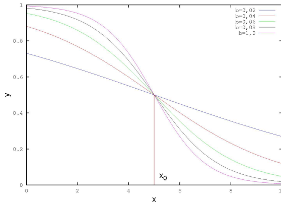
FIG. 12.5 – Tracé de quelques sigmoïdes d'équation y = \frac{1}{1 + e^{b(x-x_0)}} avec x_0 = 5 .
