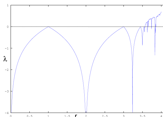
FIG. 5.7 – Estimation de l'exposant de Lyapunov pour l'application logistique en fonction du paramètre de contrôle.
