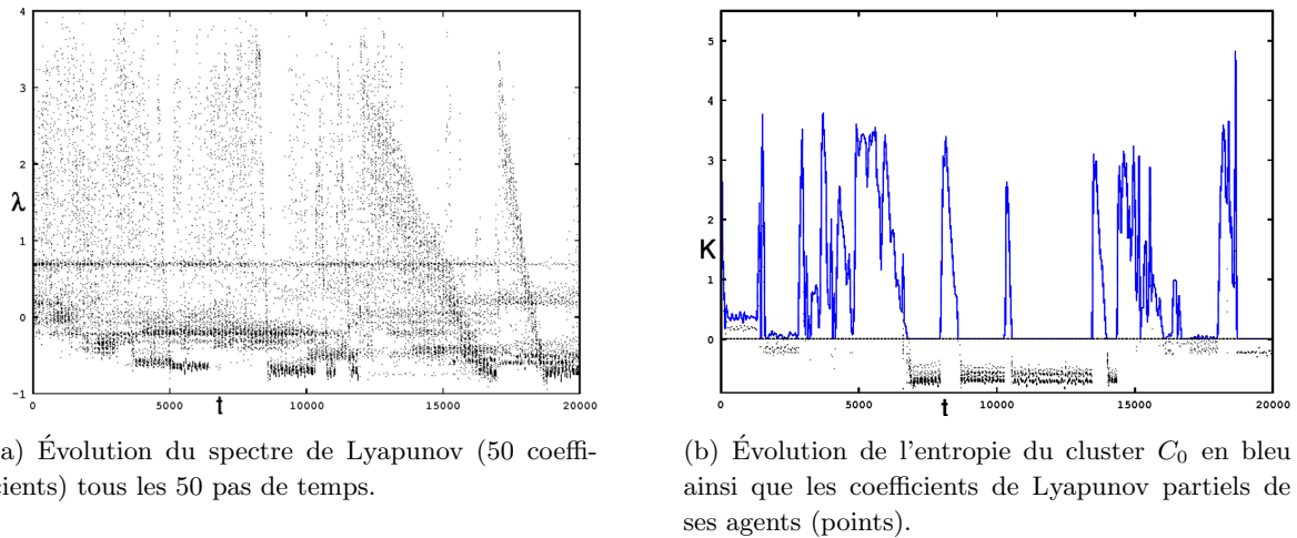
FIG. 10.9 – Spectre de Lyapunov partiel et suivi de l'entropie K du cluster C_0 en fonction du temps avec \epsilon = 0,8 . L'intervalle de temps est de 50 pas de temps à chaque évaluation.
