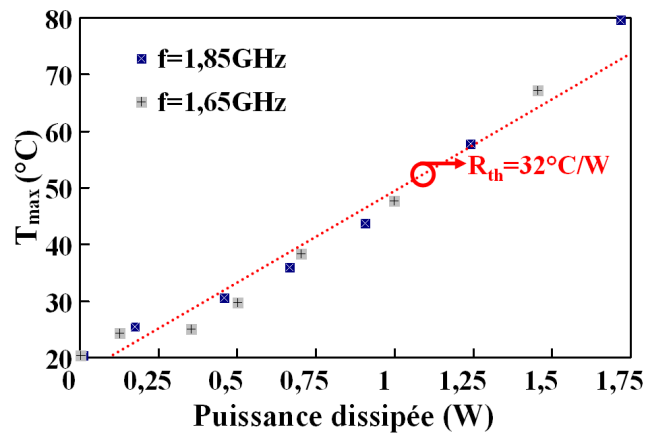
FIG.4-20: courbe de la température maximale du filtre mesurée sur le premier résonateur parallèle du filtre, les deux pentes obtenues pour deux fréquences différentes sont proches de 32°C/W
