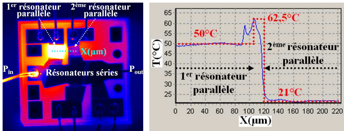
FIG.4-18: (a) Répartition de la puissance dissipée dans le filtre pour f=1,65 GHz et (b) variation de la température dans les deux résonateurs parallèles
