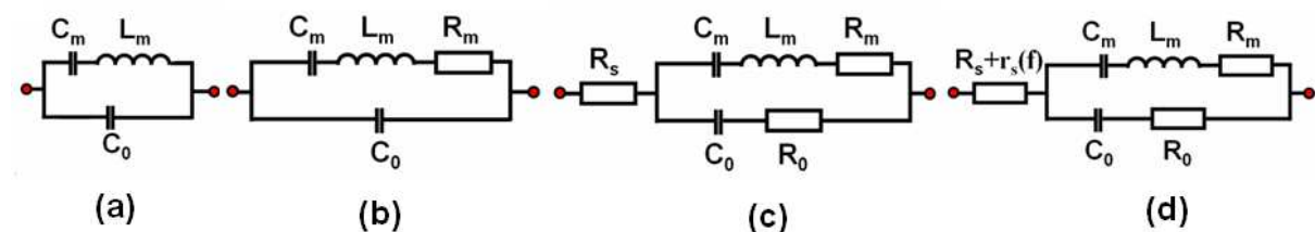
FIG.1-36: Modèle électrique équivalent pour un résonateur piézoélectrique : (a)sans pertes (b) Modèle BVD proposé par Van Dyke pour le quartz (c)avec les pertes électriques, diélectriques et mécaniques du BAW (d) avec les pertes acoustiques dues aux modes latéraux
