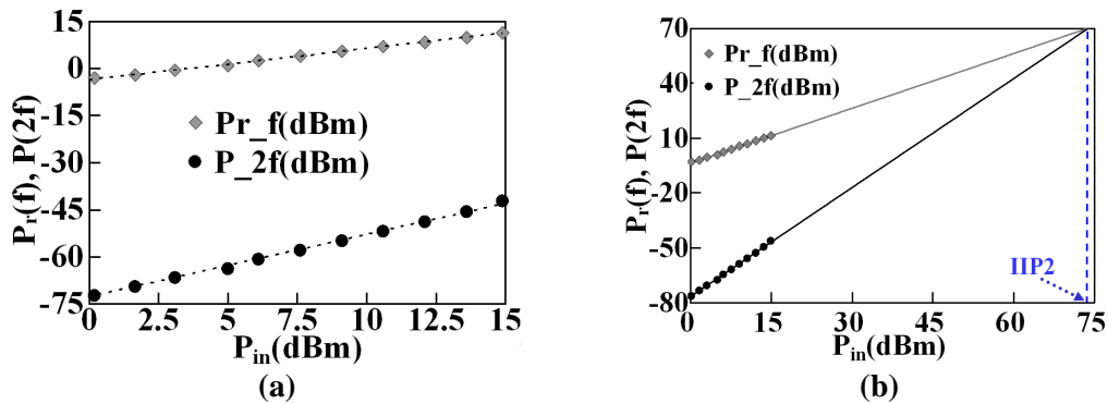
FIG.3-29: (a) Variation de la puissance réfléchie à f_{max} et la puissance générée à 2f_{max} en fonction de l'amplitude du signal d'entrée à une fréquence constante f=f_{max} , (b) Détermination du point d'interception d'ordre 2 IIP2 à 73dBm par interpolation des points expérimentaux
