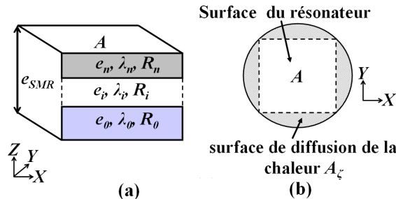
FIG.3-16:(a) l'empilement multicouche considéré pour l'étude avec les paramètres de chaque couche, (b) la surface effective de la diffusion de la chaleur dans un SMR (en vue de dessus) et le système de coordonnées
