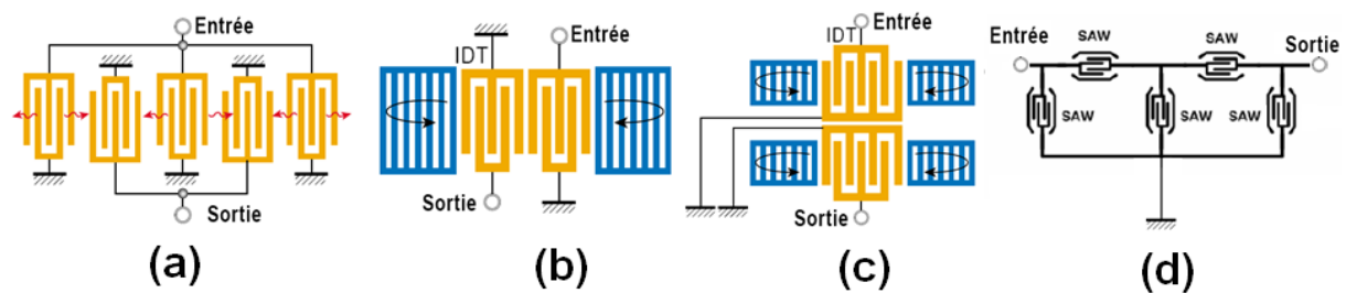
FIG.1-9: Vue supérieure de quelques structures de base des filtres SAW [R.1.31-R.1.72] :(a) IIDT (b) DMS à Couplage longitudinal (c) DMS à Couplage transverse et (d) filtre SAW à résonateurs en échelle d'ordre 5 (en jaune les transducteurs, en bleu les parois réfléchissantes)
