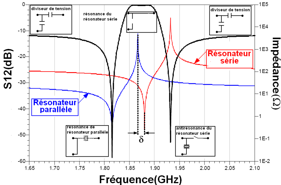
FIG.1-31: Principe de fonctionnement d'un filtre en échelle
