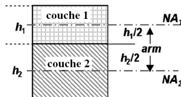
FIG.3-49:Schéma d'une bicouche
