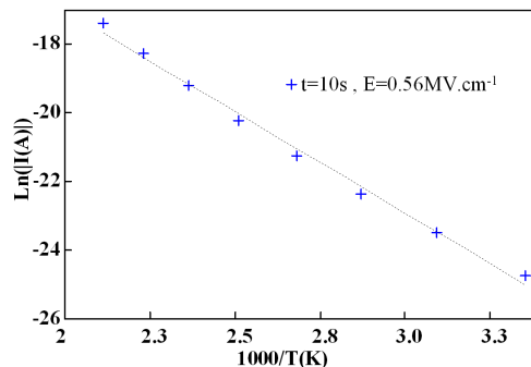
FIG.2-11: Variation du courant de décharge dans l'AlN en fonction de la température pour t et E fixés
