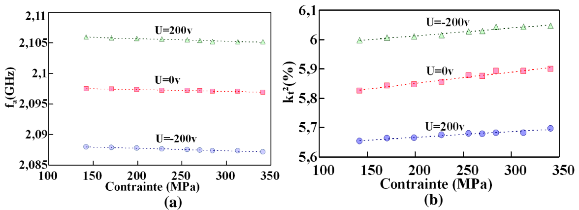
FIG.3-9 : Variation de (a) la fréquence d'antirésonance et (b) du facteur de couplage k_r^2 d'un SMR en fonction de la contrainte mécanique à tension constante
