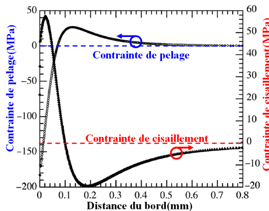
FIG.3-42: Exemple de calcul de la contrainte normale de pelage et de la contrainte de cisaillement par éléments finis ABAQUS, ces deux contraintes atteignent leur maximum (en valeur absolue) au bord de la structure tandis que loin du bord elles tendent rapidement vers zéro [R.3.208]
