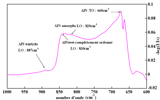
FIG.2-12 : Analyse IR de la surface d'un échantillon AlN/Mo/Si : en plus de l'AlN Wurtzite, nous remarquons la présence de l'AlN qui n'est pas complètement ordonné ainsi que des régions d'AlN amorphe
