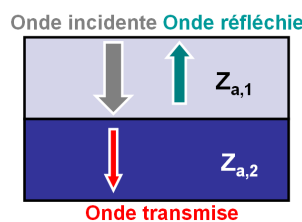
FIG.1-17: Réflexion d'une onde acoustique sur une interface entre deux matériaux d'impédances acoustiques différentes
