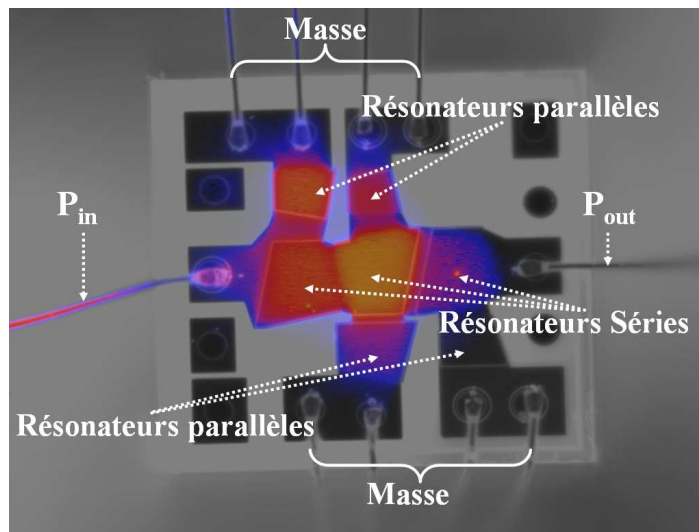
FIG.4-16: Image thermique d'un filtre BAW obtenue par la technique de thermographie modulée à une fréquence de 25Hz pour P_{in}=31dBm et f=1,815GHz qui correspond au pic de dissipation de puissance
