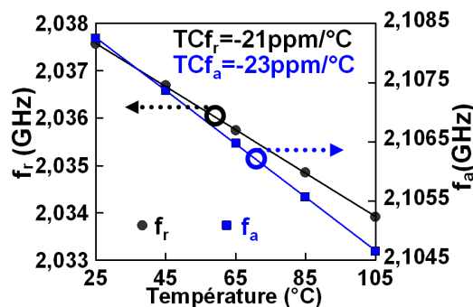
FIG.3-26: Mesure de la variation en température de f_r et f_a pour extraire le TCf_r et le TCf_a
