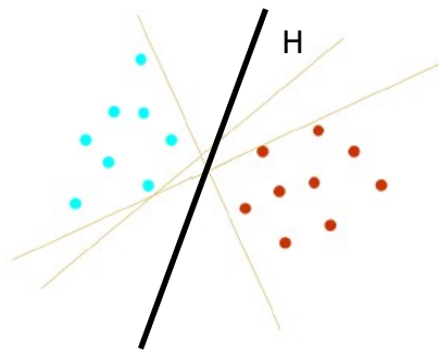
FIG. 2.5 – Exemple d'un SVM linéaire
