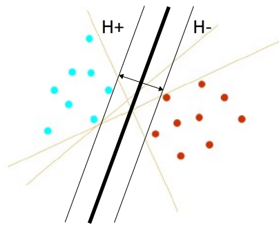
FIG. 2.6 – Exemple de marge d'un SVM linéaire
