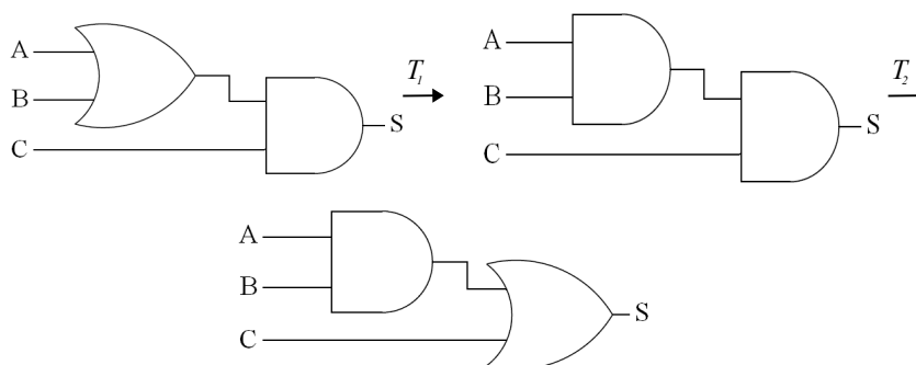
FIG. 5.8 – Exemple d'application de l'algorithme « Graph Edit Distance » entre schémas électroniques
