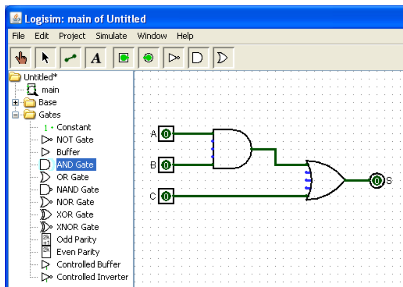
FIG. 3.5 – Interface de l’outil LogiSim
