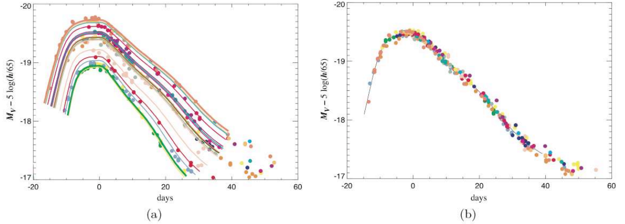
FIGURE 5.2 – La figure de gauche montre les courbes de lumière des supernovæ observées par le Cal-n-Tololo Supernovæ Search [Hamuy et al. 1993] dans la bande B. La figure de droite représente les mêmes courbes de lumière corrigées à l’aide du paramètre d’étirement (“stretch factor”). Cette correction permet de passer d’une dispersion de l’ordre de 50% de la luminosité intrinsèque des SNe Ia à un peu moins de 20%.
