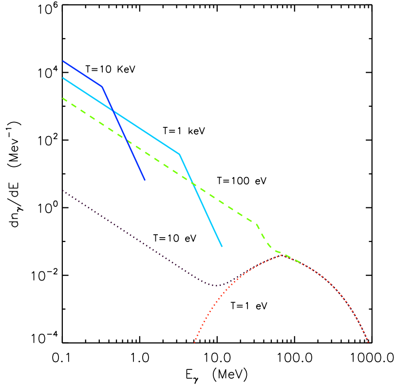
FIGURE 4.12 – Spectres des photons résultant des annihilations p\bar{p} à différentes températures. Les courbes bleues représentent les spectres de cascades à une température de 1 keV et 10 keV. Pour une température de 1 eV, l'énergie seuil est largement supérieure à l'énergie des photons d'annihilation et le spectre des photons garde sa forme initiale. Pour des énergies intermédiaires, la partie du spectre supérieure à l'énergie seuil est redistribuée selon le spectre de cascade.
