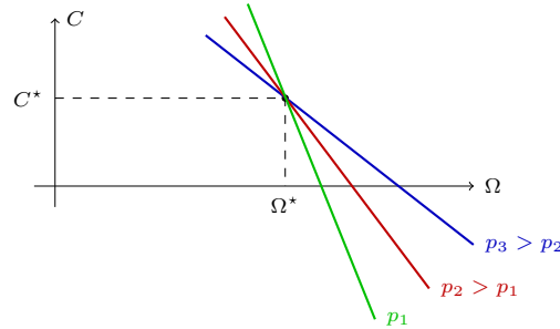
Figure 5.16 – Position des courbes couple-vitesse autour du point de consigne ( C^* ; \Omega^* ) en fonction du nombre de paires de pôles. L'alimentation ( v_s ; f_s ) est optimisée pour minimiser les pertes de fonctionnement.
