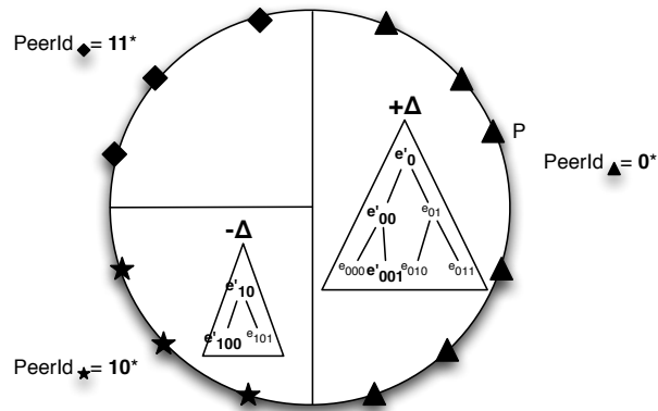
(b) Après le rafraîchissement, tous les pairs de e'_0 et e'_{10} ont mis à jour leur arbre de fragmentation. Les pairs de e'_{11} ne connaissent pas la valeur \Delta utilisée.
