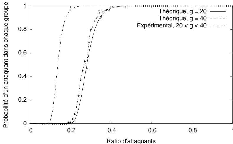
FIGURE 5.2 – Probabilité qu'il y ait un attaquant dans chaque groupe en fonction du ratio d'attaquants, dans un réseau composé de 10 000 pairs. Les deux courbes théoriques correspondent à des groupes de fragmentation composés respectivement de 20 et 40 membres et la courbe expérimentale est réalisée avec des groupes de taille comprise entre 20 et 40 membres.
