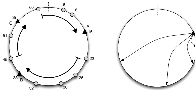
(a) Assignation des ressources aux pairs dans Chord. Ici, les ressources 60, 6 et 8 sont assignées au pair A. (b) Ensemble des raccourcis contenus dans la finger table du pair A.
