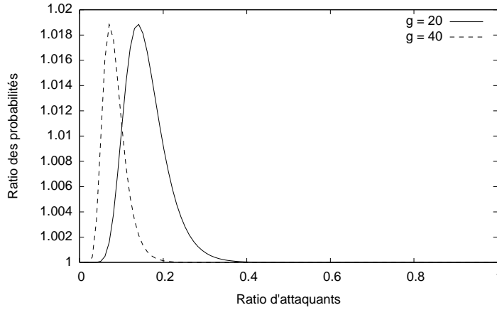
FIGURE 4.6 – Rapport entre les probabilités qu’un groupe d’attaquants connaisse un fragment dans un système idéal et dans notre système, pour des groupes de 20 ou 40 membres et après 20 rafraîchissements.
