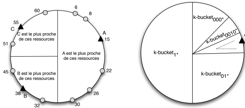
(a) Assignation des ressources aux pairs dans Kademlia. Ici, c'est le pair C qui est le plus proche des ressources 51 et 60. (b) Table de routage du pair A. Chaque k -bucket contient k pairs situés dans l'autre moitié de l' overlay , l'autre quart, etc.
