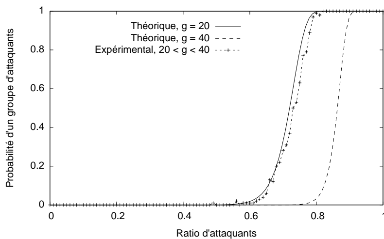
FIGURE 5.4 – Probabilité qu'un groupe ne soit composé que d'attaquants en fonction du ratio d'attaquants, dans un réseau composé de 10 000 pairs. Les deux courbes théoriques correspondent à des groupes de fragmentation composés respectivement de 20 et 40 membres et la courbe expérimentale est réalisée avec des groupes de taille comprise entre 20 et 40 membres.
