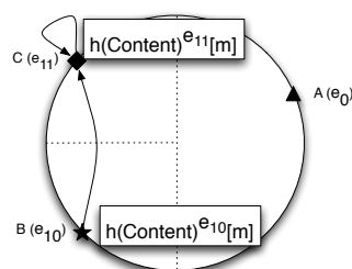
(b) B et C réalisent leurs signatures partielles avec e_{10} et e_{11}
