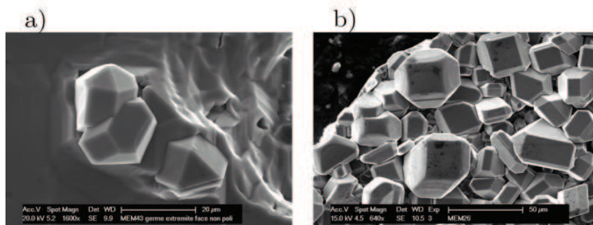
Figure IV.24 – Cristaux spontanés de 3C-SiC dont la taille est inférieure à 20\ \mu\text{m} . Pour cette taille, la forme d'équilibre est atteinte, l'anisotropie n'est pas constatée quel que soit le solvant. a) Croissance dans Si pur à 1600^\circ\text{C} . b) Croissance dans \text{Si}_{0,73}\text{Ti}_{0,27} à 1550^\circ\text{C} .
