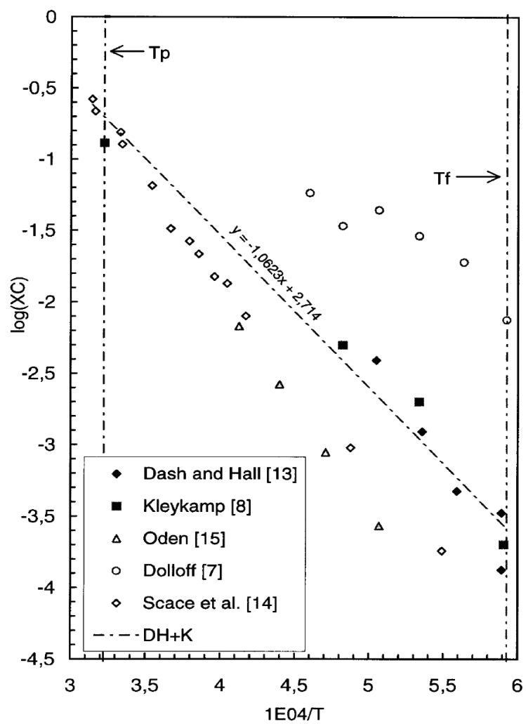
Figure II.5 – Evolution de la solubilité du carbone dans Si liquide, tiré de [99].
