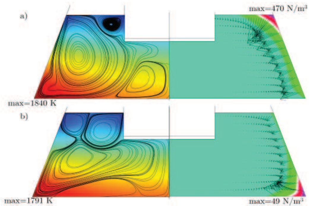
Figure III.19 – Effet de l'écran magnétique en niobium sur la température et les mouvements de convection dans le liquide. a) sans le cylindre Nb b) avec le cylindre Nb. La partie gauche montre la répartition de température (surface) et les boucles de convection (lignes de courant). La partie droite représente le module des forces électromagnétiques (surface) ainsi que l'amplitude et la direction de ces forces (flèches).
