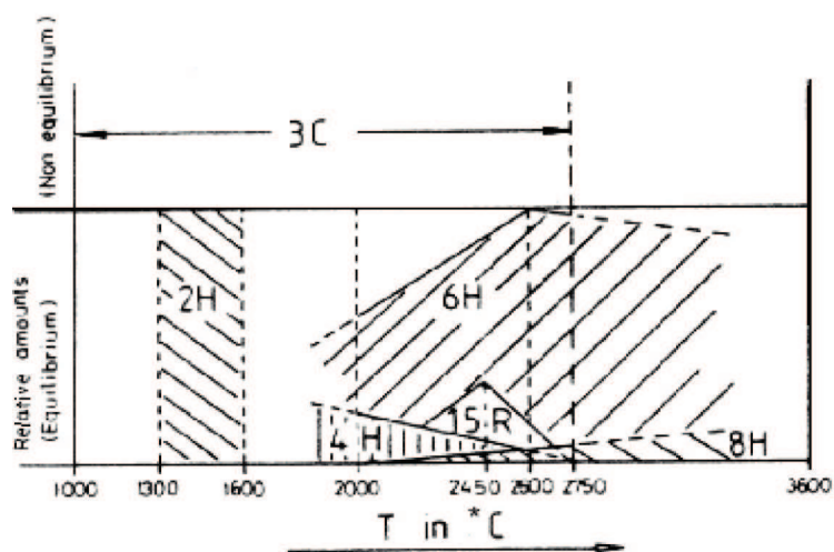
Figure I.5 – Diagramme de stabilité des polytypes du SiC en fonction de la température et de l'écart à l'équilibre, tiré de [13].
