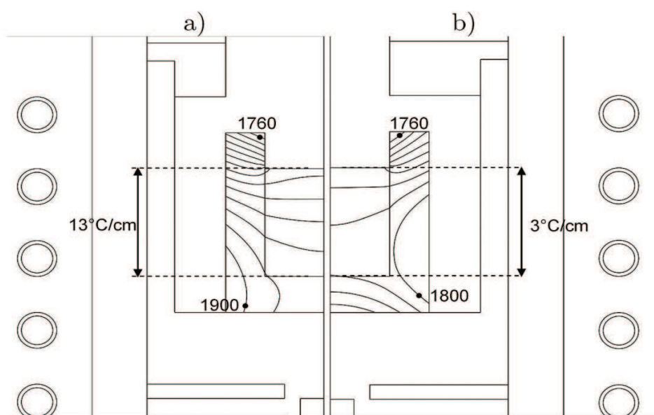
Figure III.10 – Effet de l'écran thermique sur le gradient thermique dans le liquide. a) Configuration faible gradient : Isothermes séparées de 10°C. Gradient thermique dans le liquide de 13°C/cm. I_0=320 A. b) Configuration quasi isotherme : Isothermes séparées de 5°C. Gradient thermique dans le liquide de 3°C/cm. I_0=270 A. Les températures mini et maxi du creuset en graphite sont données en Kelvin.
