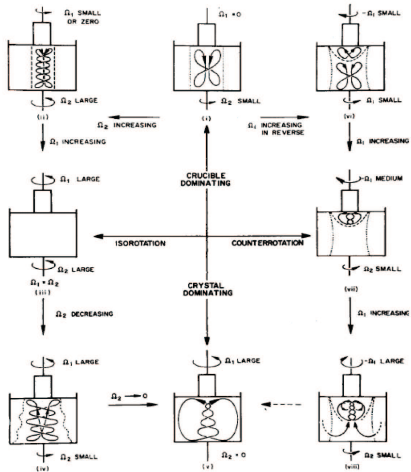
Figure II.12 – Evolution des mouvements de convection forcée suivant l'amplitude et la direction de la rotation du cristal et du creuset, tiré de [126]
