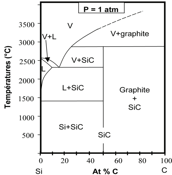
Figure I.7 – Diagramme de phase Si-C, retracé d'après [45].
