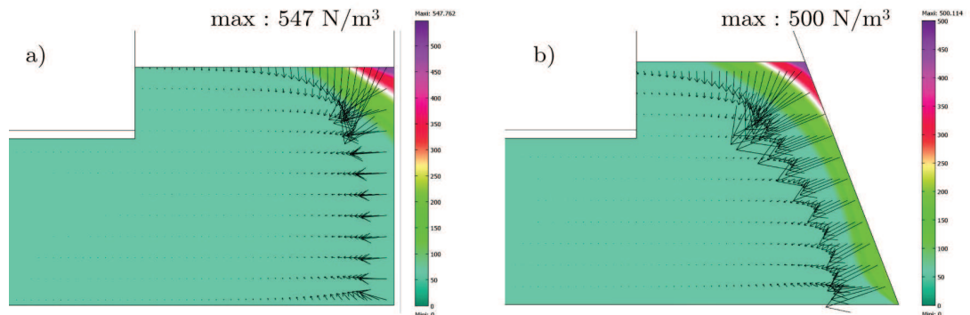
Figure III.14 – Forces électromagnétiques agissant sur le fluide. a) en creuset cylindrique, les forces agissent perpendiculairement à la paroi. b) en creuset incliné, les forces électromagnétiques ont une composante axiale dirigée vers le bas.
