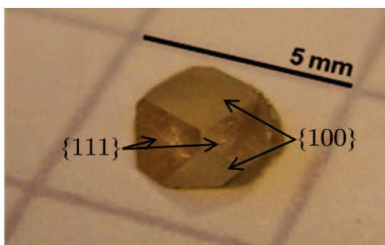
Figure IV.8 – Photographie d'un cristal 3C-SiC élaboré par CF-PVT. Facettes \{111\} et \{100\} visibles.
