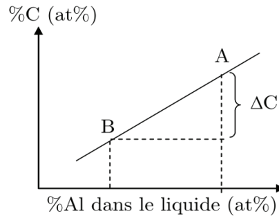
Figure IV.16 – Représentation schématique de la variation de la concentration en carbone dissout en fonction de la teneur en aluminium dans le bain. Cette variation présente à la surface du liquide du fait d’une évaporation préférentielle de l’aluminium génère une sursaturation additionnelle. Les points A et B correspondent respectivement à la composition au cœur du liquide et à la composition à la surface du liquide.
