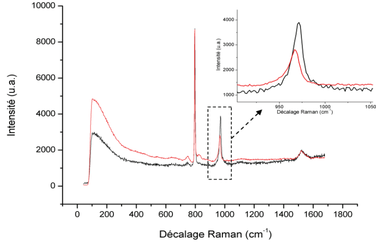
Figure V.23 – Spectre Raman de 3C-SiC à deux dopages p différents. Le cristal correspondant à la courbe rouge a un dopage p supérieur à celui de la courbe noire.
