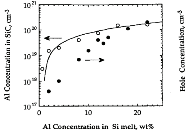
Figure V.25 – Concentration en aluminium et concentration en trous (300 K) en fonction de la teneur en aluminium. Croissance à 1600°C sur 6H-SiC on axis, polarité silicium. La courbe est calculée pour k_{ef}=0,02 , tiré de [68].
