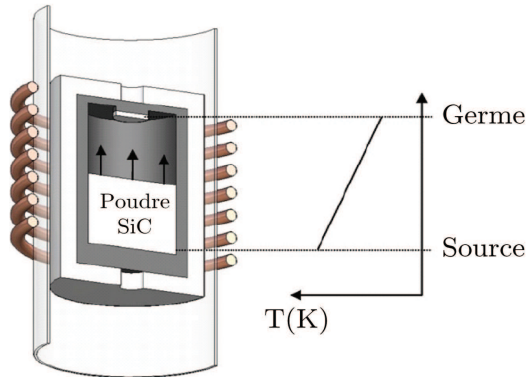
Figure I.8 – Procédé de sublimation ou PVT (Physical Vapor Transport), d'après [53].
