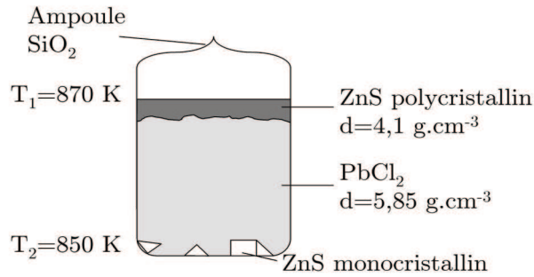
Figure II.4 – Croissance de sulfure de zinc (ZnS) par la méthode du transport par gradient thermique, d’après [98].
