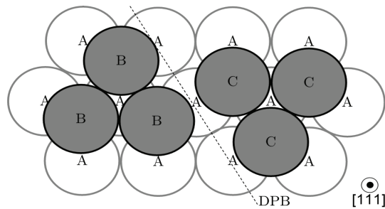
Figure V.7 – Paroi de double positionnement selon l’axe [111] . Les lettres A, B, C indiquent les positions des plans atomiques.
