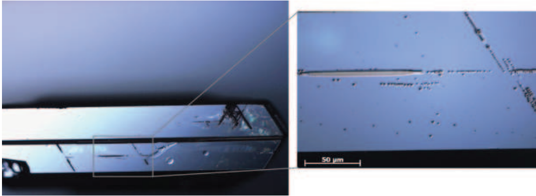
Figure V.14 – Evaluation de la densité de dislocations à partir de l'imagerie au microscope optique à contraste interférentiel. Observation de la face (111)_{Si} d'un cristal de 3C=SiC après attaque KOH à 530^{\circ}C pendant 2 minutes. La densité de dislocations sur la zone agrandie est de 3 \times 10^5 \text{ cm}^{-2} . Croissance spontanée dans Si à 1650^{\circ}C .
