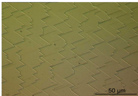
Figure IV.7 – Surface brute de croissance d'un germe 3C-SiC VLS observée au microscope optique à contraste interférentiel différentiel, d'après [44].
