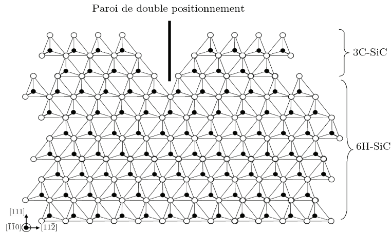
Figure V.6 – Représentation d’une paroi de double positionnement (DPB).
