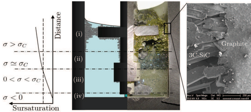
Figure IV.15 – Représentation schématique (gauche) et photographie (centre) de la localisation de la cristallisation. L'étendue de la cristallisation peut être reliée à la sursaturation ( \sigma ), \sigma_C étant la sursaturation critique. (i) : zone de cristallisation, la taille des cristaux varie entre 100 \mu\text{m} et 1 \text{mm} . (ii) : zone intermédiaire, la taille est homogène, de l'ordre de 20 \mu\text{m} . (iii) : zone sans cristallisation. (iv) : zone de dissolution. A droite, l'imagerie par microscopie électronique à balayage de la zone (i) montre l'orientation des cristaux. Croissance dans \text{Si}_{0,73}\text{Ti}_{0,27} à 1600^\circ\text{C} pendant 3 heures.
