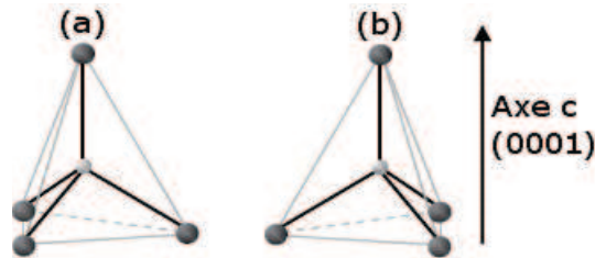
Figure I.1 – Tétraèdres réguliers dans lesquels chaque atome de silicium (carbone) est lié à 4 atomes de carbone (silicium). Une rotation de 60^\circ permet de passer d’un tétraèdre droit (a) à un tétraèdre gauche (b).
