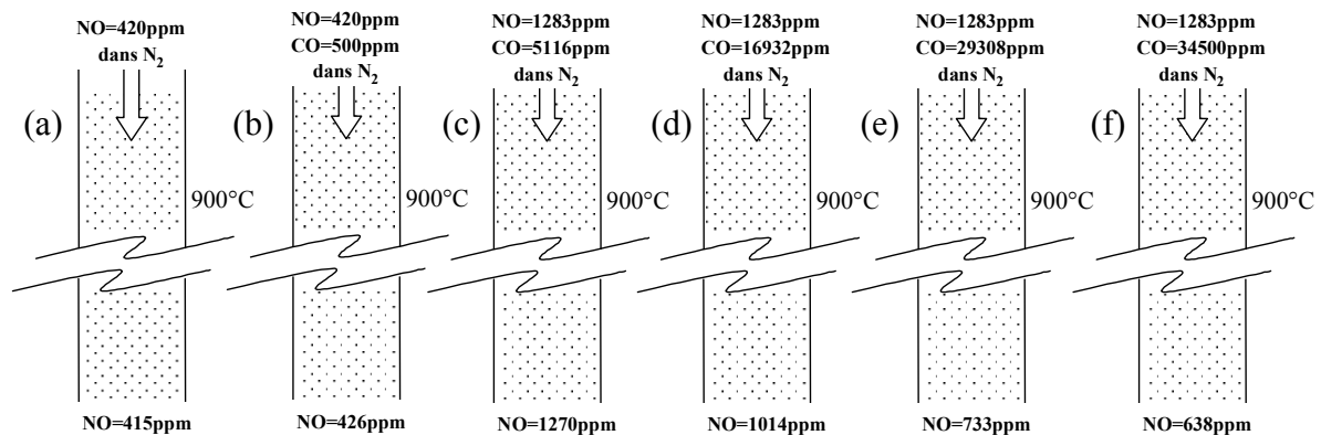
Figure IV.3-2 : Injection dans le réacteur à 900°C de (a) NO dans N 2 , et (b), (c), (d), (e), (f) de NO+CO dans N 2 et échantillonnage après un temps de séjour de 2,51s
