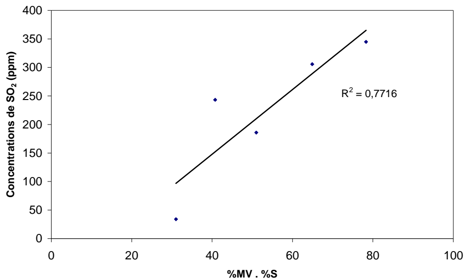
Figure IV.2-4 : Emissions de SO 2 en fonction du produit %MV.%S
