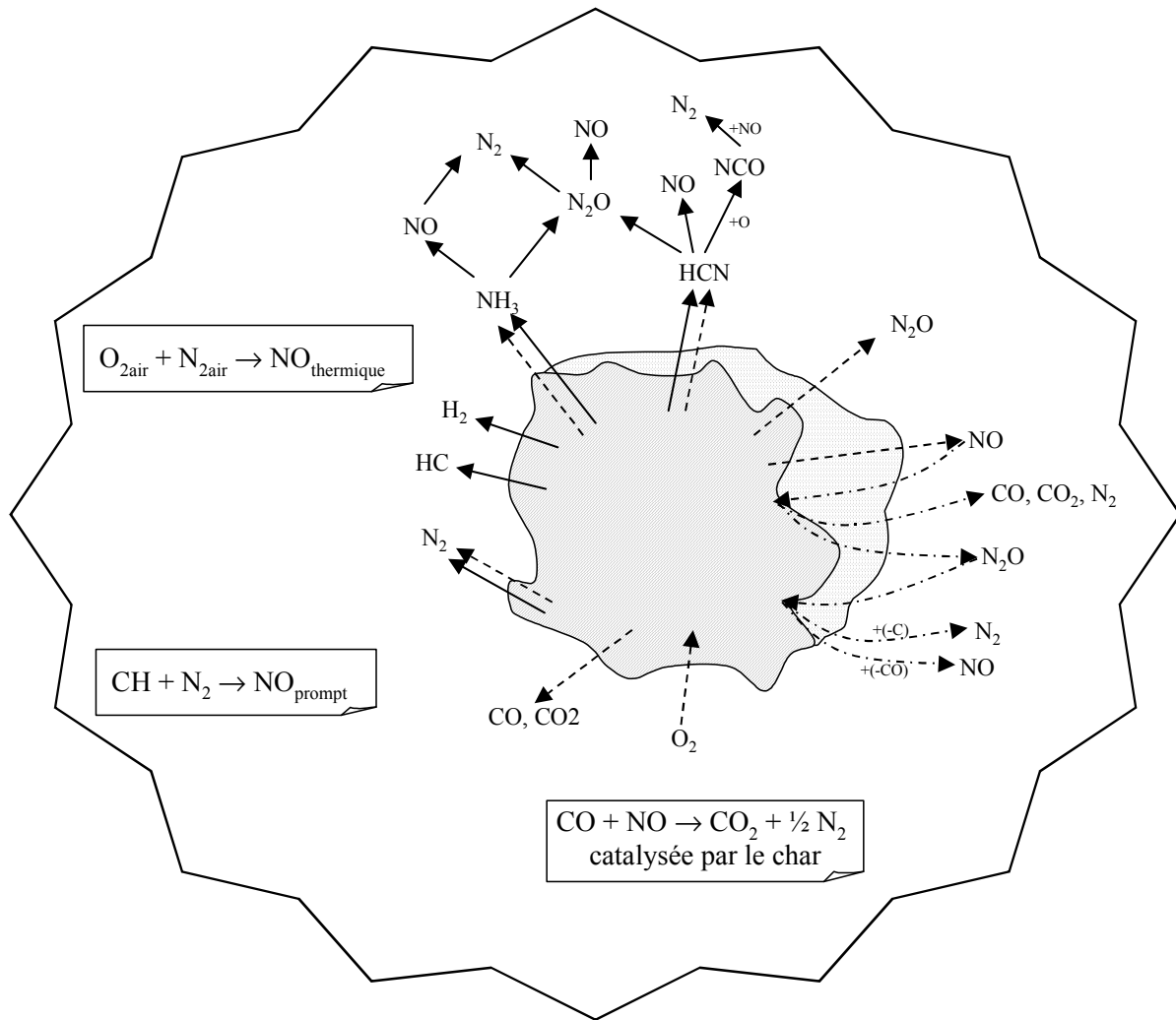
Figure II.2-2 : Réactions de formation et de destruction des oxydes d'azote : (—) pendant la dévolatilisation, (--) pendant l'oxydation du char ; (-·-) réactions hétérogènes
