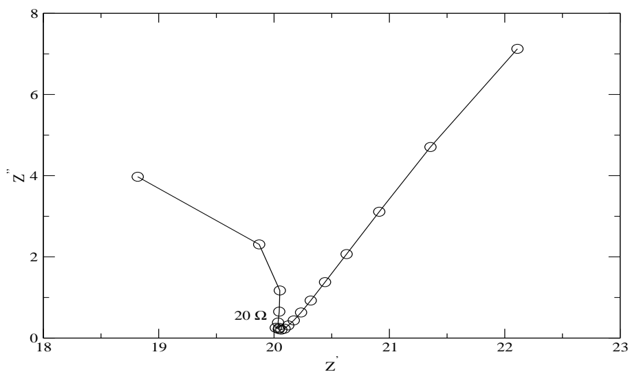
Figure 7.31: Spectre d'impédance de la membrane AW dans la cellule de mercure pour C_T = 1\text{N} et X_{NO_3^-} = 0
