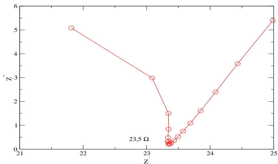
Figure 7.28: Spectre d'impédance de la membrane AW dans la cellule de mercure pour C_T = 0,5N et X_{NO_3^-} = 0
