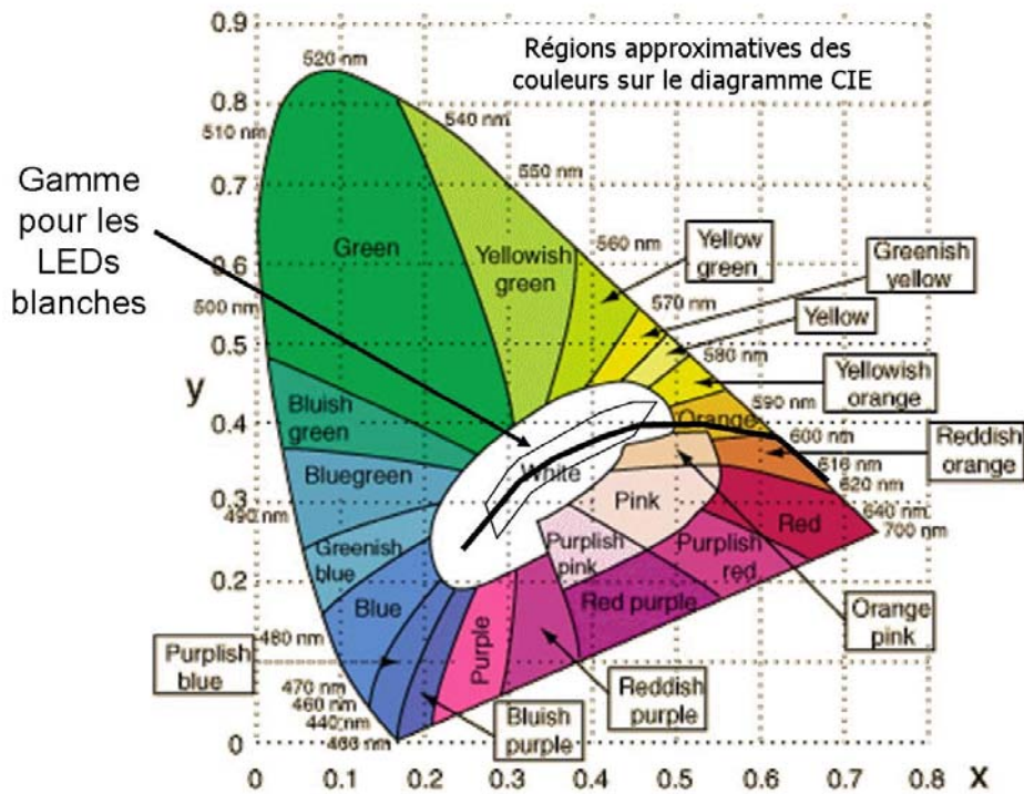
Figure V-6 : Diagramme CIE
