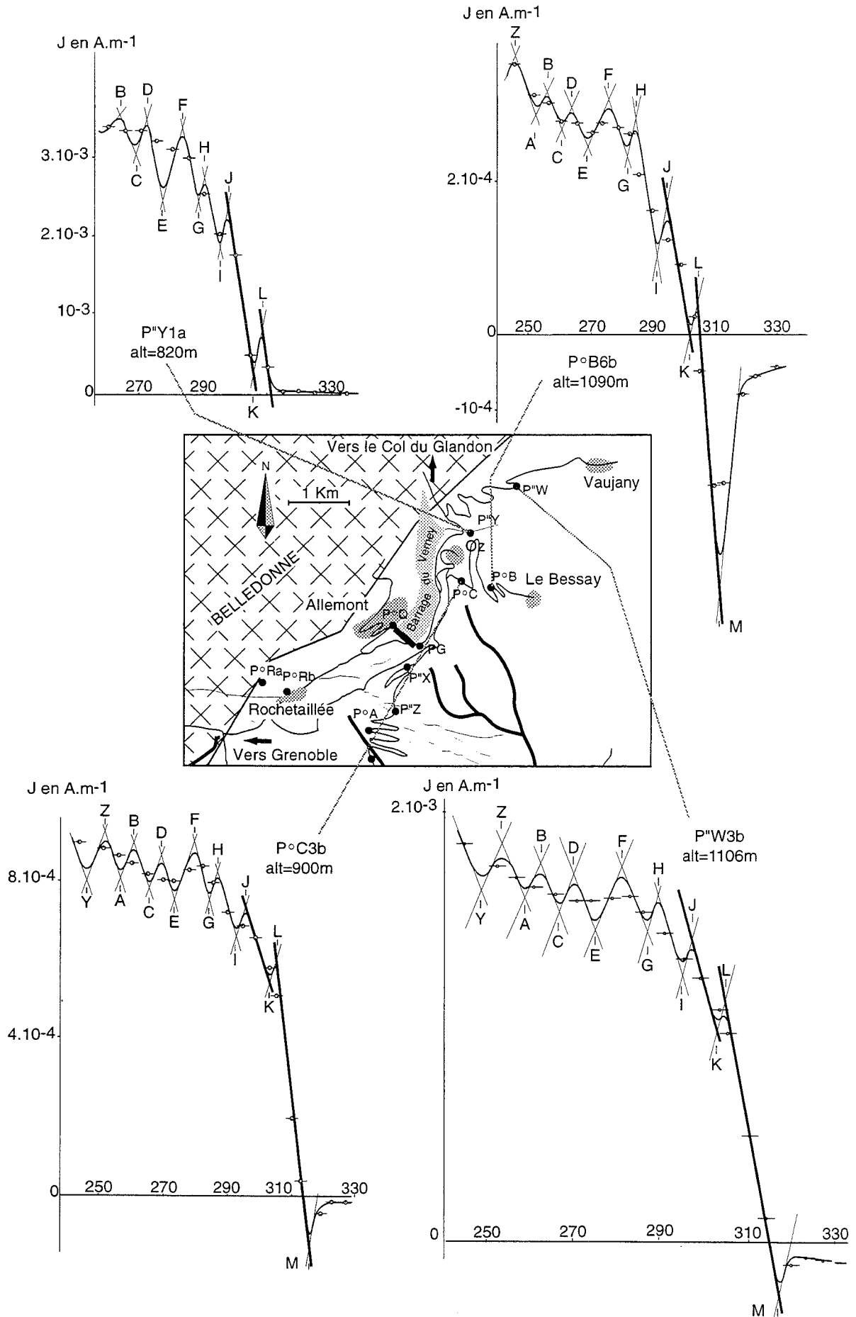
FIG. II.50. - Dessin des courbes de désaimantation thermique interprétées pour les sites du Bessay - Oz et de Vaujany. Le site P o Y, plus bas en altitude s'aimante plus tardivement que les autres. Les pentes calculées sont notées en gras.
