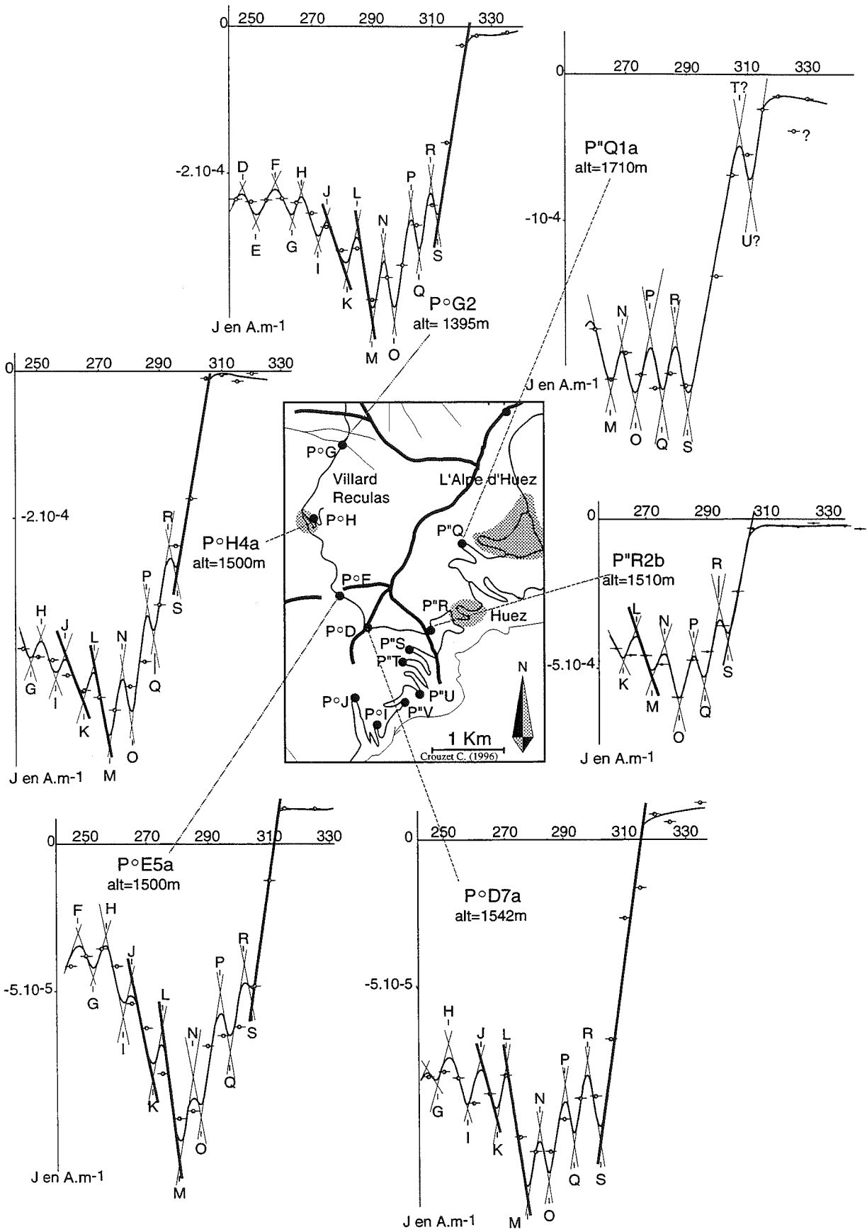
FIG. II.46 (b). – Dessin des courbes de désaimantation thermique interprétées pour les sites du haut du secteur d'Huez. Les pentes calculées sont notées en gras.
