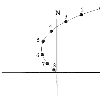
FIG. I.5. - Différents types classiques de diagramme orthogonal.
