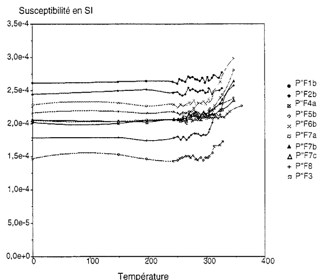
FIG. II.19. – Evolution de la susceptibilité au cours des chauffes pour les 10 spécimens du site P"F. Une légère augmentation débute sur quelques spécimens dès 310^\circ\text{C} .
