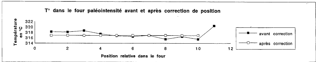
FIG. II.28. - Profil en long des températures de déblocage maximum (Tdm) dans le four à paléointensité avant et après correction de position.
