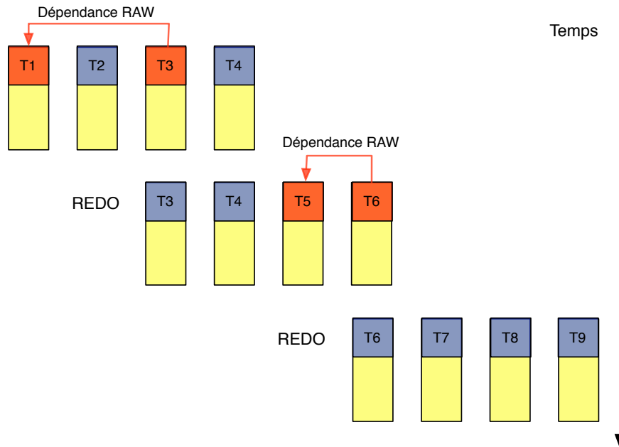
FIG. 1.15 – Schéma d'une politique de roll back and redo sur 4 processeurs.
