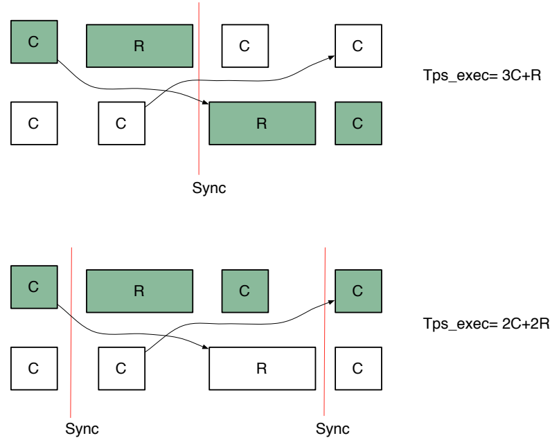
FIG. 1.24 – Deux solutions du placement des barrières de synchronisation pour un même code afin de casser les dépendances de données figurées par les flèches. Le temps d'exécution pour le code à deux barrières est plus court qu'avec une seule. Cet exemple est tiré de la référence bibliographique [19]
