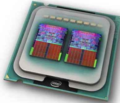
FIG. 1.5 – Le processeur Intel core2 quad core, il est composé de deux "dies" de deux cœurs chacun.
