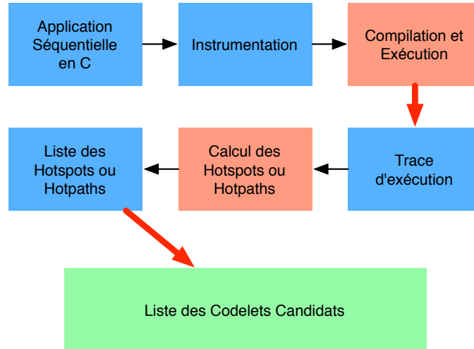
FIG. 1.18 – Schéma du pipeline de calcul des hotspots d'un programme par instrumentation et exécution.
