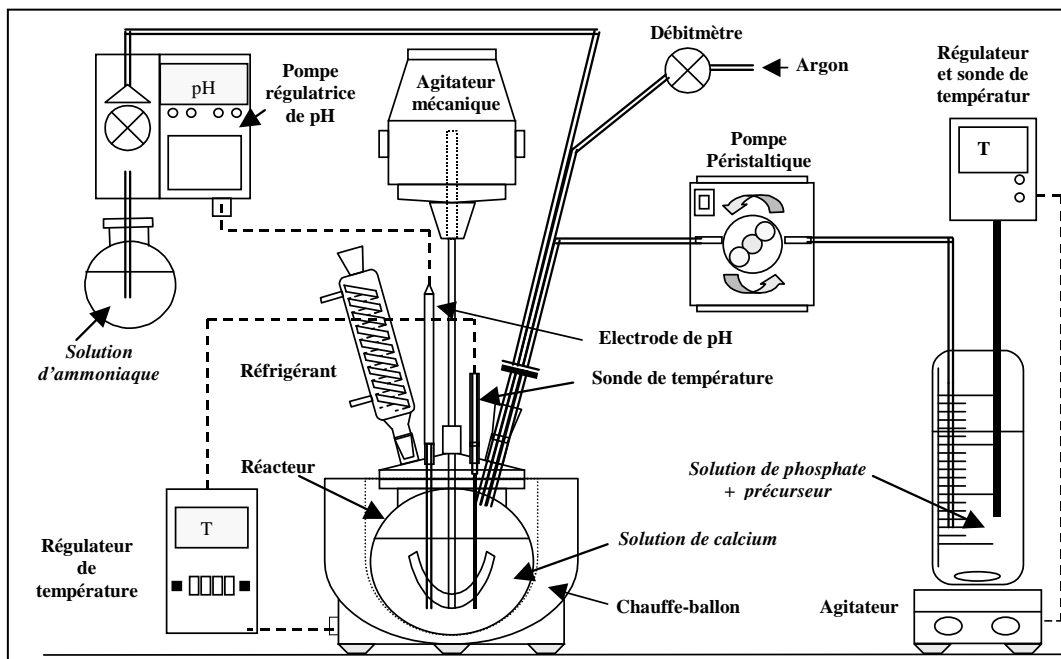
Fig. 2.1 : Schéma du montage de synthèse par précipitation en voie aqueuse
