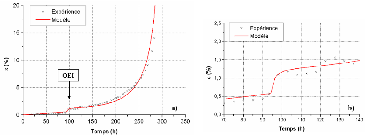
Figure VI-19: Modélisation pour t_{pré} = 100h , t_{OEI} = 150s a) Courbes totales, b) Zoom autour du primaire résiduel
