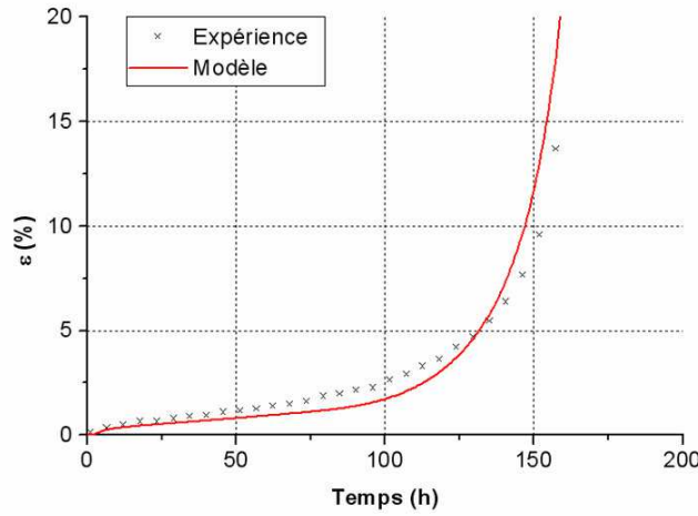
Modélisation d'un OEI initial 30s
