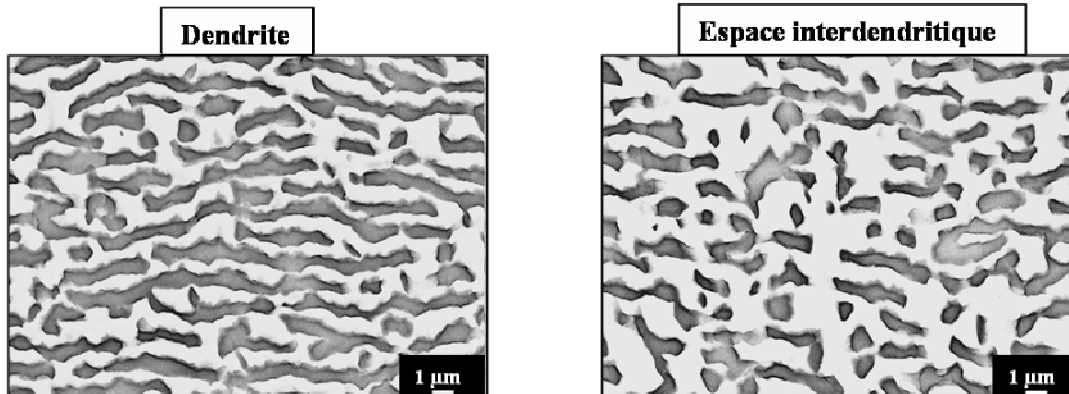
Figure IV-26: Microstructure après 400 heures de fluage ( \gamma' en gris clair)
