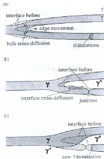
Figure IV-31: Mécanisme de l'inversion topologique entre \gamma et \gamma' [17]
