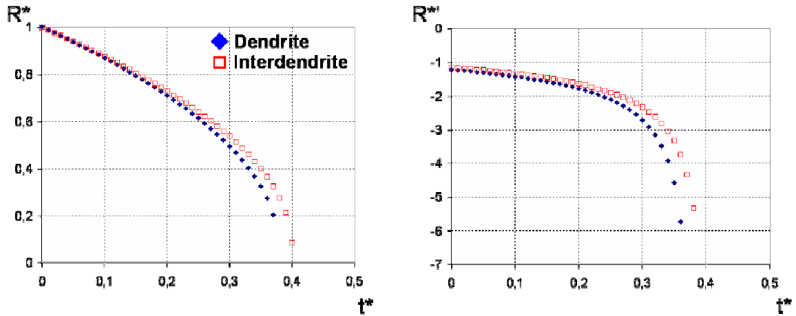
Figure III-11: Simulation de la dissolution de \gamma' : Misfit différent entre les dendrites et les interdendrites
