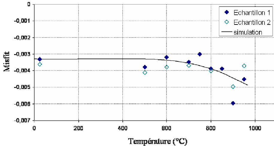
Figure II-5: Evolution du misfit avec la température
