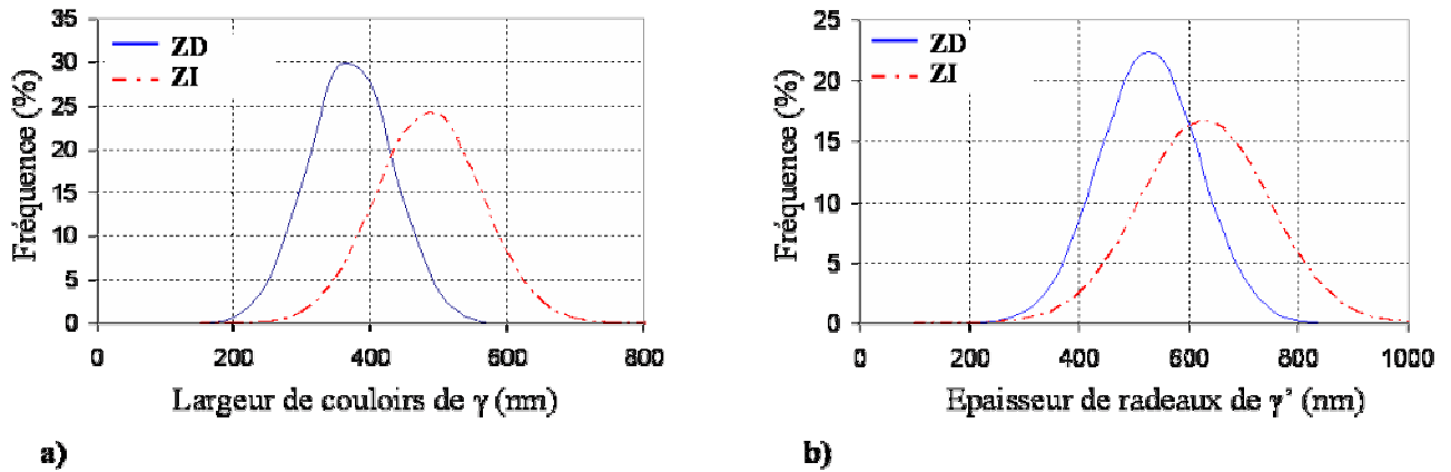
Figure IV-25: Répartition des tailles de \gamma et \gamma' dans la structure dendritique après 200 h de fluage a) Largeur des couloirs de \gamma , b) Epaisseur des radeaux de \gamma'
