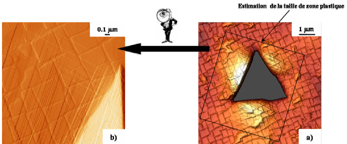
Figure II-19: a) Image AFM d'une indentation, b) Zoom d'un bord de l'indentation
