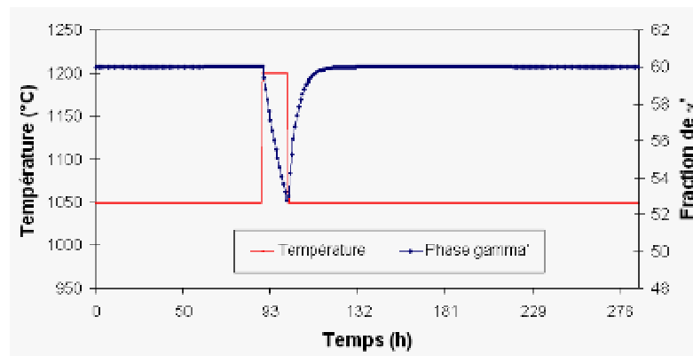
Figure VI-15: Evolution de la fraction de phase \gamma' lors d'un essai anisotherme, t_{\text{pré}} = 100\text{h} et t_{\text{OEI}} = 150\text{s}
