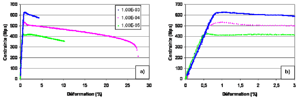
Figure 1: Courbes de traction du MCNG à 1050°C a) Courbes complètes, b) Zoom sur les 3 premiers % de déformation
