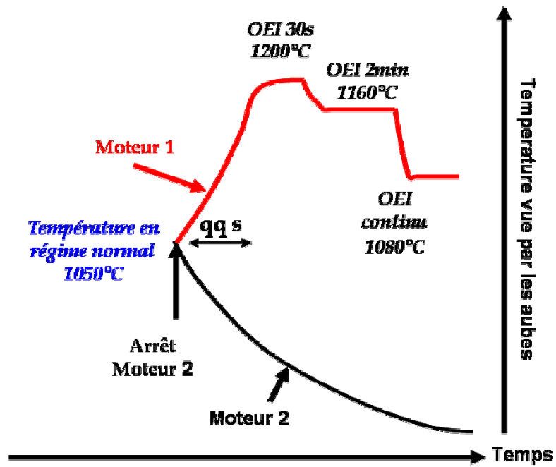
Figure 1: Présentation des régimes d'urgence OEI a) Trajectoire de l'hélicoptère lors d'un régime d'urgence OEI b) Niveaux de température vus par les aubes lors d'un régime d'urgence OEI
