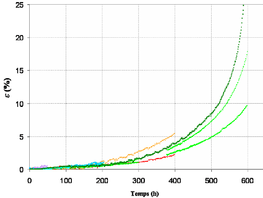
Figure IV-15: Faisceau de courbes de fluage à 1050°C / 140 MPa pour le lot 3 dans le banc FR
