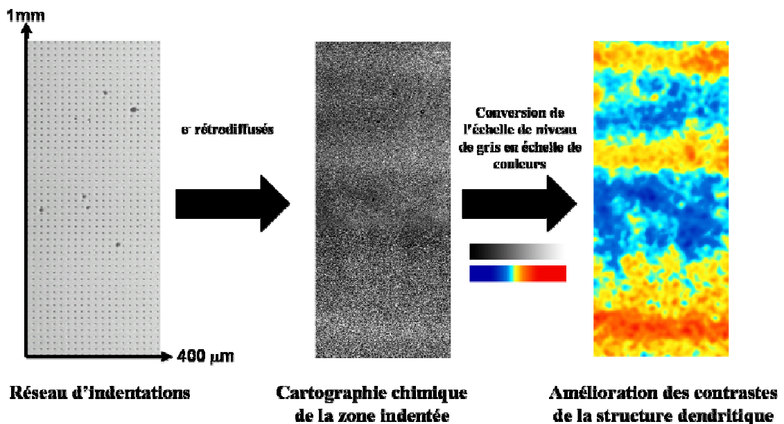
Figure II-17: Cartographie chimique du réseau d'indentations
