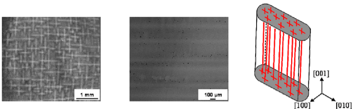
Figure I-3 : Image MEB en mode électrons rétrodiffusés du MCNG a) coupe normale à la direction de croissance \langle 001 \rangle des bras primaires b) coupe longitudinale suivant l'axe de croissance des bras primaires c) Schéma de la structure dendritique dans une éprouvette de fluage paroi mince (Cf. chapitre IV)
