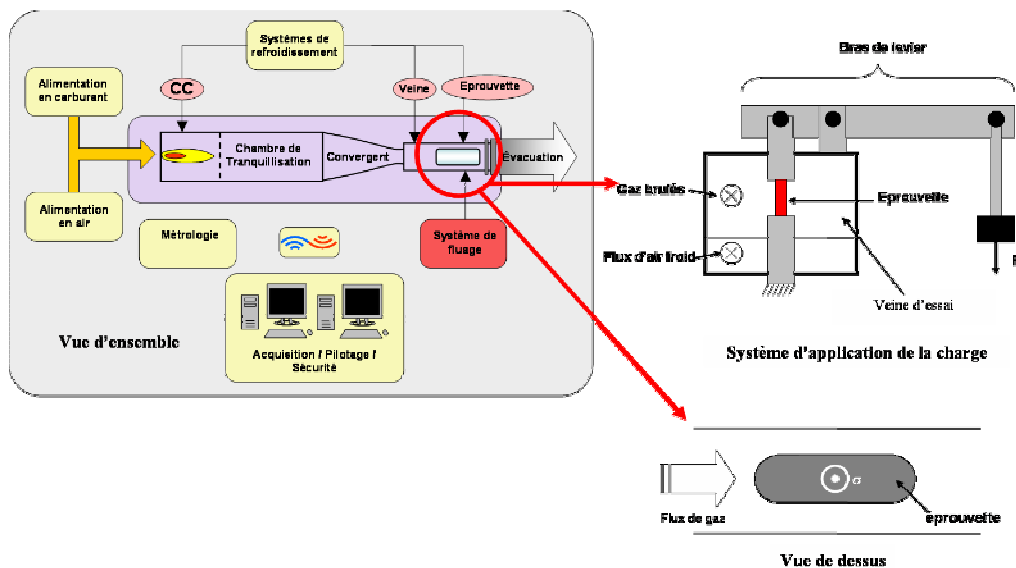
Figure V-2: Schéma de principe du banc THALIE
