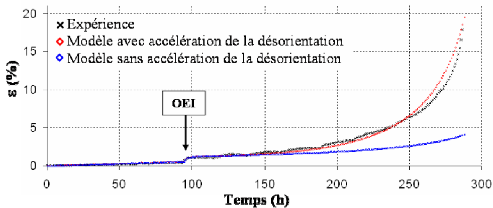
Figure VI-21: Réponse du modèle avec ou sans introduction de l'accélération de la désorientation après l'OEI ( t_{\text{pré}} = 100\text{h} , t_{\text{OEI}} = 150\text{s} )
