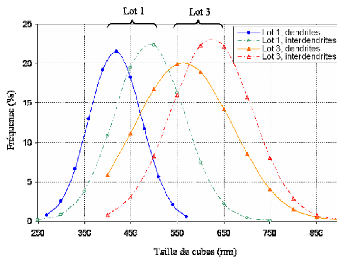
Figure I-8: Tailles des précipités cubiques dans les lots de matière 1 et 3
