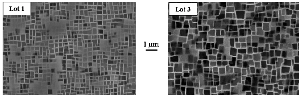
Figure I-7: Microstructure cubique initiale après les traitements thermiques standards dans les lots 1 et 3 (Images dans ZI)
