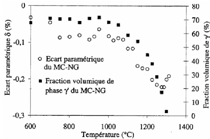
Figure II-1: Corrélation entre l'évolution de la fraction volumique de phase \gamma' et l'écart paramétrique du MCNG [35]
