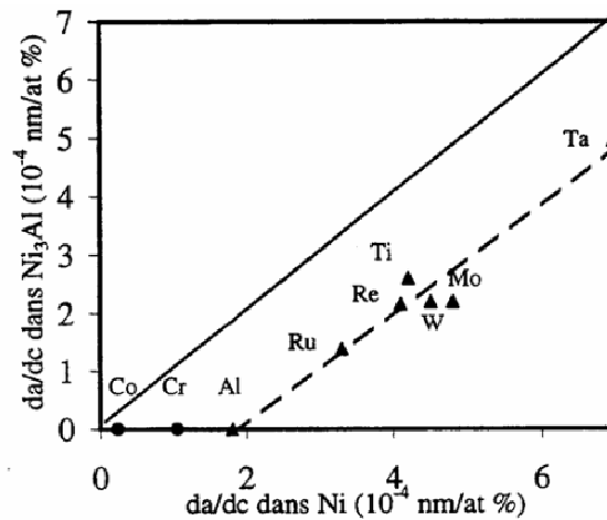
Figure II-2: coefficients de Vegard des éléments des superalliages dans Ni et Ni 3 Al [38-40]
