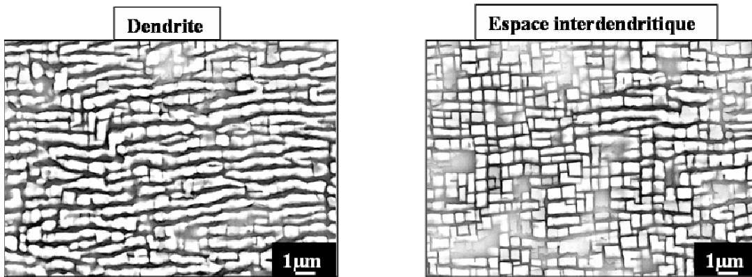
Figure IV-19: Mise en radeaux hétérogène après 50 heures de fluage ( \gamma' en gris clair)
