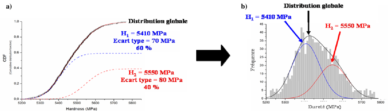
Figure II-14: a) Déconvolution de la densité de probabilité cumulée des mesures d'indentations b) Report des déconvolutions sur l'historgramme des mesures de dureté
