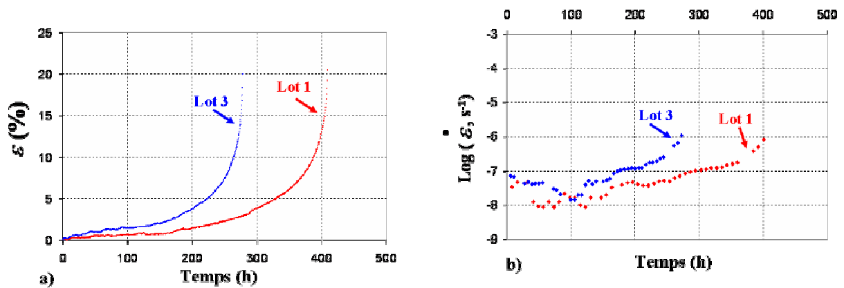
Figure IV-13: Comparaison des courbes de fluage du lot 1 et du lot 3 (banc FL)
