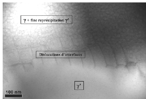
Figure II-7: Réseaux de dislocations à l'interface \gamma/\gamma' sous MET (axe de zone (001), image suivant [100])
