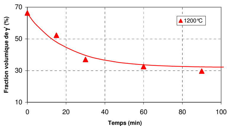
Figure V-14: Courbe de dissolution de la phase \gamma' à 1200°C en l'absence de chargement mécanique
