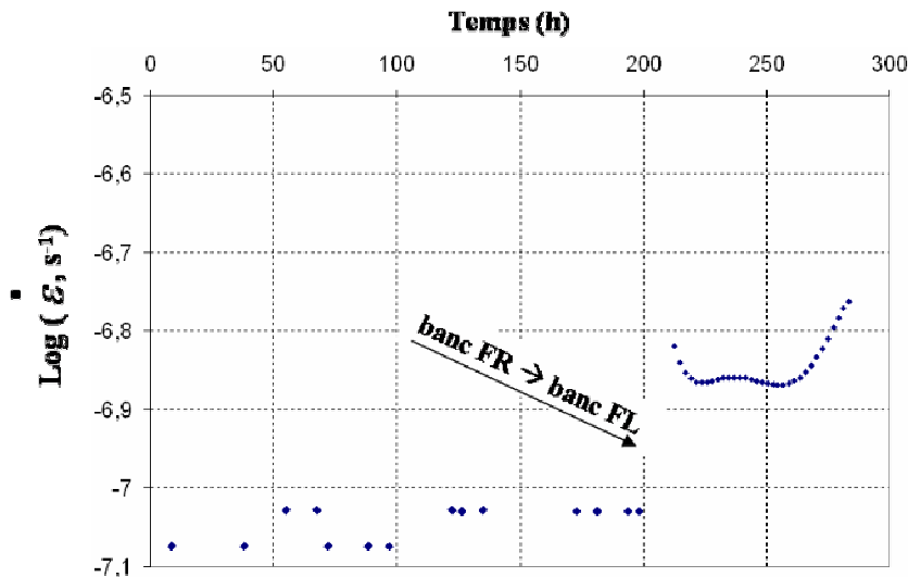
Figure IV-7: Changement de moyen d'essai
