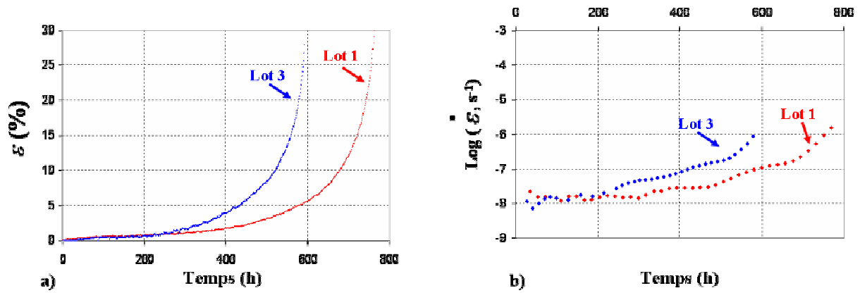
Figure IV-12: Comparaison des courbes de fluage du lot 1 et du lot 3 (banc FR)
