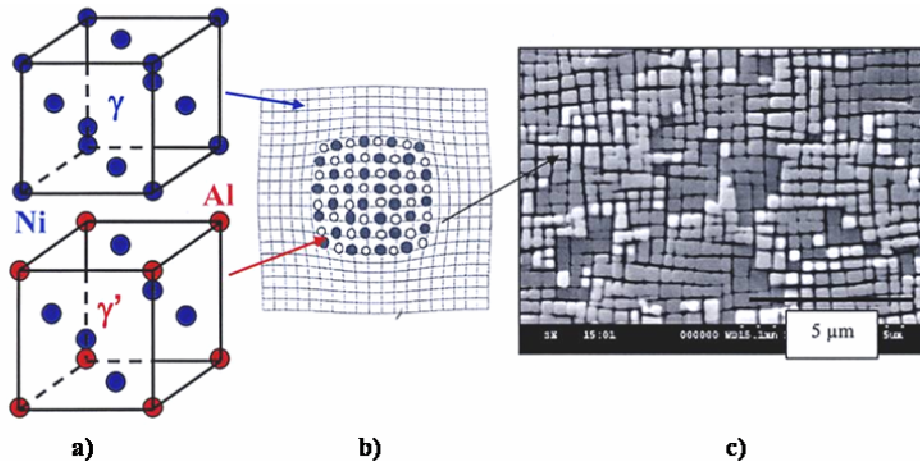
Figure I-1: microstructures d'un superalliage à différentes échelles
