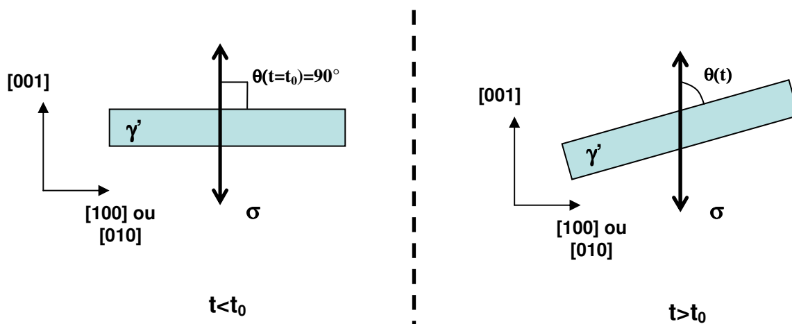
Figure VI-7: Désorientation des radeaux de \gamma'
