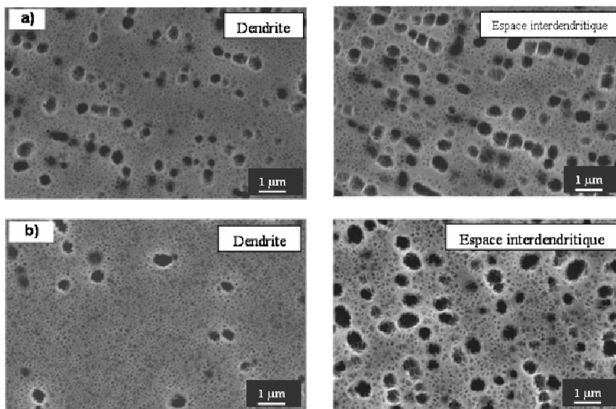
Figure III-9: Microstructures dans les dendrite et les espaces interdendritiques a) après 60 min à 1 250°C, b) 90 min à 1 250°C
