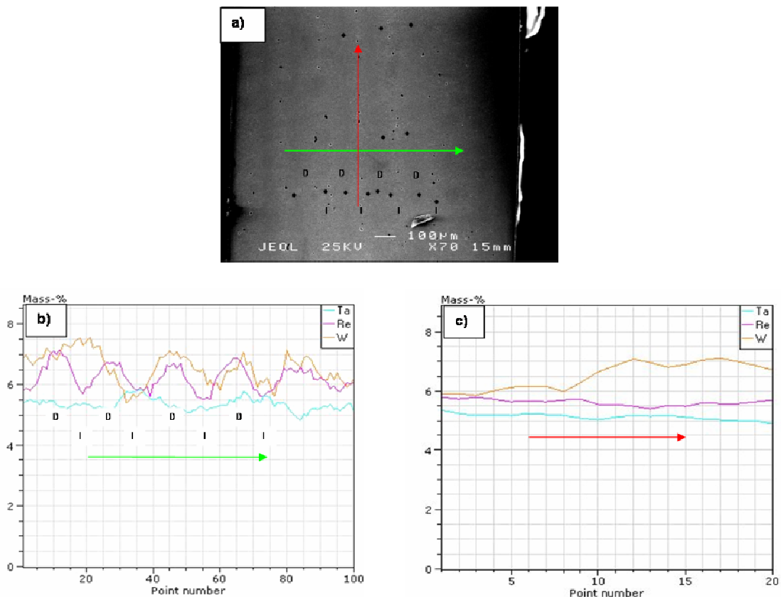
Figure I-5: Analyse EDSX de la structure dendritique a) Section parallèle à l'axe \langle 001 \rangle , repérage préalable des ZD et ZI par microindentation b) Profils de concentration en Re, W et Ta perpendiculairement à l'axe primaire des ZD (% mas.) c) Profils de concentration en Re, W et Ta le long d'une ZI (% mas.)
