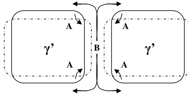
Figure IV-23: Schéma de la mise en radeaux A: flux des \gamma' -formeurs, B: flux de \gamma' -formeurs [10]
