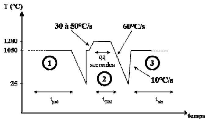
1: Préfluage à 1050°C/140 MPa, banc FR - 2: Surchauffe à 1200°C/145 MPa, banc THALIE - 3: Vie résiduelle à 1050°C/140 MPa, banc FL
