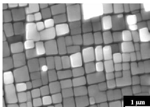
Figure I-9: Microstructure cubique initiale dans MC2 après MS [30]
