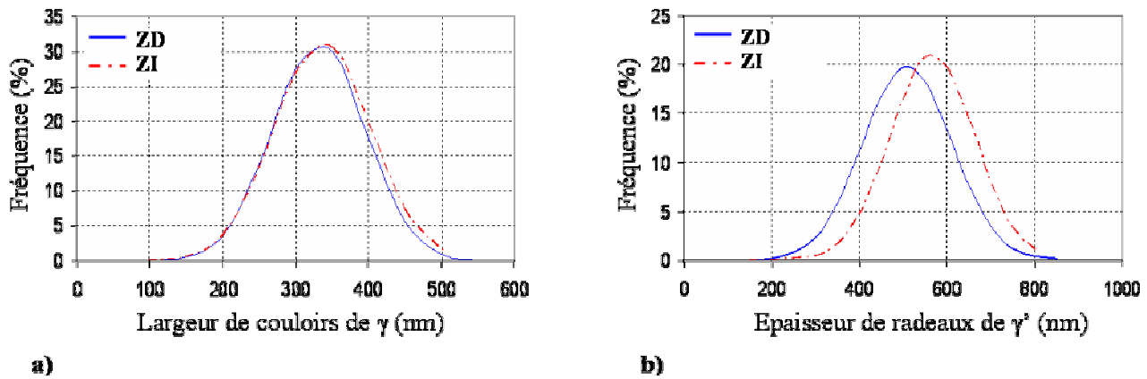
Figure IV-22: Répartition des tailles de \gamma et \gamma' dans la structure dendritique après 100 h de fluage a) Largeur des couloirs de \gamma , b) Epaisseur des radeaux de \gamma'
