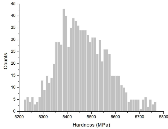
Figure II-13: Histogramme des 1 000 mesures de dureté du réseau d'indentations
