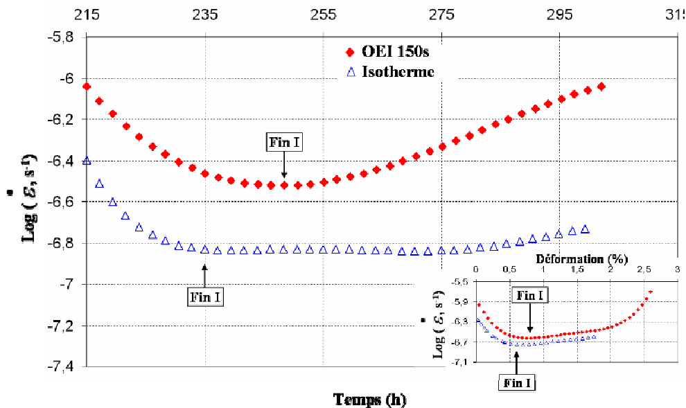
Figure V-9: Comparaison des fluages résiduels des essais {préfluage banc FR ( t_{\text{pré}} = 200\text{h} ) / OEI banc THALIE ( t_{\text{OEI}} = 150\text{s} ) / résiduel banc FL} et {préfluage banc FR ( t_{\text{pré}} = 200\text{h} ) / résiduel banc FL}
