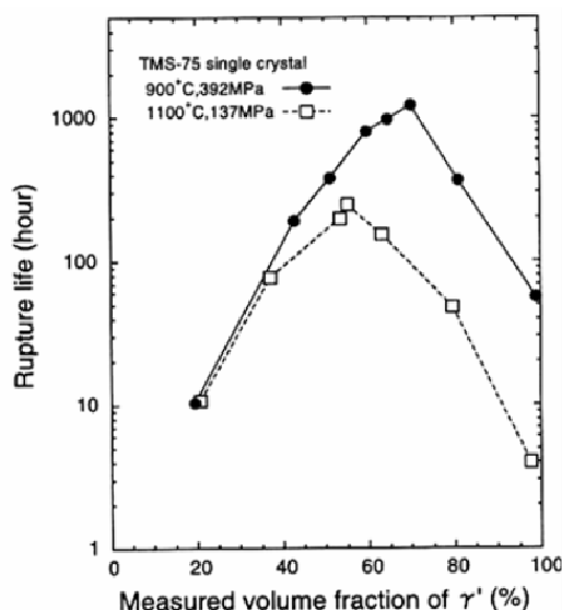
Figure I-2 : Influence du taux de \gamma' sur le temps à rupture pour deux conditions de température/contrainte sur le superalliage monocristallin TMS-75 [5]
