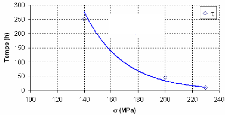
Figure VI-9: Evolution de \tau avec la charge (approximation de la tendance par une loi exponentielle)
