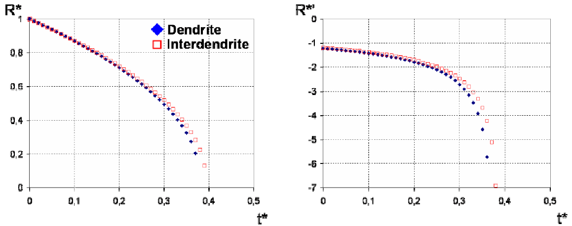
Figure III-14: Simulation de la dissolution de \gamma' : Misfit, coefficient de diffusion et composition chimique différents entre les dendrites et les interdendrites
