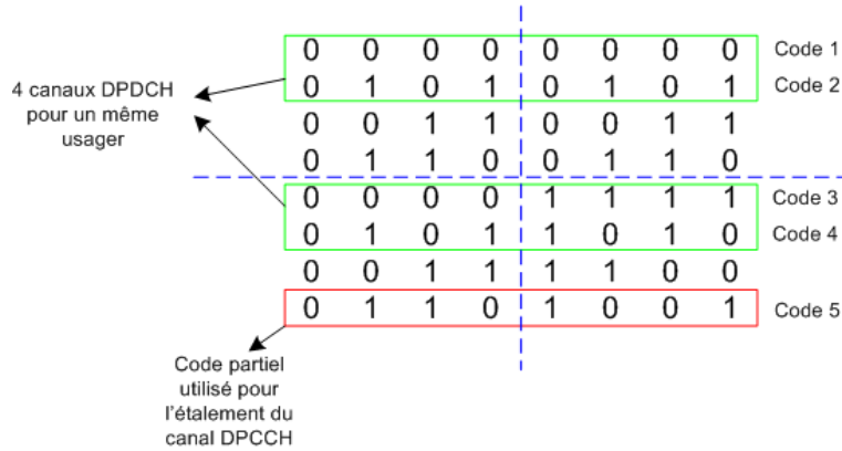
FIGURE 3.42 – Exemple de sélection de 5 codes OVSF (matrice d'Hadamard) : 1 code pour le canal DPCCH et 4 codes pour les 4 canaux DPDCH ( FE = 8 ), alloués à un usager.
