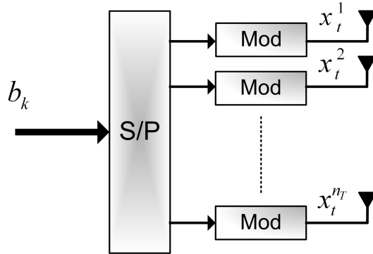
FIGURE 1.6 – Architecture du transmetteur VBLAST.
