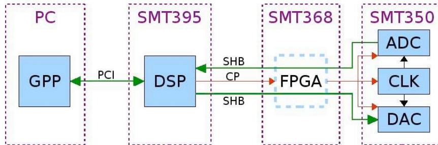
FIG. C.3 – Schéma simplifié de la plat-forme Sundance
