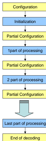
FIG. 3.27 – Séquencement de reconfigurations partielles
