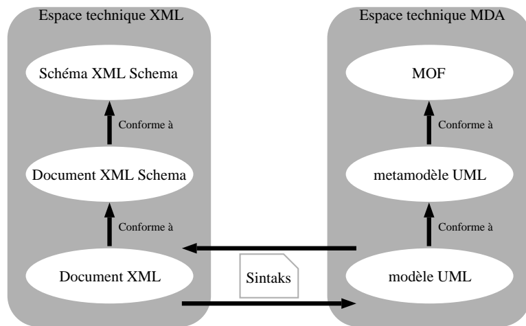
FIG. 3.10: Différences entre l'approche fondée sur le schéma et l'IDM
