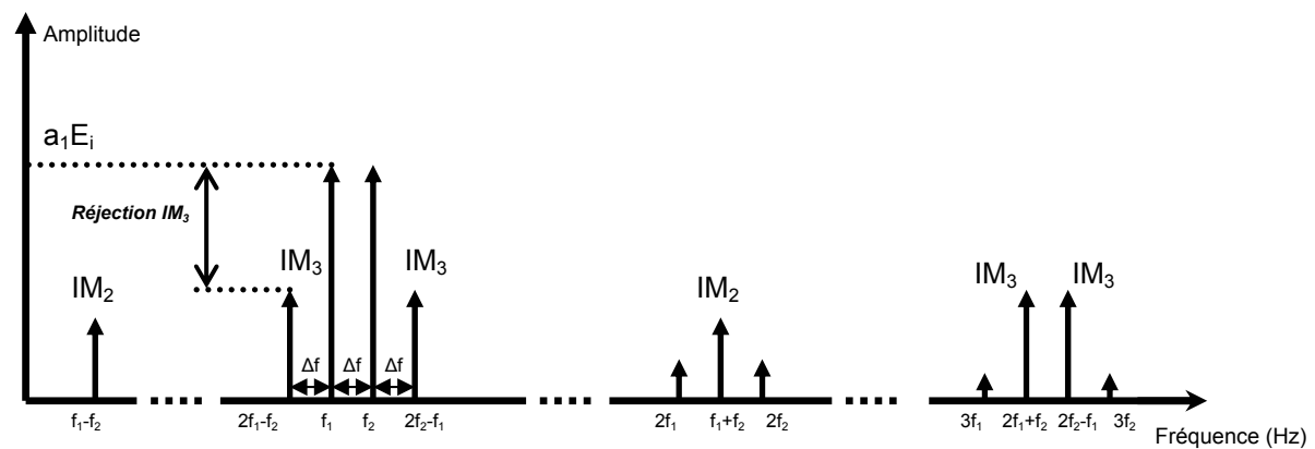
Figure I. 24 : Spectre fréquentiel d'un signal au sortie d'un système non linéaire.
