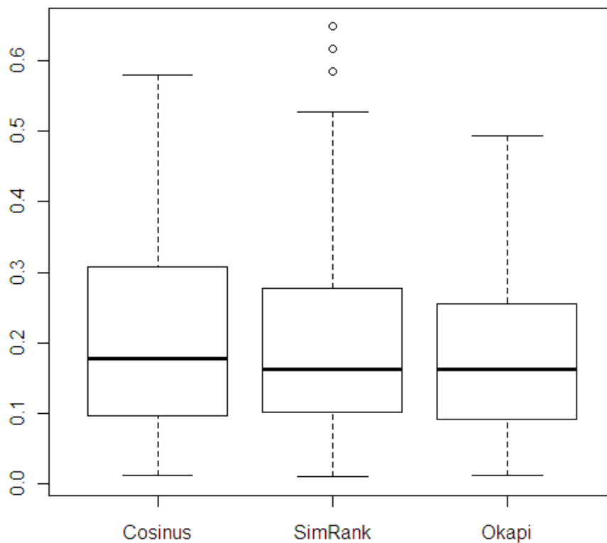
Figure 58 : représentation des MAP pour Cosinus, SimRank et Okapi sur Cisi
