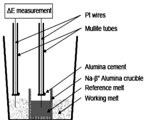
Figure II.9 : Schéma de principe du système expérimental
