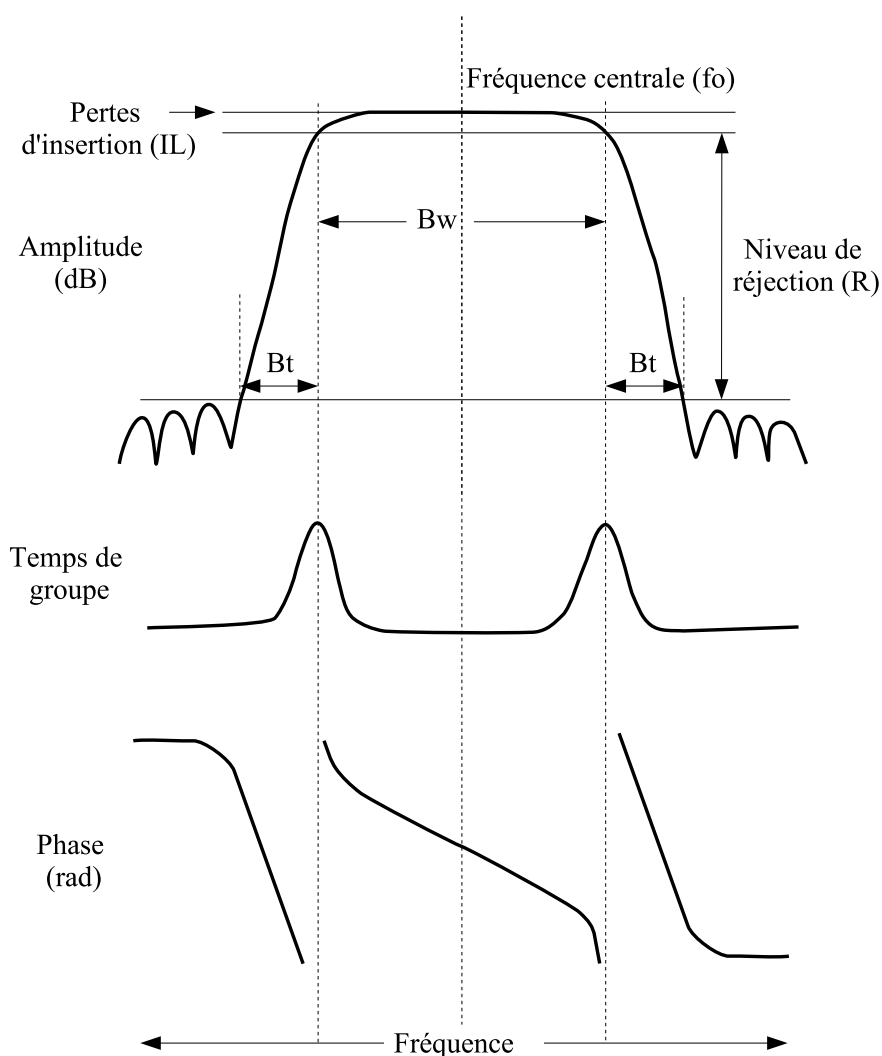
FIG. 1.11 – Caractéristiques électriques types d'un filtre
