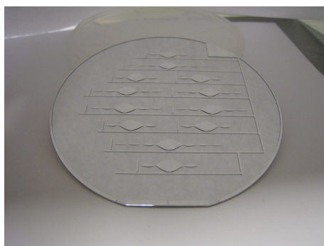
FIG. 6.20 – Photographie des filtres réalisés sur substrat 3 pouces de niobate de lithium
