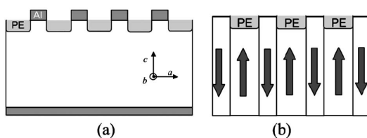
FIG. 4.10 – Principe du masque en échange protonique [75] : (a) Après métallisation et échange protonique – (b) Après gravure du masque métallique et inversion de domaines
