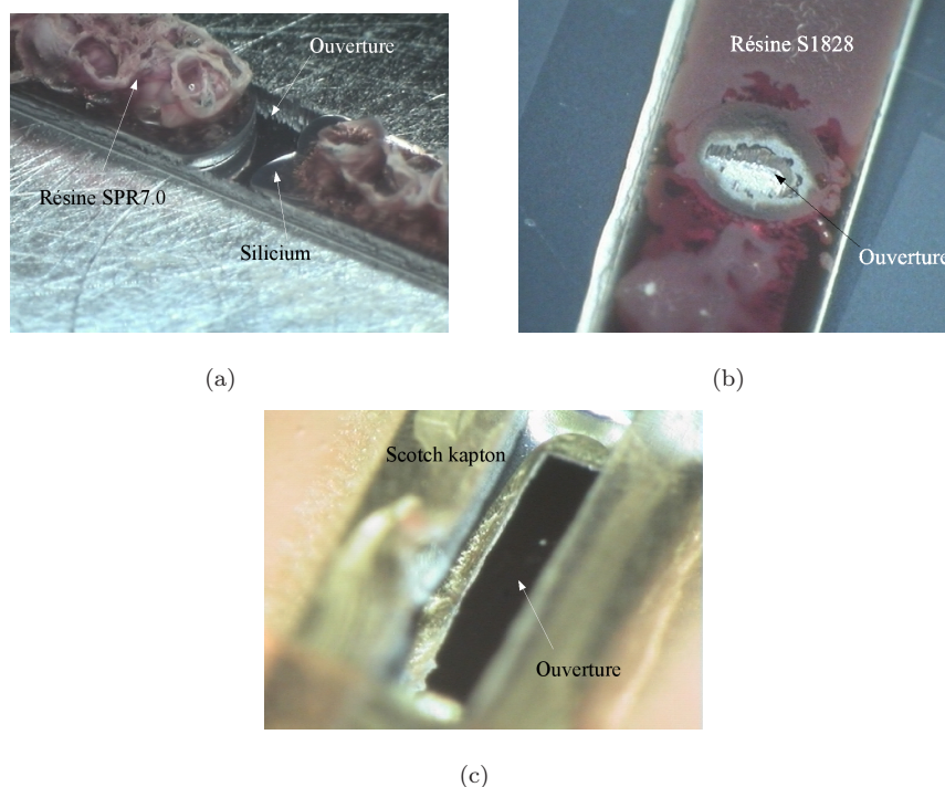
FIG. 4.29 – Photographies de différentes gravures du silicium sur des puces réalisées au microscope 3D (a) Avec un masque en résine épaisse SPR7.0 – (b) Avec un masque en résine fine S1828 – (c) Avec un masque en scotch kapton
