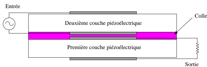
FIG. 1.16 – Principe d'un filtre constitué de deux résonateurs superposés : le Stacked Crystal Filter SCF
