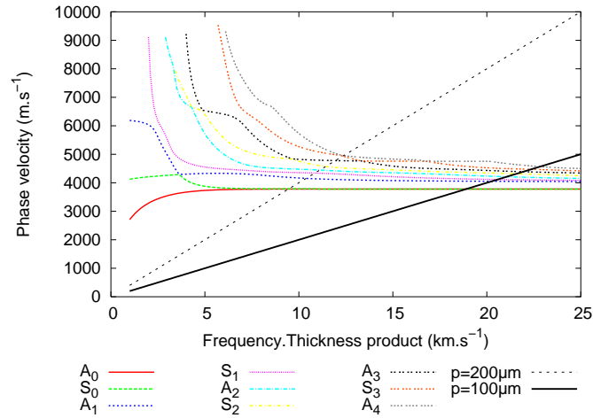
FIG. 5.5 – Courbes de dispersion des modes de Lamb sur du \text{LiNbO}_3 coupe Z. Les droites indiquent les fréquences de fonctionnement attendues pour chaque mode pour une longueur d'onde donnée. [95]
