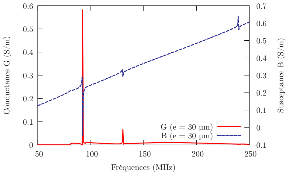
FIG. 5.28 – Réponse d'un transducteur sur niobate de lithium aminci inséré entre deux substrats semi-infinis de niobate de coupe Z ( \lambda = 50 \mu\text{m} , rapport cyclique = 50 %, e_{LiNbO_3} = 30 \mu\text{m} )
