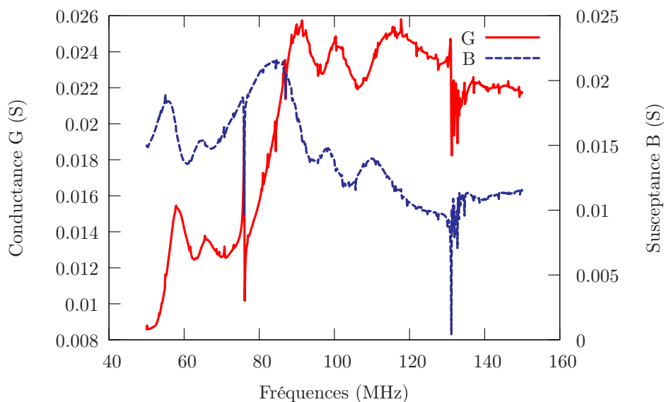
FIG. 6.2 – Réponse d'un transducteur sur niobate de lithium épais ( \lambda = 50 \mu\text{m} , rapport cyclique = 60 %, e_{LiNbO_3} = 500 \mu\text{m} )
