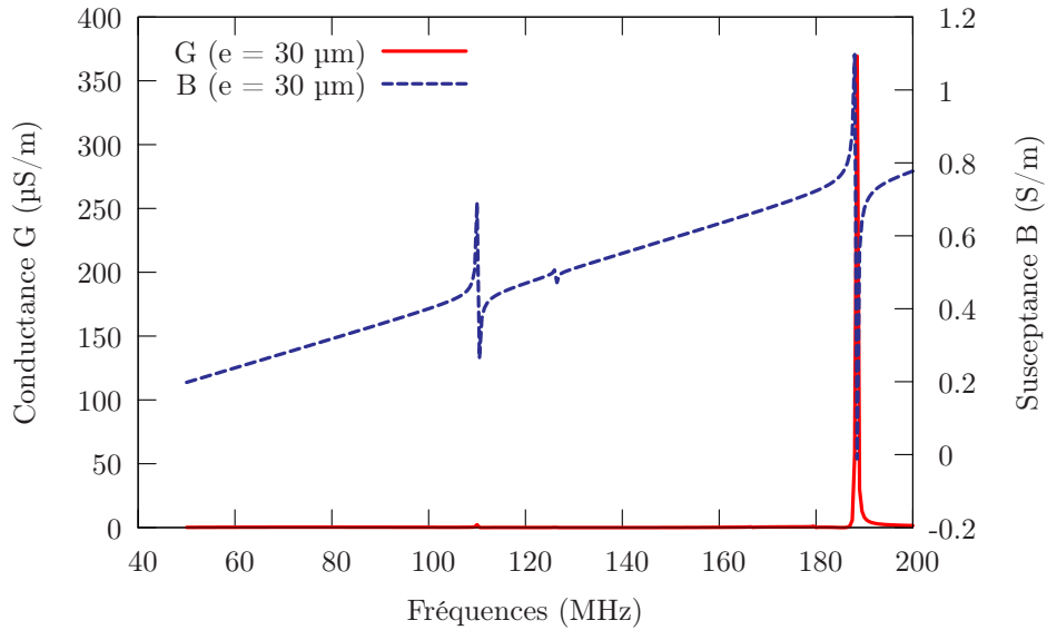
FIG. 5.27 – Réponse d'un transducteur sur tantalate de lithium aminci inséré entre deux substrats semi-infinis de diamant axe C ( \lambda = 50 \mu\text{m} , rapport cyclique = 50 %, e_{LiTaO_3} = 30 \mu\text{m} )
