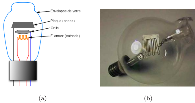
FIG. 1.3 – Schéma (a) et photographie (b) de la triode, ancêtre du transistor (Lee De Forest 1906)
