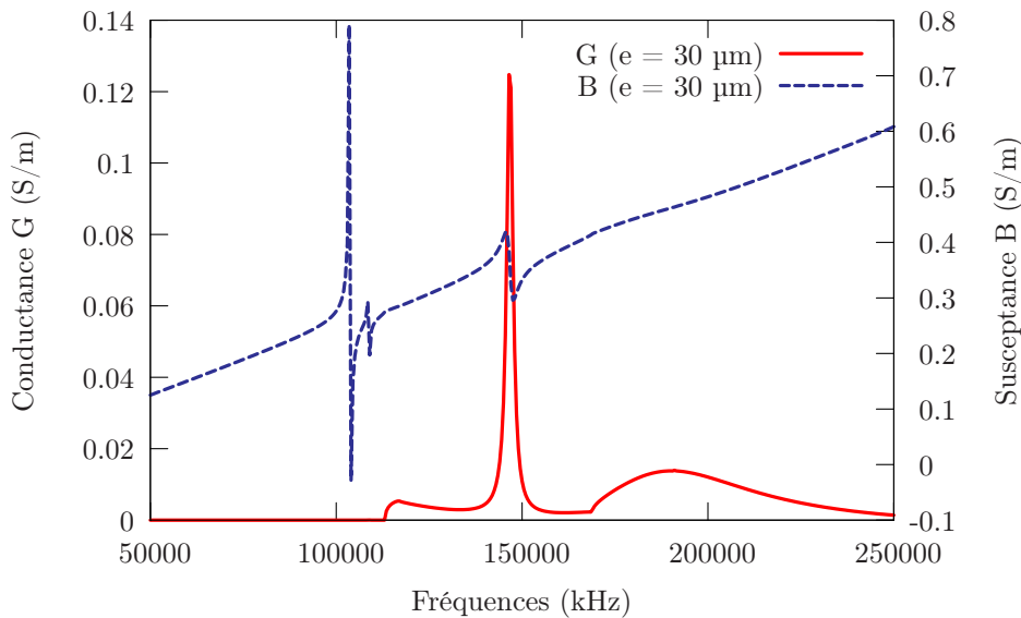
FIG. 5.20 – Réponse d'un transducteur sur niobate de lithium aminci inséré entre deux substrats semi-infinis de silicium ( \lambda = 50 \mu\text{m} , rapport cyclique = 50 %, e_{LiNbO_3} = 30 \mu\text{m} )
