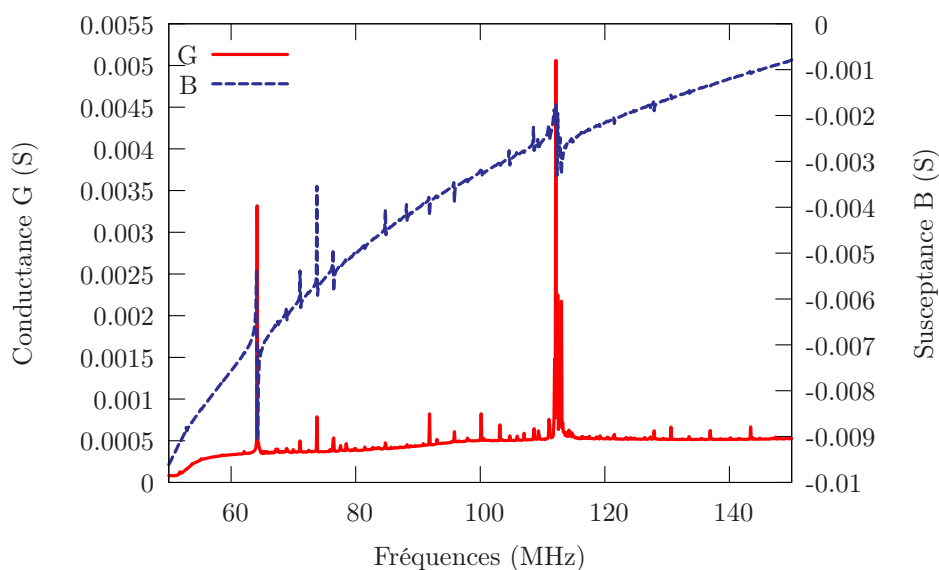
FIG. 6.3 – Réponse d'un transducteur sur tantalate de lithium épais ( \lambda = 50 \mu\text{m} , rapport cyclique = 60 %, e_{LiTaO_3} = 500 \mu\text{m} )
