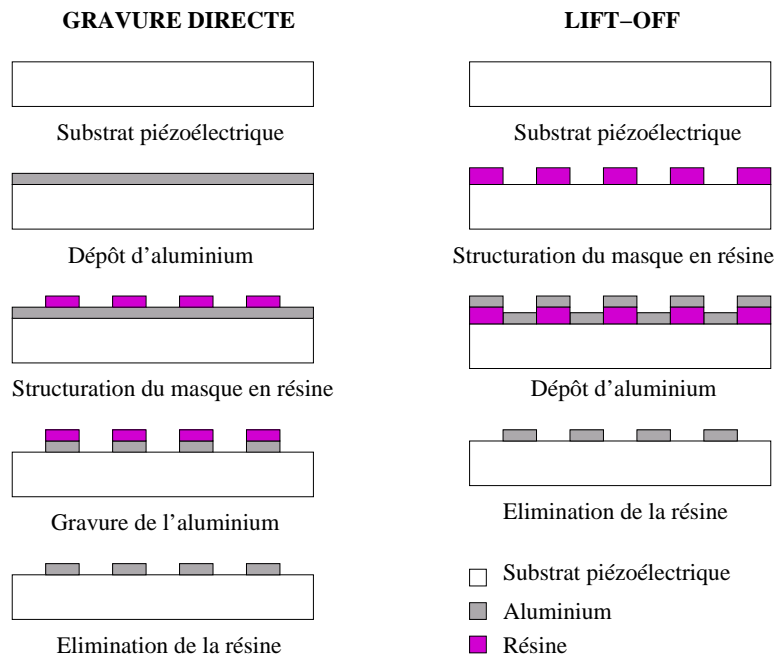
FIG. 2.11 – Schéma de principe des deux méthodes utilisées pour la réalisation de peignes interdigués
