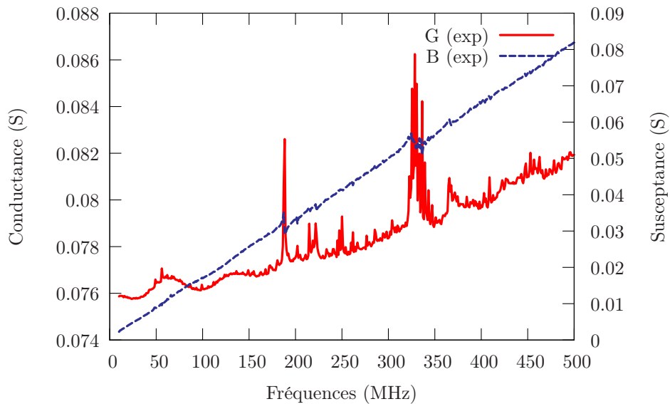
FIG. 6.9 – Admittance expérimentale d'un transducteur sur niobate de lithium aminci ( \lambda = 20\ \mu\text{m} , rapport cyclique = 60 %, e_{LiNbO_3} = 50\ \mu\text{m} )
