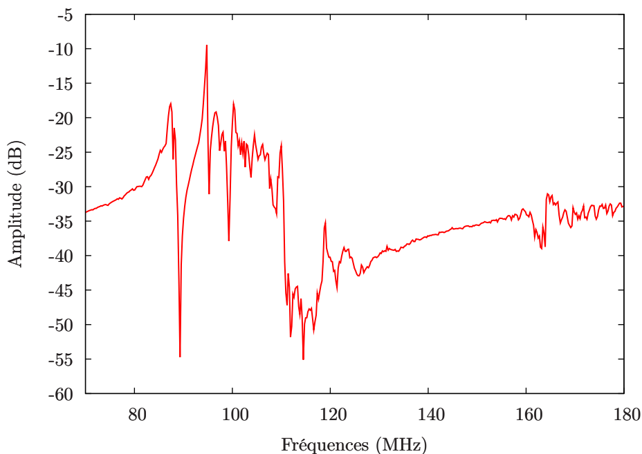
FIG. 6.14 – Fonction de transfert obtenue avec un filtre à base de rectangles (de largeurs respectives 10 et 20 \lambda ) séparés par 15 \lambda ( \lambda = 40 \mu\text{m} , e_{\text{LiNbO}_3} = 500 \mu\text{m} )
