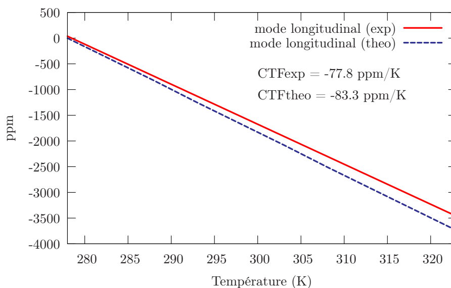
FIG. 6.29 – Comparaison des dérives en température expérimentale et théorique du véhicule de test \text{Si}(380\ \mu\text{m})/\text{Niobate}(500\ \mu\text{m})/\text{Si}(380\ \mu\text{m})
