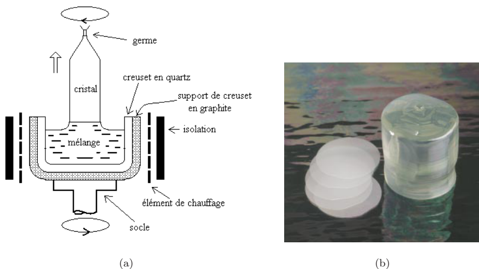
FIG. 2.5 – (a) Schéma de principe du procédé de croissance d'un cristal de Czochralski et (b) « carotte » de niobate de lithium (CrystalTechnologies) obtenue par cette technique [55]
