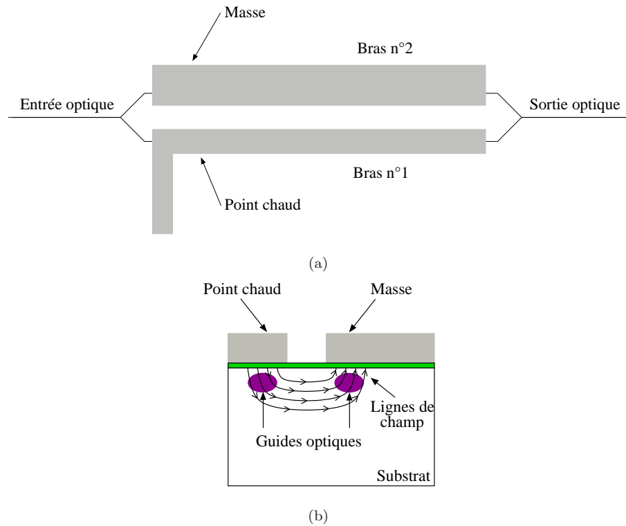
FIG. 3.12 – Représentation d'un modulateur Mach-Zehnder : (a) vue de dessus et (b) vue en coupe : la zone colorée entre les électrodes et le substrat est une couche tampon pour éviter les pertes optiques dans le métal
