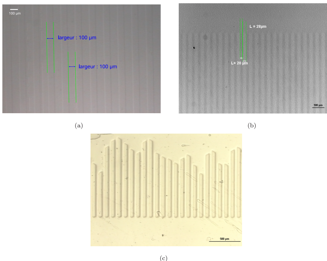
FIG. 4.5 – Inversion de domaines vues au microscope optique (a) Inversion totale sur LiNbO 3 (rapport cyclique de 50 %) – (b) Inversion totale sur LiTaO 3 (rapport cyclique de 35 %) – (c) Inversion incomplète sur LiNbO 3
