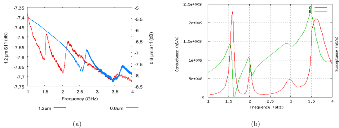
FIG. 2.15 – (a) Paramètre S_{11} mesurés expérimentalement sur deux PIT de différentes longueurs d'onde; (b) Admittance harmonique théorique calculée pour un PIT de 1,2\ \mu\text{m} de longueur d'onde
