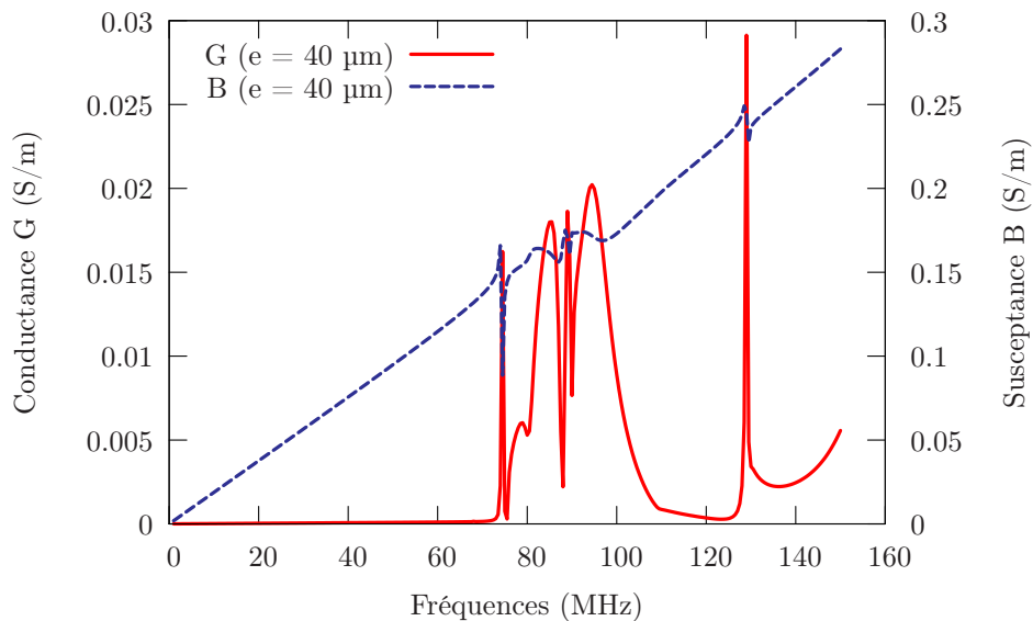
FIG. 5.19 – Réponse d'un transducteur sur niobate de lithium aminci reporté sur un substrat semi-infini de quartz coupe (YXl)/60 ( \lambda = 50 \mu\text{m} , rapport cyclique = 50 %, e_{LiNbO_3} = 40 \mu\text{m} )
