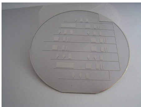
FIG. 6.13 – Photographie des dispositifs de validation réalisés sur substrat 3 pouces de niobate de lithium
