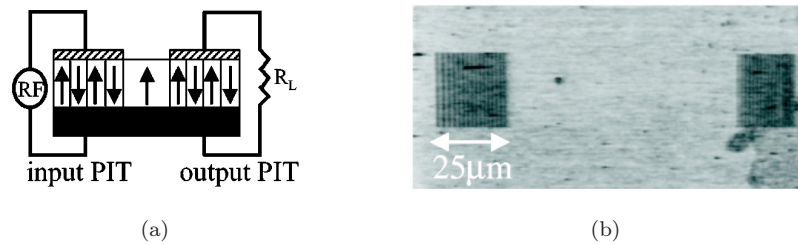
FIG. 2.14 – Schéma de principe du dispositif SAW (a) : image d'un des premiers prototypes SAW réalisé (b) : la distance entre les deux transducteurs est d'environ 70\ \mu\text{m} et la distance entre deux domaines de polarisations différentes est de 0,6\ \mu\text{m} , ce qui correspond à une longueur d'onde acoustique de 1,2\ \mu\text{m} [63]
