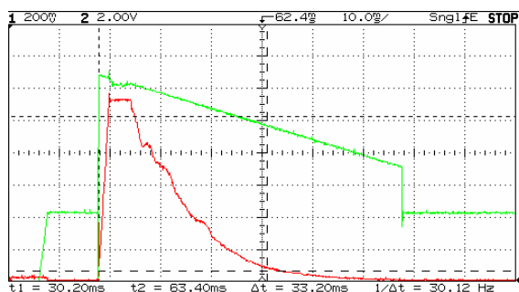
FIG. 4.12 – Courbes tension/courant délivrés lors de l'inversion de domaines avec un masque en échange protonique
