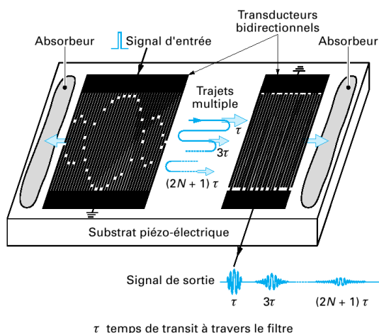
FIG. 3.6 – Structure classique d'un filtre à deux transducteurs bidirectionnels [69]
