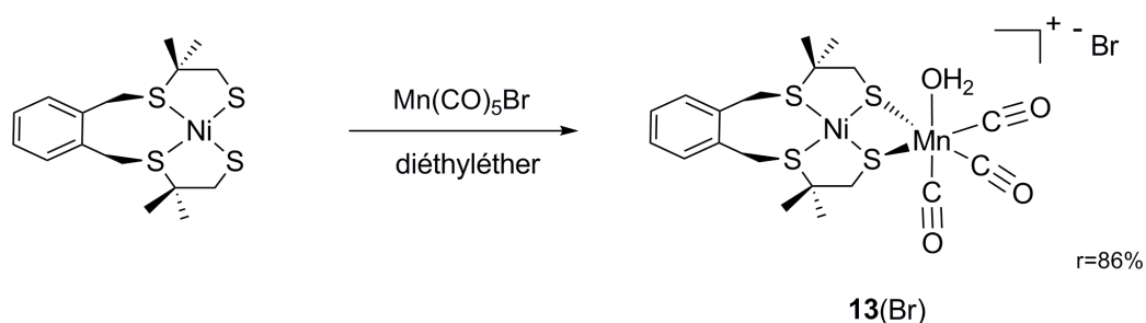
Figure 105 : synthèse du complexe dinucléaire Ni-Mn \mathbf{13}(\text{Br})
