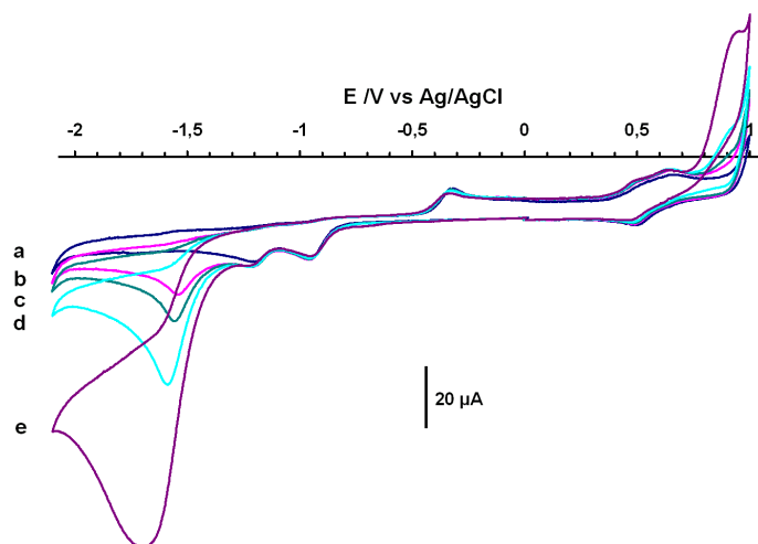
Figure 83 : voltammogrammes cycliques de 9(Cl) ( 1,0 \text{ mmol.L}^{-1} ) en présence de plusieurs équivalents de l'acide \text{Et}_3\text{NHCl} ( a ) 0 éq ; b) 1 éq ; c) 1,5 éq ; d) 3 éq ; e) 10 éq) enregistrés dans une solution de n\text{-Bu}_4\text{NBF}_4 dans le DMF ( 0,1 \text{ mmol.L}^{-1} ) sur une électrode de carbone vitreux à 100 \text{ mV.s}^{-1}
