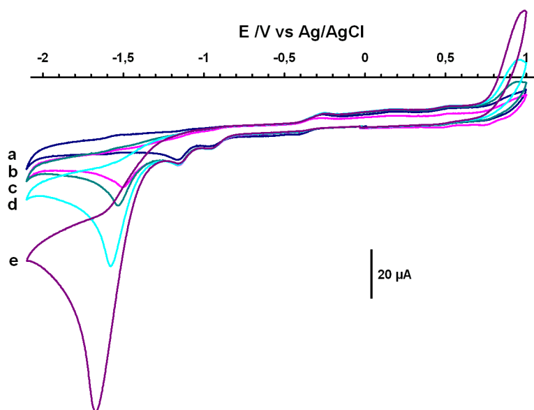
Figure 84 : voltammogrammes cycliques de 10(\text{NO}_3)_2 ( 1,0 \text{ mmol.L}^{-1} ) en présence de plusieurs équivalents de l'acide \text{Et}_3\text{NHBF}_4 ( a ) 0 éq ; b) 1 éq ; c) 1,5 éq ; d) 3 éq ; e) 10 éq) enregistrés dans une solution de n\text{-Bu}_4\text{NBF}_4 dans le DMF ( 0,1 \text{ mmol.L}^{-1} ) sur une électrode de carbone vitreux à 100 \text{ mV.s}^{-1}
