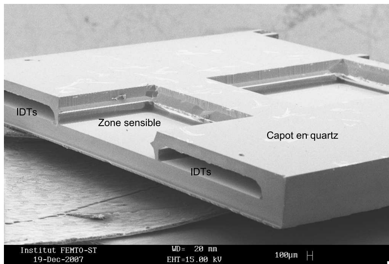
FIG. 4.34 – Capteur équipé de son capot en quartz
