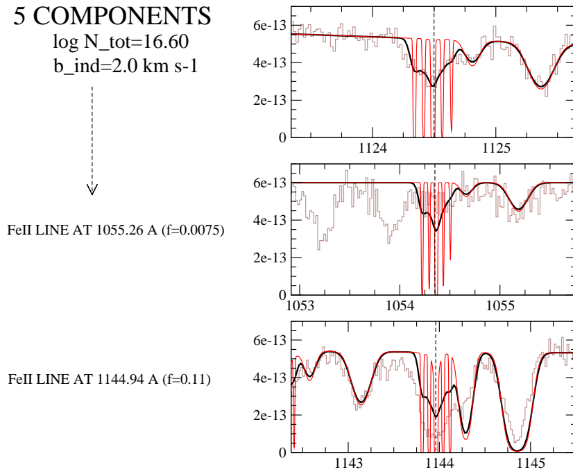
FIG. 5.5 – On utilise une distribution arbitraire de 5 composantes ayant des largeurs Doppler de 2 \text{ km s}^{-1} pour reproduire le profil de la raie de profondeur intermédiaire à 1125 \text{ \AA} . La densité de colonne obtenue n'est pas cohérente avec les profils de la raie faible à 1055 \text{ \AA} et de la raie saturée à 1145 \text{ \AA} . Cette distribution ne parvient pas à reproduire toutes les raies de Fe II.
