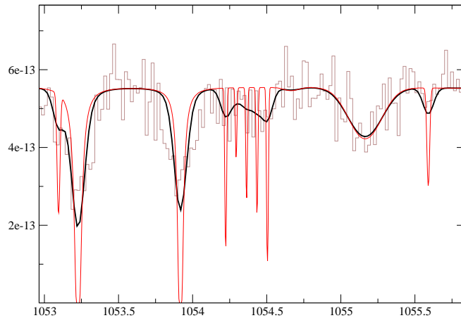
FIG. 5.4 – La faible raie de Fe II à 1055.26 \text{ \AA} ne peut pas être constituée de composantes saturées si ces composantes ont des largeurs Doppler \geq 2 \text{ km s}^{-1} .
