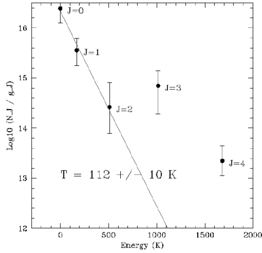
FIG. D.1 – Diagramme d’excitation du \text{H}_2 diffus dans NGC604. Les densités de colonne des niveaux rotationnels divisés par les poids statistiques sont tracés en fonction de l’énergie d’excitation. Le rapport des niveaux J = 0 et 1 donnent une température rotationnelle de T_{01} = 112 \pm 10 K.
