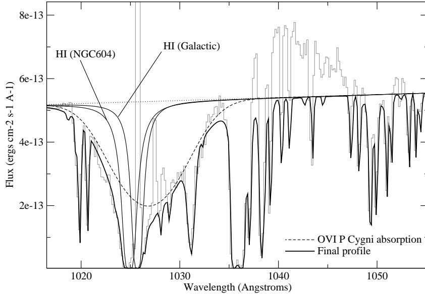
FIG. 4.7 – Le profil \text{Ly}\beta observé dans le spectre LWRFS FUSE est contaminé par l'absorption du doublet stellaire P Cygni O VI. La composante en émission n'a pas été prise en compte pour le calcul des ajustements de profils. Pour des raisons d'affichage, toutes les autres raies interstellaires ne sont pas identifiées et les données ont été rééchantillonnées par un facteur 8.
