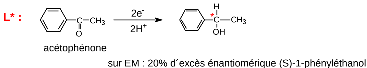
Schéma 4: Hydrogénation de l'acétophénone par le complexe [Rh(Cl)_2(L^*)_2]^+
