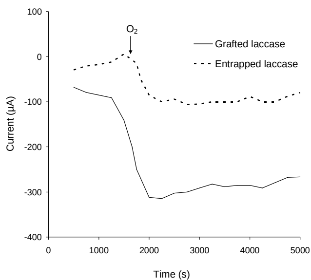
Figure 3 : Electrolyse de l'oxygène dissous en eau à +0.4V vs Ag/AgCl dans la solution tampon citrate/phosphate pH 3 en présence d'ABTS à la biocathode laccase piégée (—) et biocathode laccase greffée (---).
