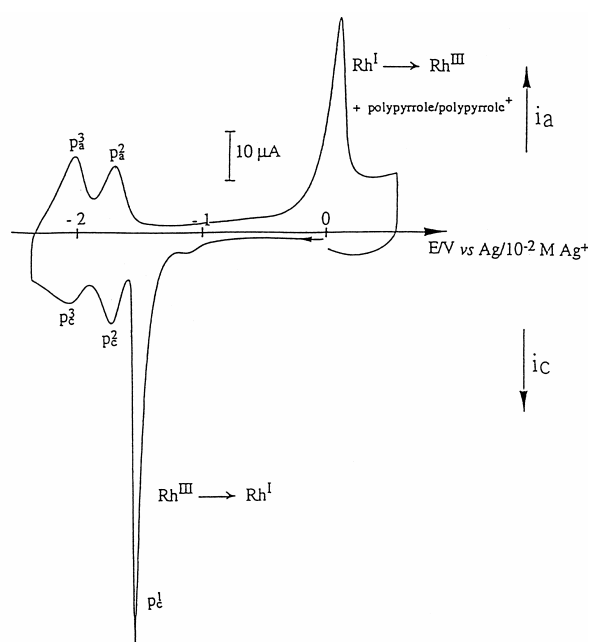
Figure 1 : Courbe de voltammétrie cyclique du matériaux C/[Rh(Cl)_2(L_1)_2]^+ dans l'acétonitrile, 0.1M perchlorate de tétra- n -butylammonium, vitesse de balayage = 100 \text{ mV.s}^{-1} .
