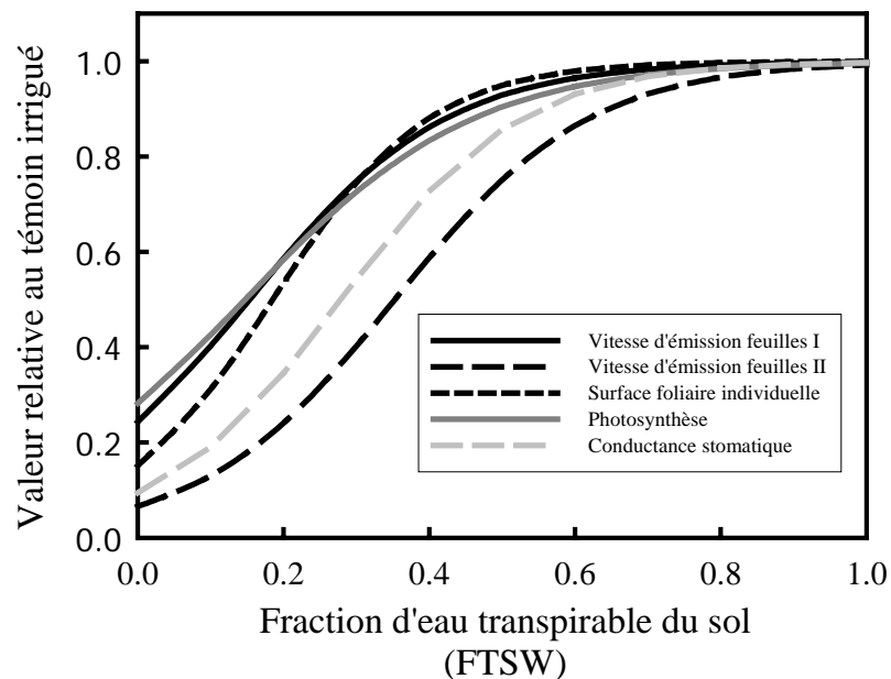
Figure I.15 : Courbes de réponse des différents processus au déficit hydrique (d'après Lebon et al. , 2006)
