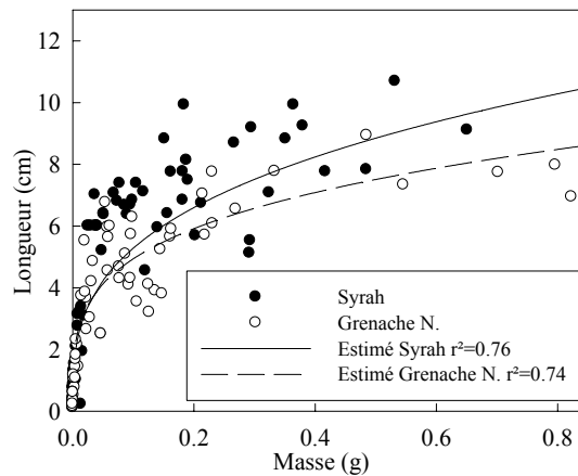
Figure II.10 : Relations allométriques obtenues entre les longueurs des entrenœuds et leur masse associée au cours de leur expansion
