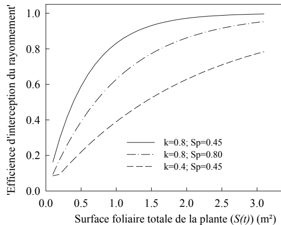
Figure II.11 : Évolution de l'efficacité d'interception du rayonnement [(1-\exp(-k.(S(t)/S_p)))] en fonction de la surface foliaire totale S(t)
