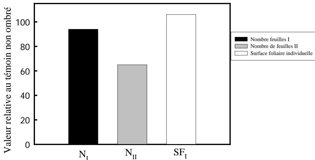
Figure I.16 : Influence de la compétition trophique sur les différents processus de développement
