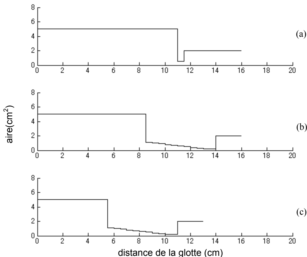
Figure 78. Fonctions d'aire de /ʃ/. La glotte est représentée à gauche et les lèvres à droite. (a) Configuration avec constriction courte. (b) /ʃ/ avec constriction longue (palatalisé). (c) /ç/ avec constriction longue, et conduit vocal court.
