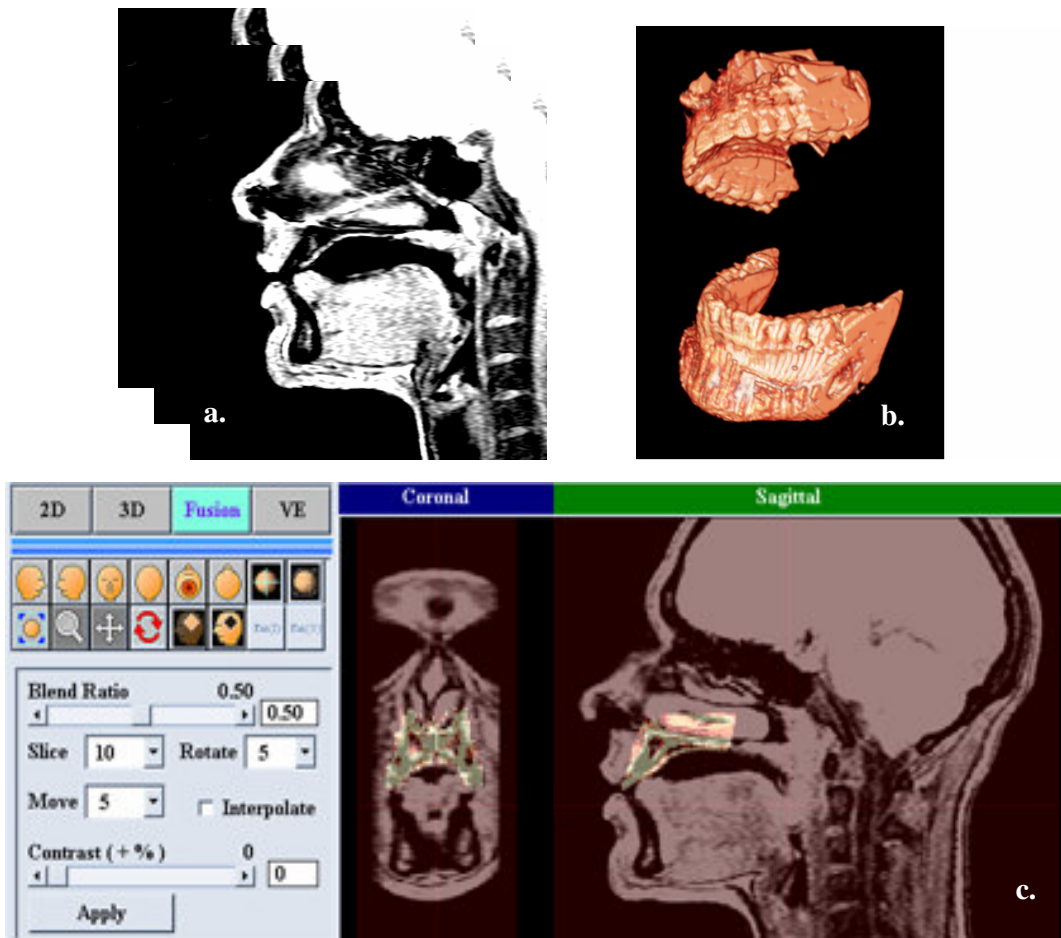
Figure 5. Insertion des moulages numériques des dents supérieures et inférieures. (a) Données 3D des fricatives ; (b) moulages numériques 3D des dents ; (c) copie d'écran illustrant l'insertion des dents par rotation et translation dans un logiciel de traitement de données volumétriques, Intage-rv.
