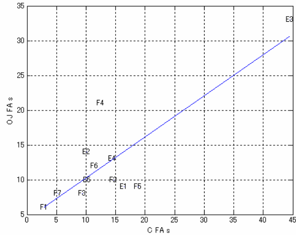
Figure 176. Overjet en fonction de l'aire de la constriction, /s/, français et anglais.
