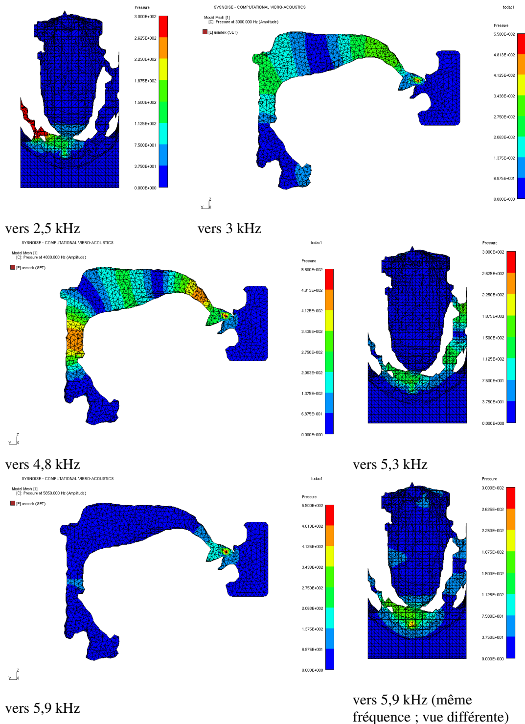
Figure 88. Distribution de pression à la fréquence des pics spectraux, à l'intérieur du conduit vocal 3D /s j / jp de FrJ. Vues de l'intérieur du conduit vocal 3D (tranche médio-sagittale) et vues du haut. Une pression élevée est représentée en rouge ; une pression basse en bleu.
