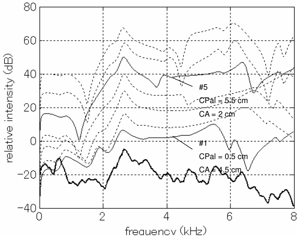
Figure 75. Spectre moyen du bruit de friction de /ʃ/ extrait de la séquence /aʃa/ (ligne épaisse, en bas) et, de bas en haut, fonctions de transfert des configurations de /ʃ/ donnant lieu à un pic proche du bruit naturel numérotées de 1 à 7 dans la Figure 74. La source de pression est localisée aux dents.
