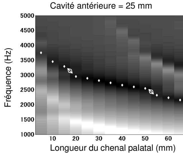
Figure 63. Nomogramme spectrographique (le gris foncé correspond à une forte intensité, c'est-à-dire les pics) pour les configurations dont la cavité antérieure est fixée à 25 mm (indiqué par une flèche dans la Figure 62), et dont la longueur du chenal palatal varie de 5 à 65 mm, avec une source dentale de pression. Les losanges blancs indiquent la fréquence de coupure détectée. Les flèches indiquent des sauts de la fréquence de coupure (voir texte).
