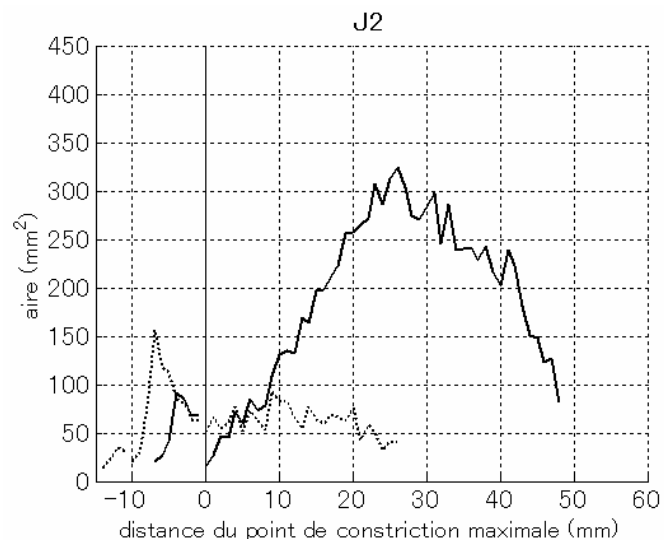
Figure 128. Fonctions d'aire de /s/ (lignes pleines) et /sʲ/ (pointillées) ; mesures effectuées sur les coupes coronales perpendiculaires aux images d'origine.
