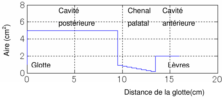
Figure 69. Fonction d'aire pour un /ʃ/ sans cavité branchante (ici, configuration palatale).
