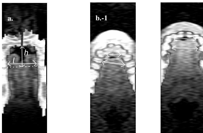
Figure 165. (a) Hauteur palatale H, largeur palatale W, et rapport largeur/hauteur sur le plan coronal, COR (sujet E2). La coupe coronale utilisée est alignée au centre des premières prémolaires. Plus l'indice est élevé, plus le palais est plat ; inversement, plus l'indice est petit, plus le palais est profond. (b) Largeur palatale pré-alvéolaire Ant ++ (espace entre les deuxièmes incisives), largeur palatale post-alvéolaire Ant + (distance entre les premières prémolaires), et indice d'arcure palatale sur le plan axial, AX, qui est le rapport de largeur pré-alvéolaire/ post-alvéolaire. Le sujet de gauche (b.-1), FR1, présente un palais en forme de V et un petit indice d'arcure axiale, tandis que le sujet de droite (b.-2), J7, présente un palais en forme de U et un indice élevé (plus proche de 1).
