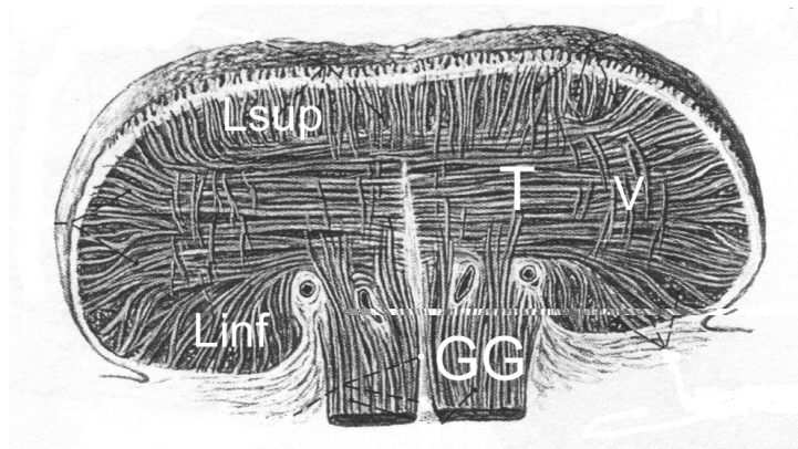
Figure 2. Principaux muscles de la langue. Linf : longitudinal inférieur ; GG : génio-glosse ; (GH : génio-hyoïde), PG : palato-glosse, SG : stylo-glosse, HG : Hyo-glosse, (Cmp : constricteur moyen du pharynx), Lsup : longitudinal supérieur, T : transverse de la langue. Image du haut : vue latérale à 80 % ; image du milieu : vue latérale, coupe médiane ; image du bas : coupe transversale à hauteur de la partie moyenne. D'après Sobotta (2000), p. 109-110.
