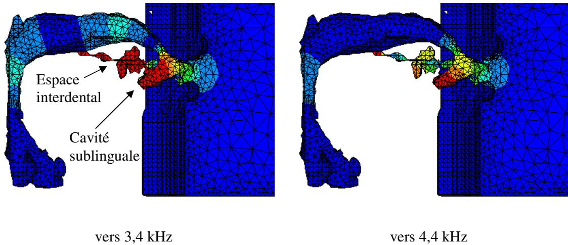
Figure 90. Distribution de pression à la fréquence des pics spectraux, à l'intérieur du conduit vocal 3D FrJ /s/_{tr} construit à partir d'un maillage de 1 mm (en correspondance avec la courbe pointillée (2) de la Figure 89). Vue de l'intérieur du conduit vocal 3D coupé en deux dans le sens sagittal. Une pression élevée est représentée en rouge ; une pression basse en bleu.
