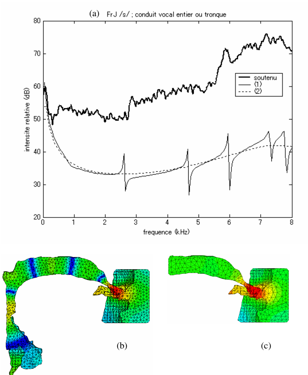
Figure 91. (a) Fonctions de transfert calculées à l'aide de la méthode des éléments finis pour /s/fr, FJ. (1), Ligne pleine : fonction de transfert d'un conduit vocal entier illustré en (b), dérivé d'un maillage de surface de 2 mm ; et (2), en ligne pointillée, pour un conduit vocal tronqué dans la région vélaire illustré en (c). Les images (b) et (c) représentent la distribution de pression à l'intérieur des conduits vocaux 3D (coupé en deux dans le sens sagittal), vers 7,8 kHz. Une source dipôle a été placée en arrière des incisives, dans la direction antéro-postérieure. Il est à noter que l'échelle des couleurs n'est pas nécessairement la même que la Figure 86.
