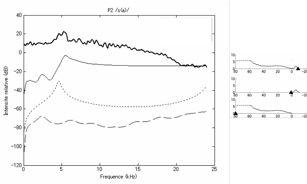
Figure 204. Spectre moyen (ligne épaisse) et fonctions de transfert obtenues avec le modèle original (source dentale), un modèle antérieur tronqué à la constriction, et un modèle postérieur. Les courbes ont été décalée de 30 dB entre elles pour une meilleure visibilité.
