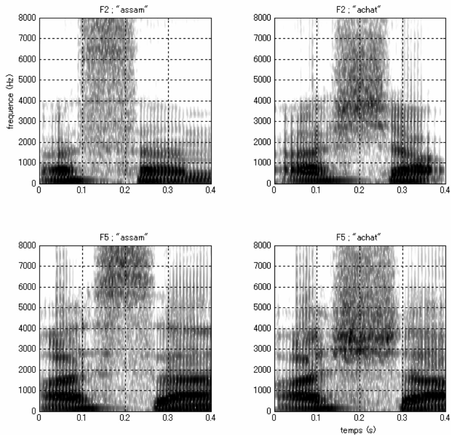
Figure 32. Spectrogrammes extraits des occurrences « Assam » (gauche) et « achat » (droite) produites en position assise par les locuteurs Fr2 (haut) et Fr5 (bas). Tous les spectrogrammes présentés dans cette thèse ont été créés dans Matlab, et ne comportent pas de pré-emphase. Les niveaux de gris correspondent donc au niveau sonore (dB).
