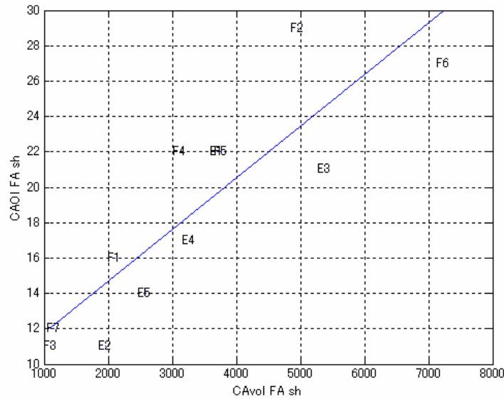
Figure 172. Volume de la cavité antérieure (CAvol) en fonction de la longueur de la cavité orale antérieure (CAOI), /sh/, français et anglais.
