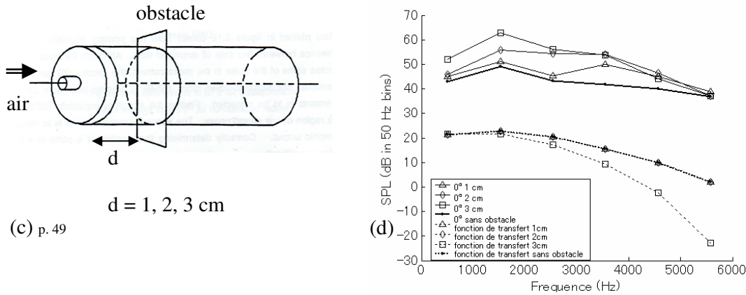
Figure 46. (a) et (c) : schéma des modèles mécaniques du conduit vocal de Shadle (1985) et « 0° avec obstacle » (le flux d'air entrant est parallèle au mode principal de résonance du modèle) de Pastel (1987), respectivement ; (b) magnitude du bruit en dB SPL obtenu par le modèle de Shadle (1985) en (a) ; avec (courbe du haut) ou sans (courbe du milieu) obstacle. En (d), magnitude du bruit en dB SPL du modèle de Pastel (1987 ; illustré en c), aux fréquences de résonance du modèle, ainsi que les fonctions de transfert théoriques. Le modèle est alimenté par un débit d'air de 442 cm 3 /sec (l'arrivée d'air se situe à gauche sur le schéma (c)). Les trois courbes du haut en (d) sont obtenues avec les configurations où l'obstacle se trouvait à 1, 2 et 3 cm en aval du flux entrant. La courbe épaisse correspond à une configuration sans obstacle. Les courbes pointillées, en bas, indiquent l'enveloppe de la fonction de transfert 65 (aux fréquences de résonance) du modèle mesurant 17 cm de long, globalement
