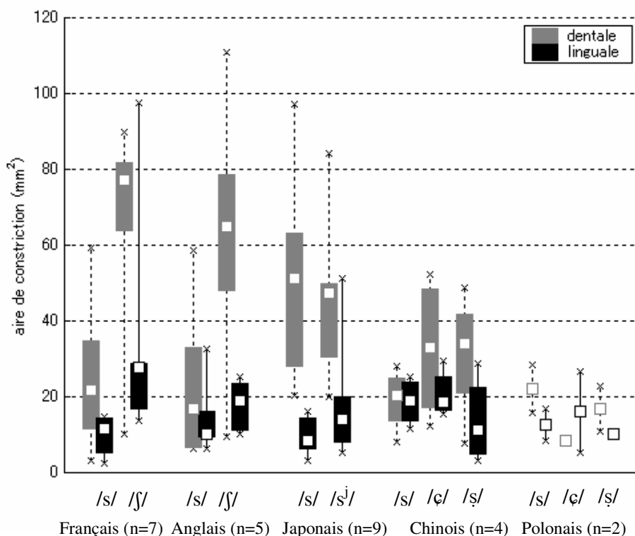
Figure 28. Taille des constriction dentales (rectangles gris et lignes pointillées) et linguale (rectangles noirs et lignes pleines) en fonction des langues et des sibilantes. Les croix indiquent les maxima et minima, les rectangles couvrent du premier au troisième quartiles et les carrés blancs indiquent le mode (ou médiane).
