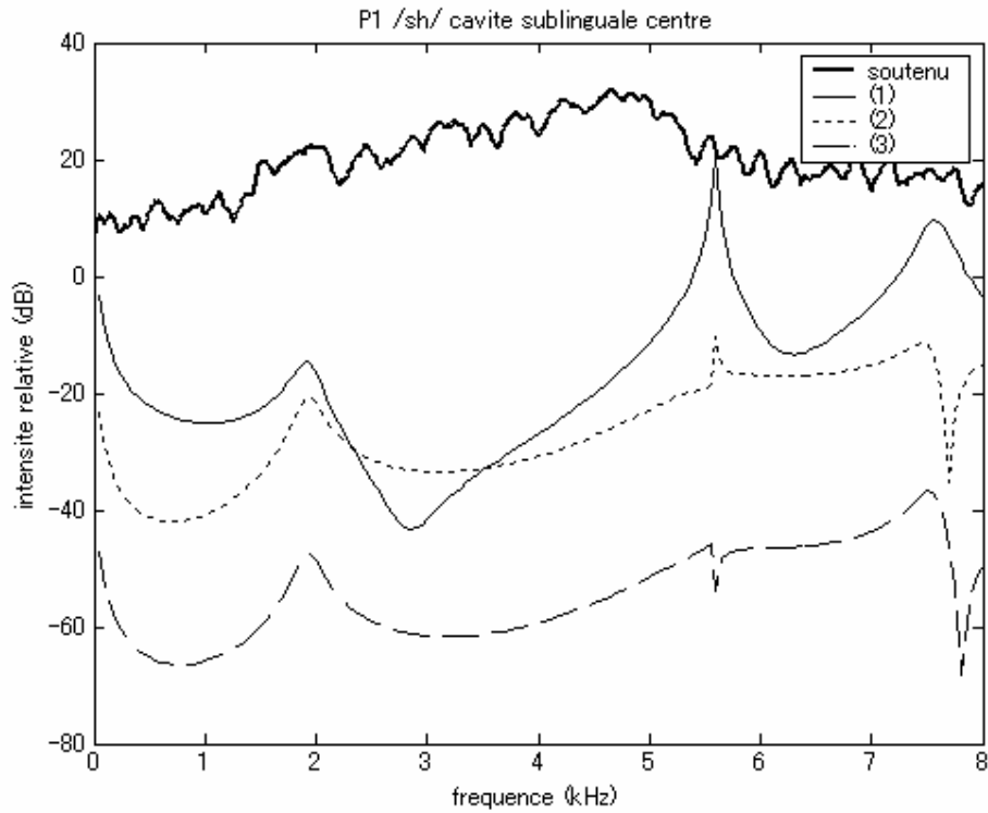
Figure 211. Spectre moyen du bruit de friction tenu (ligne foncée) et fonctions de transfert calculées à l'aide de la méthode des éléments finis pour P1 /sʃ/ (maillage de 1,5 mm) avec une source localisée au centre de la cavité orale antérieure (qui comprend une partie sublinguale). (1) Source orientée dans l'axe droite-gauche ; (2) source orientée dans l'axe antéro-postérieure ; (3) Source orientée dans l'axe haut-bas. Les fonctions de transfert sont décalées de 20 dB entre elles pour une meilleure lisibilité.
