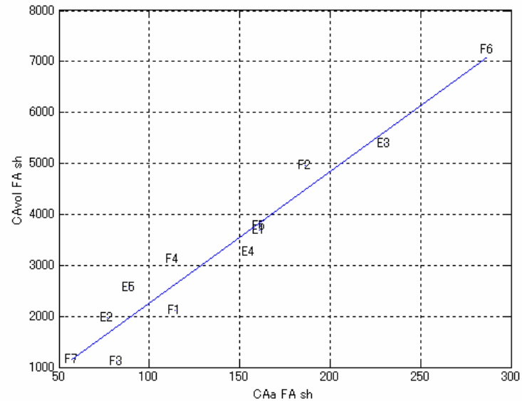
Figure 173. Volume de la cavité antérieure (CAvol) en fonction de l'aire de la cavité antérieure (CAa), /sh/, français et anglais.
