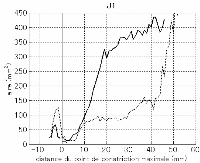
Figure 126. Fonctions d'aire de /s/ (lignes pleines) et /sj/ (pointillées) ; mesures effectuées sur les coupes coronales perpendiculaires aux images d'origine.
