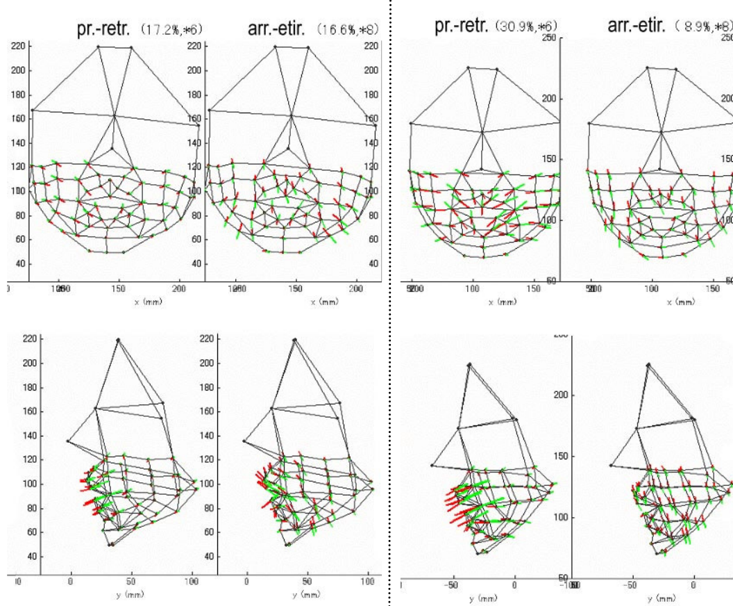
Figure 3. Facteurs labiaux pour deux locuteurs du français. Cf. Maeda et al. (2002), Toda (2001). Pour chacun des locuteurs, la première colonne représente le facteur « protrusion-rétraction » 23 et la deuxième colonne le facteur « arrondissement- étirement ». Les segments superposés au maillage représentent les vecteurs pour +/- 6 et 8 \sigma , respectivement.
