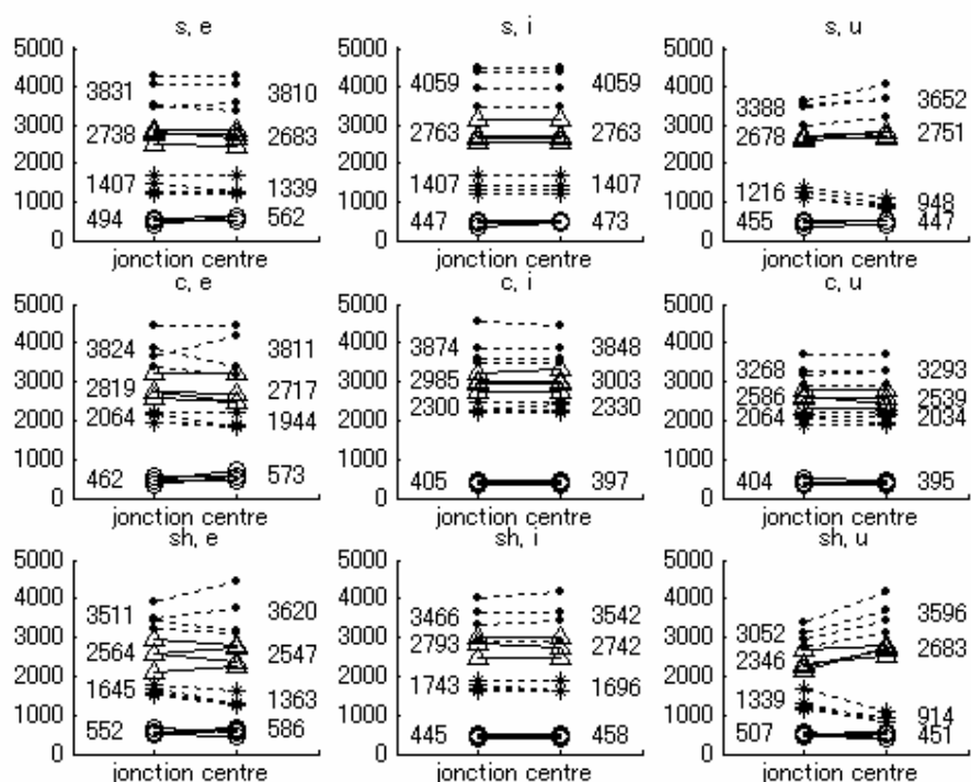
Figure 38. Fréquence des formants F1 à F4 à la jonction et à la cible pour les sibilantes /s/, /ʃ/ (représenté ‘c’) et /ɕ/ (représenté ‘sh’) du chinois. (Voir légende de la Figure 34.)
