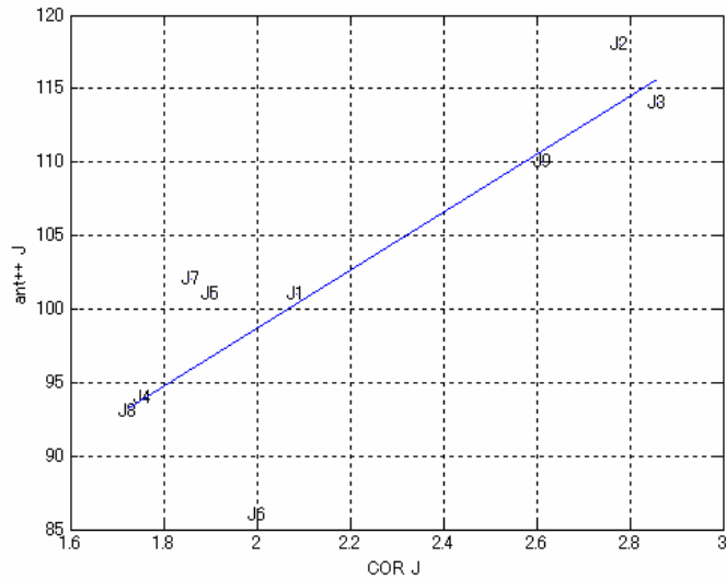
Figure 178. Largeur du palais au niveau post-alvéolaire (Ant+ en fonction de l'indice de courbure du palais sur le plan coronal (COR), japonais.
