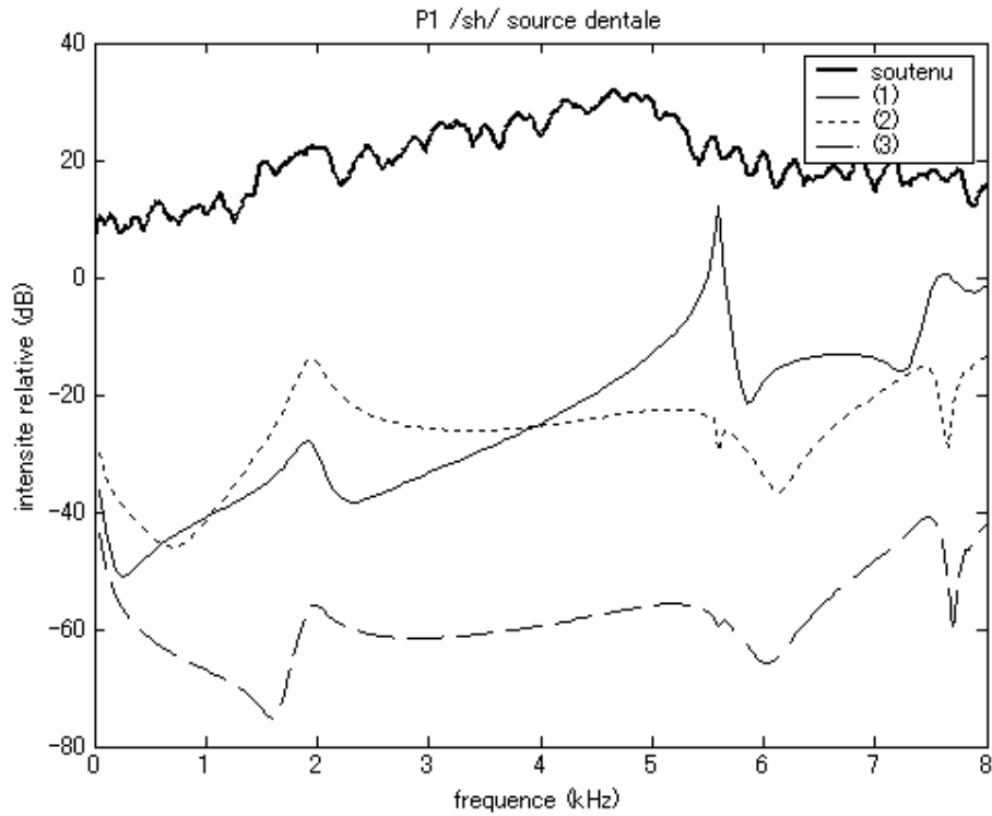
Figure 210. Spectre moyen du bruit de friction tenu (ligne foncée) et fonctions de transfert calculées à l'aide de la méthode des éléments finis pour P1 /sʃ/ (maillage de 1,5 mm) avec une source localisée en arrière de la constriction dentale. (1) Source orientée dans l'axe droite-gauche ; (2) source orientée dans l'axe antéro-postérieure ; (3) Source orientée dans l'axe haut-bas. Les fonctions de transfert sont décalées de 20 dB entre elles pour une meilleure lisibilité.
