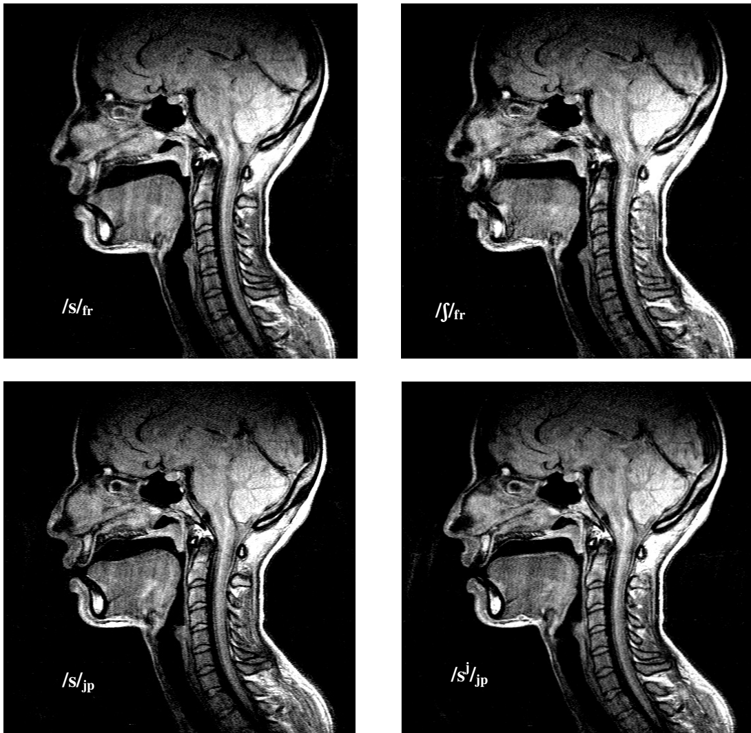
Figure 146. Coupes médio-sagittales des données IRM couvrant le conduit vocal en entier pour la locutrice FJ. Ces données, après insertion du contour
