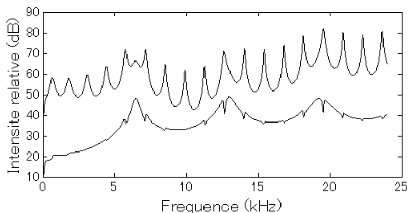
Figure 51. Fonctions de transfert d'un modèle simple de [s]. Les deux courbes sont décalées de 30 dB pour plus de clarté. La courbe supérieure correspond au résultat avec une source de pression localisée à la glotte (emplacement 1 de la Figure 50), tandis que la courbe inférieure est obtenue avec une source de pression localisée à la jonction des cavités postérieure et antérieure (emplacement 2 dans la Figure 50).
