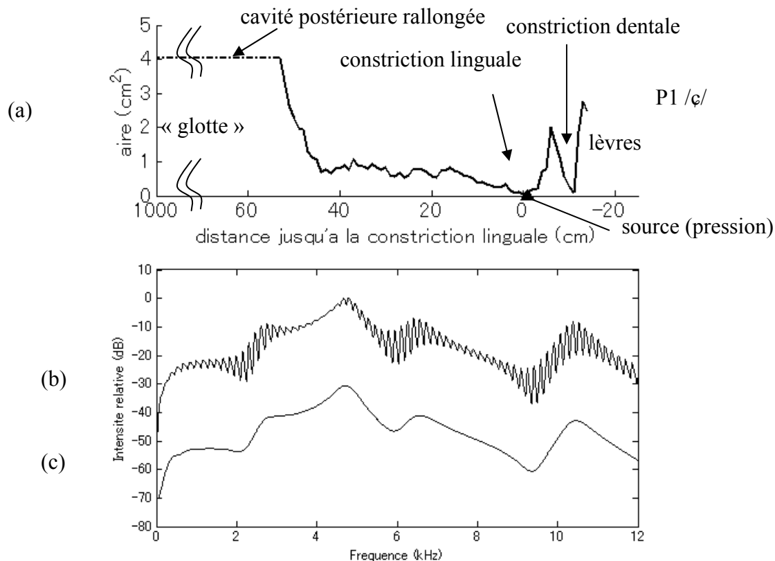
Figure 79. (a) Exemple de fonction d'aire dont la cavité postérieure a été rallongée d'un mètre, (b) sa fonction de transfert brute et (c) sa fonction de transfert après lissage cepstral.
