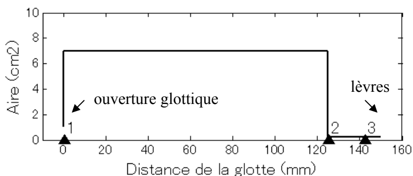
Figure 50. Configuration simple du conduit vocal pour la fricative [s], constituée de deux tubes uniformes, d'après Flanagan (1972). Les numéros indiquent les différents emplacements de la source de bruit utilisés en modélisation acoustique : à la glotte (1), à la jonction des deux tubes (2), et à 8 mm en arrière de l'extrémité labiale (3). La cavité postérieure mesure 12,5 cm pour une aire constante de 7 cm 2 ; La cavité antérieure est de 2,5 cm pour une aire de 0,2 cm 2 . L'aire de la glotte est de 1 cm 2 .
