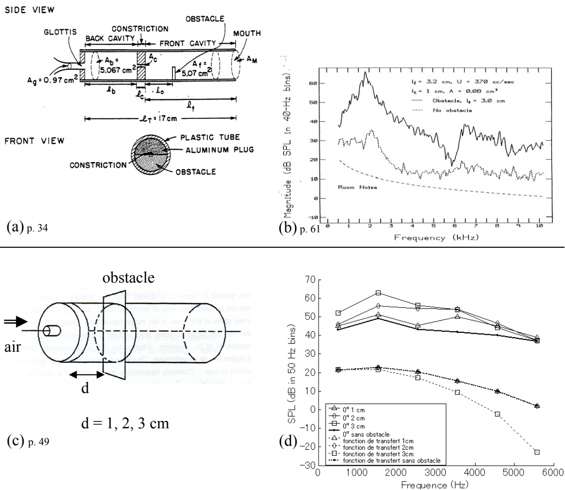
Figure 46. (a) et (c) : schéma des modèles mécaniques du conduit vocal de Shadle (1985) et « 0° avec obstacle » (le flux d'air entrant est parallèle au mode principal de résonance du modèle) de Pastel (1987), respectivement ; (b) magnitude du bruit en dB SPL obtenu par le modèle de Shadle (1985) en (a) ; avec (courbe du haut) ou sans (courbe du milieu) obstacle. En (d), magnitude du bruit en dB SPL du modèle de Pastel (1987 ; illustré en c), aux fréquences de résonance du modèle, ainsi que les fonctions de transfert théoriques. Le modèle est alimenté par un débit d'air de 442 cm 3 /sec (l'arrivée d'air se situe à gauche sur le schéma (c)). Les trois courbes du haut en (d) sont obtenues avec les configurations où l'obstacle se trouvait à 1, 2 et 3 cm en aval du flux entrant. La courbe épaisse correspond à une configuration sans obstacle. Les courbes pointillées, en bas, indiquent l'enveloppe de la fonction de transfert 64 (aux fréquences de résonances) du modèle mesurant 17 cm de long, globalement fermé à un bout (gauche) et ouvert à l'autre (droite). Données des tableaux en p. 101
