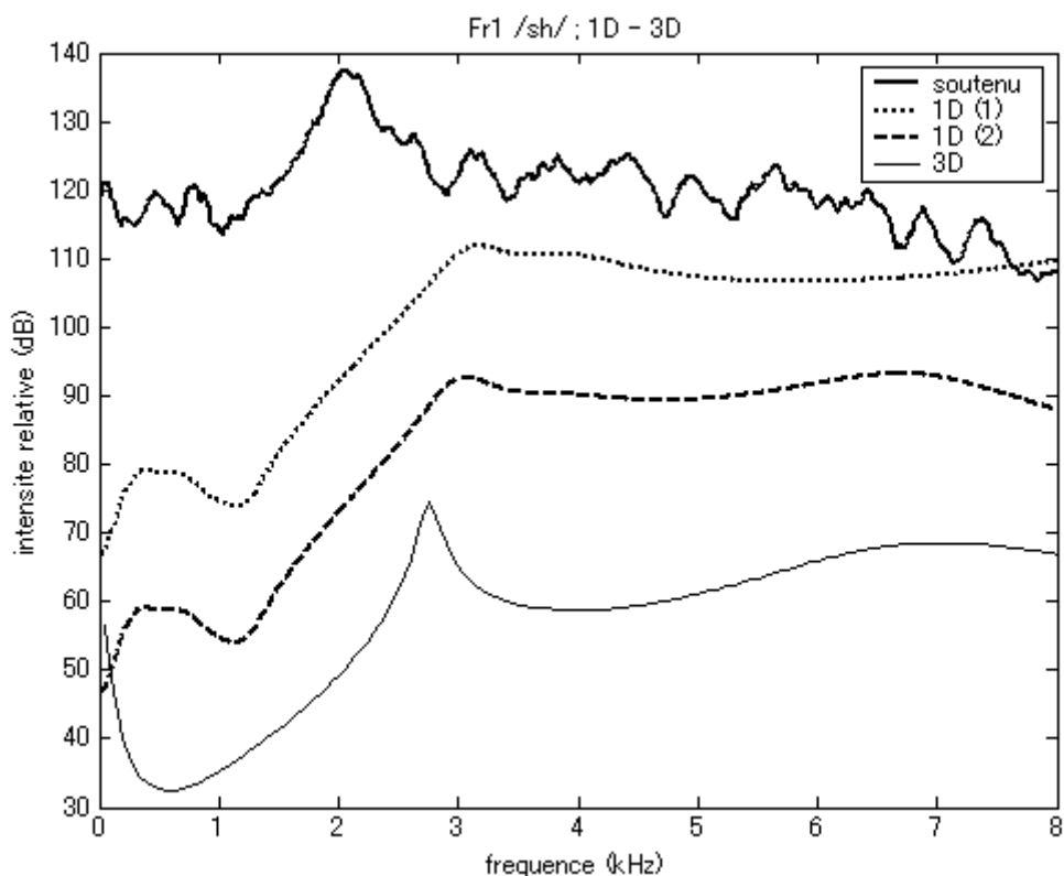
Figure 93. De haut en bas, spectre moyen d'un bruit tenu, /ʃ/, locuteur Fr1, en position allongée (ligne épaisse pleine), fonction de transfert calculée à l'aide de VTF_fric (simulation 1D) à partir de la fonctions d'aire (la fonction d'aire se trouve en Annexe III – lignes épaisses pointillées (1) et (2)), et fonction de transfert 3D, calculée à l'aide de la méthode des éléments finis (ligne fine). Source dentale dans les trois simulations. Source de pression pour la simulation 1D et source dipôle orientée dans le sens avant-arrière pour la simulation 3D. Dans la courbe 1D (2), la cavité labiale a été artificiellement prolongé par un tube uniforme, de 5 mm de long et 4 cm 2 d'aire de section.
