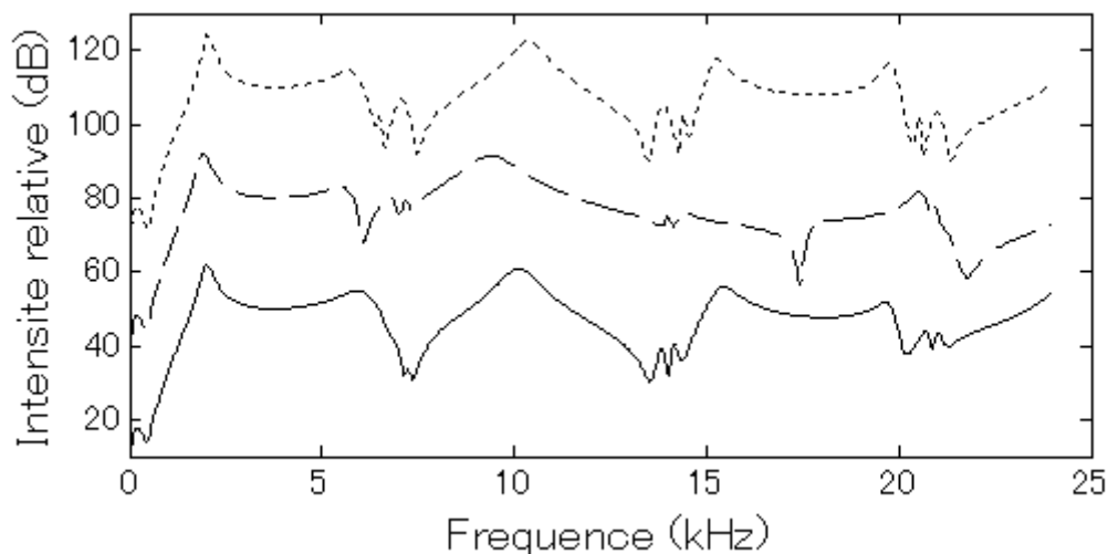
Figure 55. Fonctions de transfert de configurations du conduit vocal pour sibilante post-alvéolaire. Ligne pointillée : modèle branchant (Figure 54, haut) ; ligne interrompue : modèle branchant (Figure 54, milieu) ; ligne pleine : modèle non-branchant (Figure 54, bas). La source de pression se situe à 10 mm en arrière de l'extrémité labiale des fonctions d'aire. Les courbes sont décalées de 30 dB pour une meilleure visibilité.
