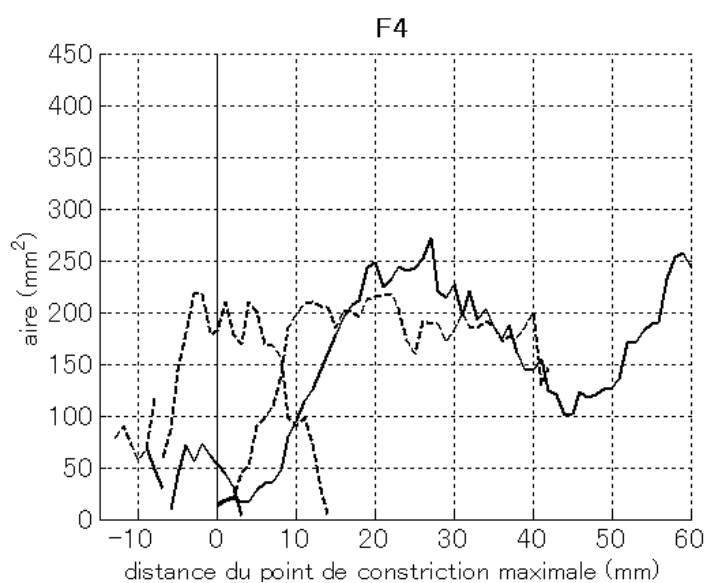
Figure 109. Fonctions d'aire de /s/ (lignes pleines) et /ʃ/ (lignes discontinues) ; mesures effectuées sur les coupes coronales perpendiculaires aux images d'origine.
