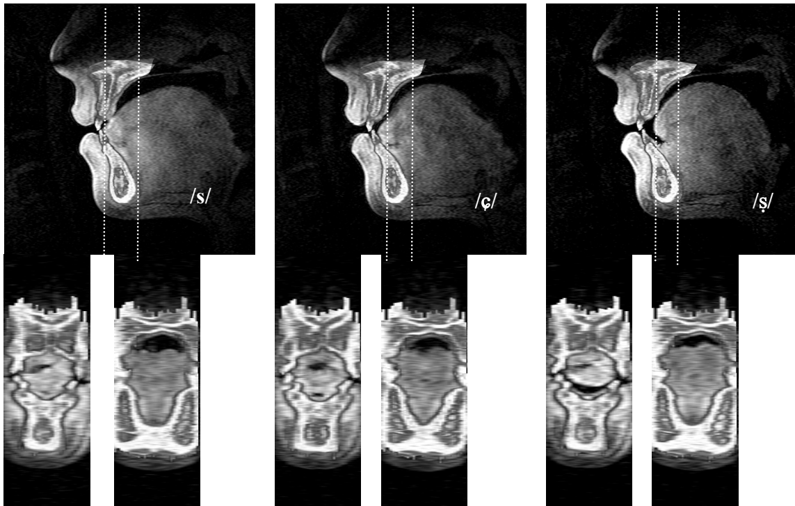
Figure 148. Coupes médio-sagittales (haut) et coronales (bas) des données IRM complétées des dents. A gauche, /s/ ; au centre, /ç/ ; à droite, /ʃ/. Les lignes pointillées blanches sur les profils sagittaux indiquent l'emplacement approximatif des coupes coronales.
