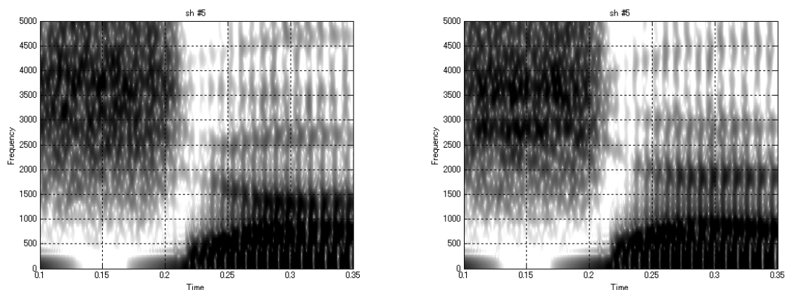
Figure 77. Spectrogrammes de la transition /ʃa/ synthétisée avec une configuration /ʃ/ de constriction longue (numéro 5). A gauche, configuration /a/ antérieur d'un rapport cavité postérieure/cavité antérieure = 1,4, et une longueur totale de 16 cm. A droite, configuration /a/ de type féminin, d'un rapport cavité postérieure/cavité antérieure = 0,5, et une longueur totale de 13 cm.
