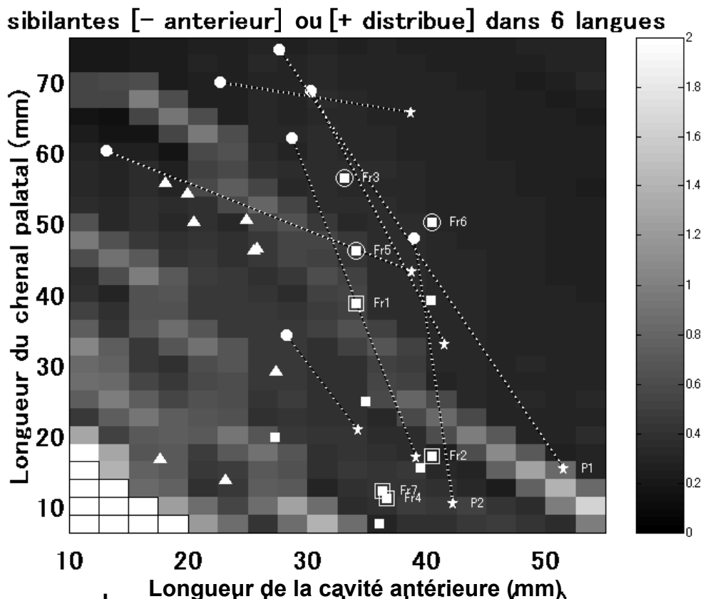
Figure 66. Dispersion des sibilantes en fonction de la longueur de la cavité antérieure et du chenal palatal mesurées sur les coupes IRM médio-sagittales et normalisée en fonction d'un facteur individuel de longueur du conduit vocal (Tableau 13), superposées aux zones de stabilité et d'instabilité acoustique prédites par simulation acoustique (source dentale ; v. légende de la Figure 61). Les triangles sont pour le /s j / japonais, les carrés pour les /ʃ/ français et anglais, les cercles pour l'alvéolo-palatale en chinois, suédois et polonais, et les étoiles pour la post-alvéolaire non palatalisée de ces trois dernières langues. Les sibilantes produites par les mêmes sujets sont connectées par des segments pointillés. En français, les données des locuteurs de la stratégie articulaire « recul » (cf. I-2) sont entourées d'un carré ; celles des locuteurs de la stratégie « déformation » par un cercle.
