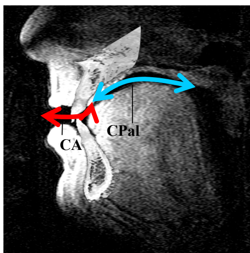
Figure 65. Mesure approximative de la longueur de la cavité antérieure (CA) et du chenal palatal (CPal) sur le profil médio-sagittal des données IRM.
