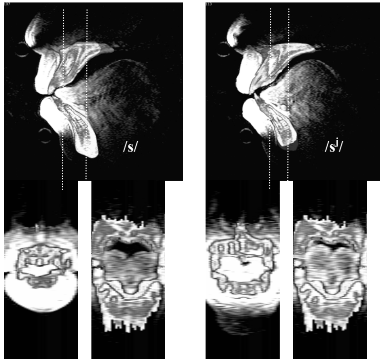
Figure 128. Coupes médio-sagittales (haut) et coronales (bas) des données IRM complétées des dents. A gauche, /s/ ; à droite, /sʲ/. Les lignes pointillées blanches sur les profils sagittaux indiquent l'emplacement approximatif des coupes coronales.
