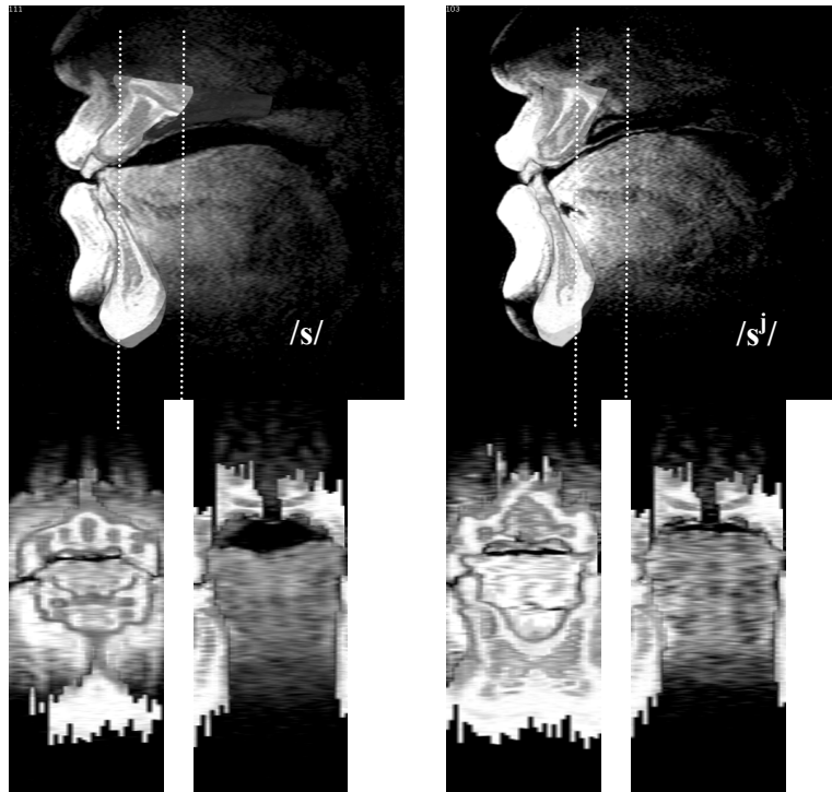
Figure 126. Coupes médio-sagittales (haut) et coronales (bas) des données IRM complétées des dents. A gauche, /s/ ; à droite, /sʲ/. Les lignes pointillées blanches sur les profils sagittaux indiquent l'emplacement approximatif des coupes coronales.
