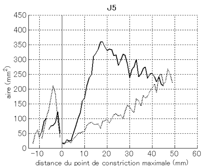
Figure 133. Fonctions d'aire de /s/ (lignes pleines) et /sʲ/ (pointillées) ; mesures effectuées sur les coupes coronales perpendiculaires aux images d'origine.
