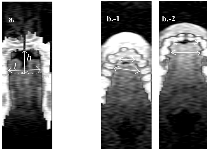
Figure 164. (a) Hauteur palatale H, largeur palatale W, et rapport largeur/hauteur sur le plan coronal, COR (sujet E2). La coupe coronale utilisée est alignée au centre des premières prémolaires. Plus l'indice est élevé, plus le palais est plat ; inversement, plus l'indice est petit, plus le palais est profond. (b) Largeur palatale pré-alvéolaire Ant ++ (espace entre les deuxièmes incisives), largeur palatale post-alvéolaire Ant + (distance entre les premières prémolaires), et indice d'arcure palatale sur le plan axial, AX, qui est le rapport de largeur pré-alvéolaire/ post-alvéolaire. Le sujet de gauche (b.-1), FR1, présente un palais en forme de V et un petit indice d'arcure axiale, tandis que le sujet de droite (b.-2), J7, présente un palais en forme de U et un indice élevé (plus proche de 1).
