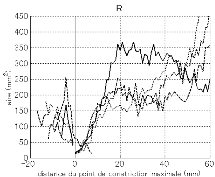
Figure 162. Fonctions d'aire ; mesures effectuées sur les coupes coronales perpendiculaires aux images d'origine. Lignes pleines : /s/ ; lignes interrompues par des points : /sj/ ; lignes interrompues /ʃ/ ; lignes pointillées : /ç/.
