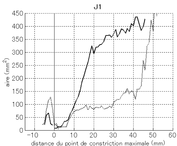
Figure 125. Fonctions d'aire de /s/ (lignes pleines) et /sj/ (pointillées) ; mesures effectuées sur les coupes coronales perpendiculaires aux images d'origine.
