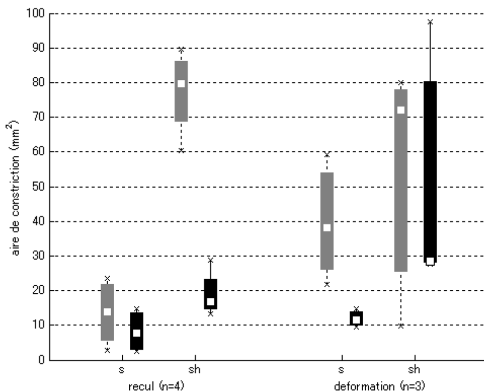
Figure 29. Taille des constrictions dentale (rectangles gris et lignes pointillées) et linguale (rectangles noirs et lignes pleines) en français (/s/ et /ʃ/ 'sh'), locuteurs groupés par type articulaire « recul » (Fr1, Fr2, Fr4, Fr7) et « déformation » (Fr3, Fr5, Fr6) ; cf. I-3.
