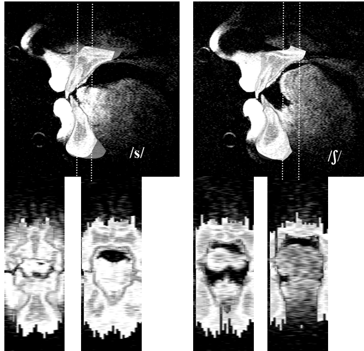
Figure 110. Coupes médio-sagittales (haut) et coronales (bas) des données IRM complétées des dents. A gauche, /s/ ; à droite, /ʃ/. Les lignes pointillées blanches sur les profils sagittaux indiquent l'emplacement approximatif des coupes coronales.
