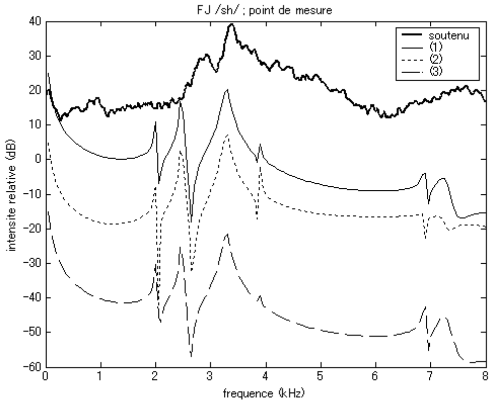
Figure 212. Spectre moyen du bruit de friction tenu (ligne foncée) et fonctions de transfert calculées à l'aide de la méthode des éléments finis pour FJ /ʃ/fr (maillage de 1 mm ; modèle tronqué à la constriction linguale) avec une source localisée en arrière de la constriction dentale et orientée dans l'axe antéro-postérieur. (1) Pression mesurée en avant, vers le bas gauche de l'espace de rayonnement ; (2) pression mesurée vers le centre de l'espace de rayonnement ; (3) pression mesurée vers le bas, à gauche, de l'espace de rayonnement, près du visage. Les fonctions de transfert sont décalées de 20 dB entre elles pour une meilleure lisibilité.
