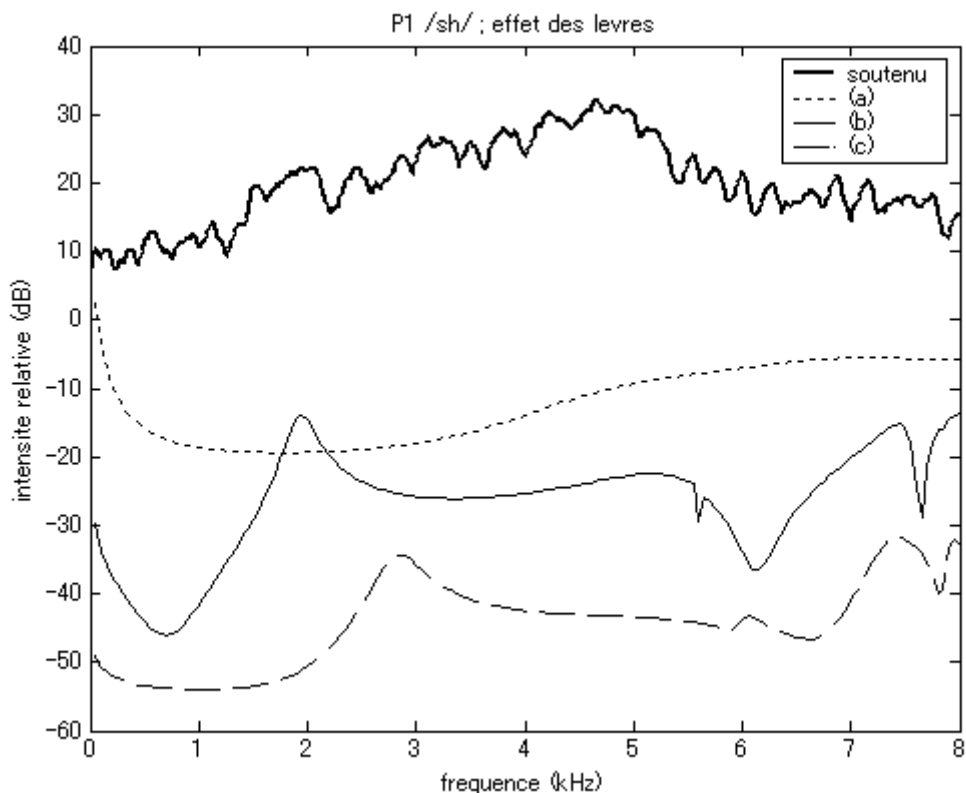
Figure 97. De haut en bas, spectre moyen du bruit de friction tenu (ligne épaisse) et fonctions de transfert calculées à l'aide de la méthode des éléments finis, pour P1 / \text{ʃ} / ; maillage de 1,5 mm. (a) Les lèvres seulement (conduit vocal 3D tronqué à la constriction dentale), avec une source localisée en avant de la constriction dentale ; (b) conduit vocal 3D original, des lèvres jusqu'à la région vélaire; (c) sans les lèvres (couvrant de la région vélaire jusqu'à la constriction dentale), avec une source derrière la constriction dentale.
