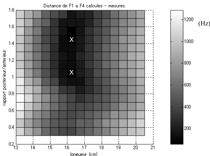
Figure 71. Fonction de distance des formants F1 à F4 calculés et mesurés, basée sur la somme des carrés, exprimée en niveaux de gris, pour le locuteur Fr8. Les axes horizontale et verticale correspondent aux paramètres articulatoires de la configuration /a/ (Figure 69). Les formants F1 à F4 mesurés pendant la partie stable de la voyelle /a/ postconsonantique pour le locuteur Fr8 étaient de 734, 1368, 2690, 3488 Hz, respectivement.
