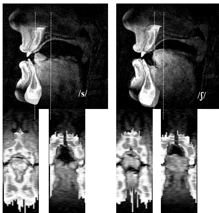
Figure 114. Coupes médio-sagittales (haut) et coronales (bas) des données IRM complétées des dents. A gauche, /s/ ; à droite, /ʃ/. Les lignes pointillées blanches sur les profils sagittaux indiquent l'emplacement approximatif des coupes coronales.
