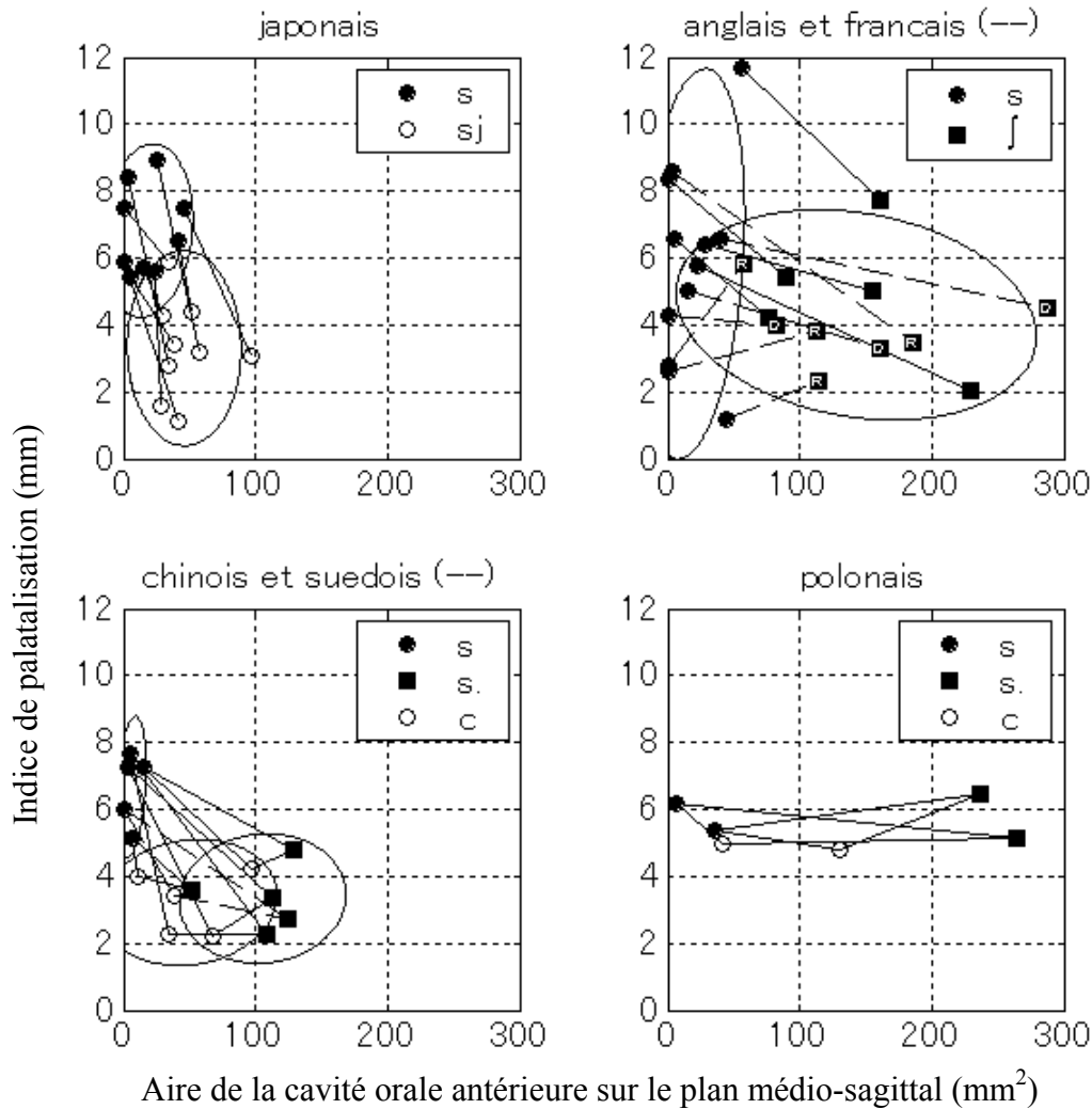
Figure 27. Dispersion des sibilantes dans l'espace articulatoire défini par l'aire de la cavité orale antérieure sur le plan médo-sagittal et l'indice de palatalisation (voir texte) en fonction du système phonologique des langues. Les ellipses correspondent à +/- 2 écarts types. En français, les /ʃ/ de la stratégie « recul » sont marqués par la lettre « R » et ceux de la stratégie « déformation » par la lettre « D ».
