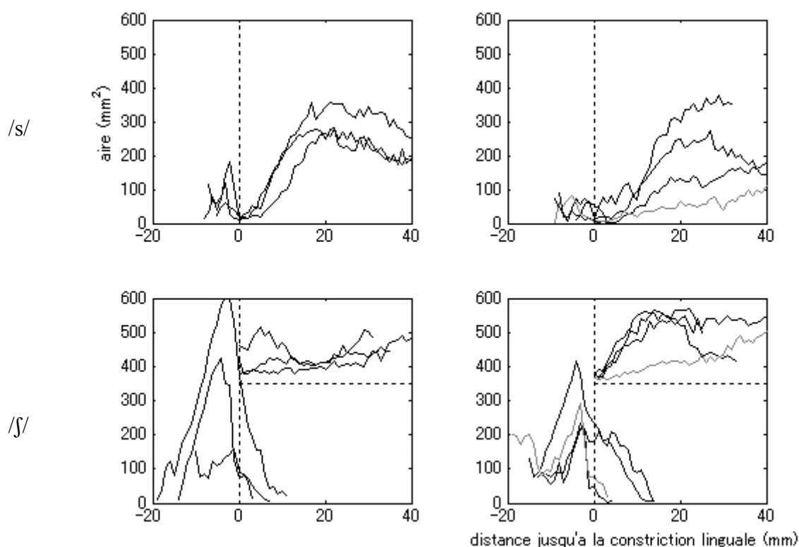
Figure 23. Fonction d'aire de /s/ et /ʃ/ pour deux groupes locuteurs du français classés en fonction de la manière dont ils réalisent le contraste entre /s/ et /ʃ/. Toutes les courbes sont alignées au point de constriction linguale maximale (0 mm ; les lèvres se situent à gauche). Pour /ʃ/, la partie postérieure à la constriction est décalée vers le haut pour améliorer la visibilité. Sa ligne de base se situe à 350 mm 2 . La partie de la cavité antérieure qui dépasse en arrière du point de constriction maximal correspond à la cavité sublinguale.
