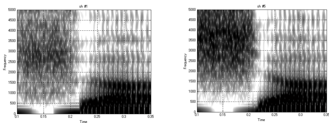
Figure 75. Spectrogrammes de la transition /ʃa/ synthétisée à l'aide de vcvSynt. La configuration cible /a/ est caractérisée par un rapport cavité postérieure/cavité antérieure = 0,9 et une longueur totale de 16 cm. A gauche, configuration cible /ʃ/ de constriction courte (numéro 1 ; cavité antérieure de 45 mm et constriction de 5 mm) et à droite, de constriction longue (numéro 5 ; cavité antérieure de 15 mm et chenal palatal de 55 mm).
