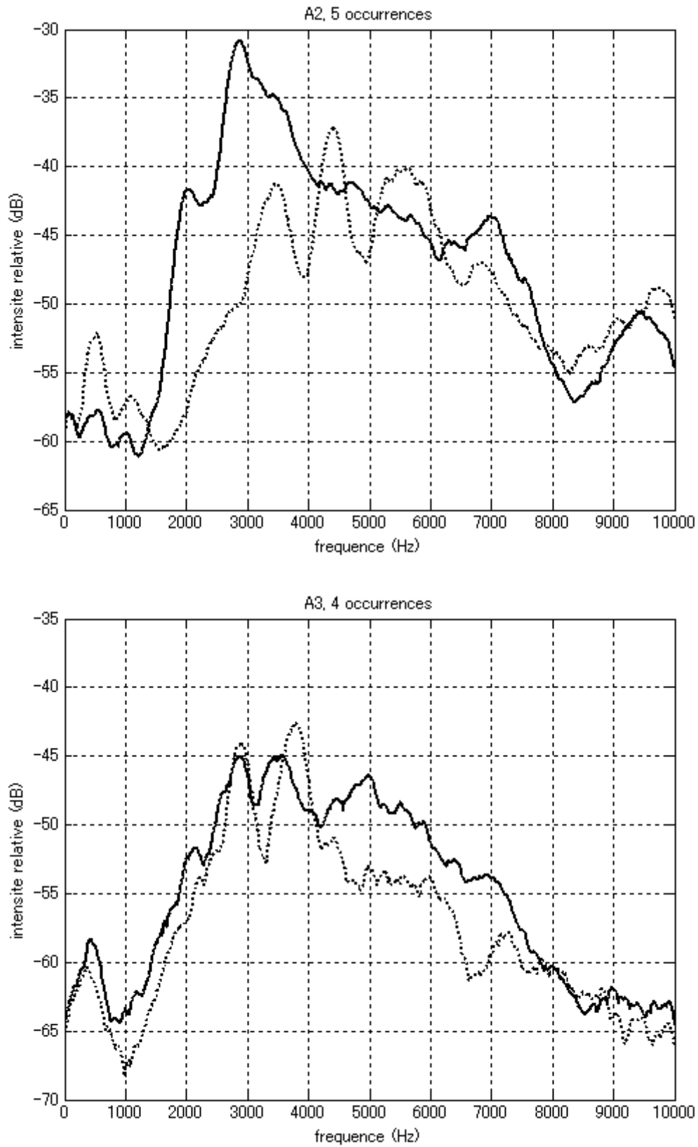
Figure 98. Spectre moyen (moyenne de la portion centrale de 4 ou 5 occurrences) des
