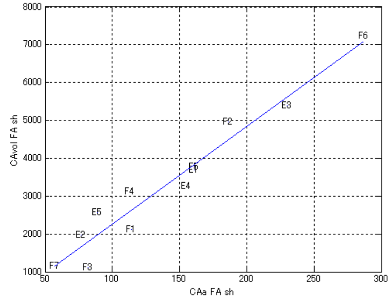
Figure 172. Volume de la cavité antérieure (CAvol) en fonction de l'aire de la cavité antérieure (CAa), /sh/, français et anglais.
