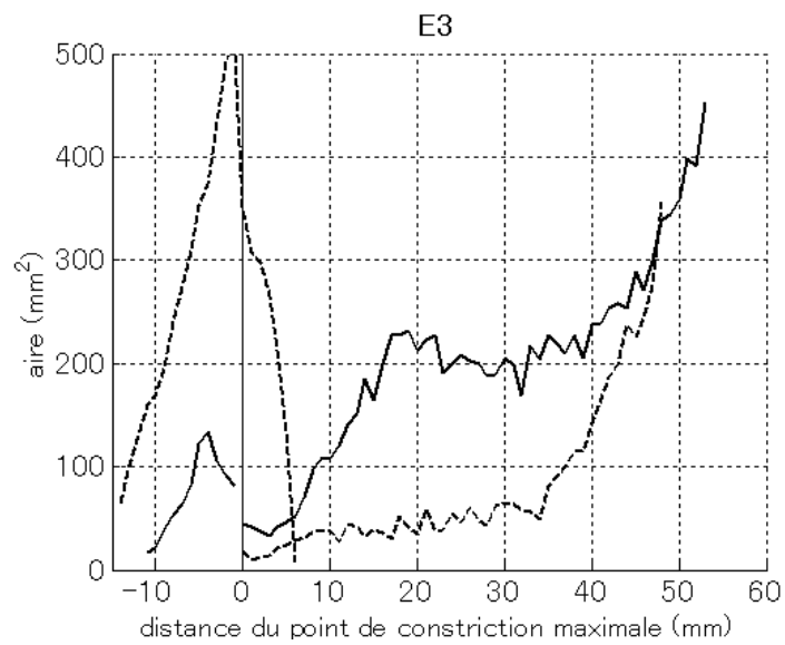
Figure 119. Fonctions d'aire de /s/ (lignes pleines) et /ʃ/ (lignes discontinues) ; mesures effectuées sur les coupes coronales perpendiculaires aux images d'origine.
