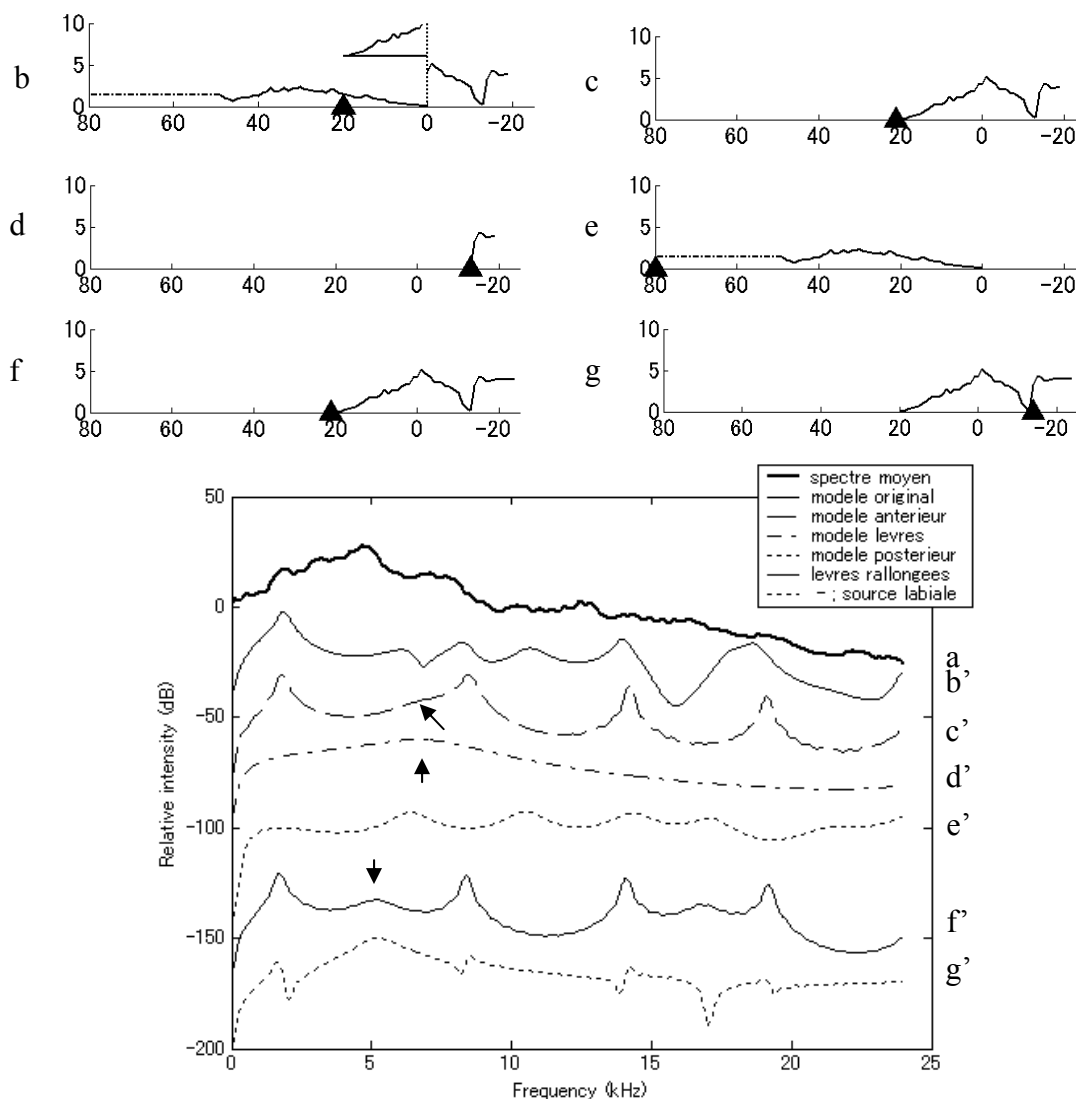
Figure 80. Fonctions d'aire de six configurations de /s/ du locuteur P1 (petites figures du haut, de b à g), le spectre moyen du bruit de friction enregistré (figure du bas, ligne épaisse a), et les fonctions de transfert (lignes fines, de b' à g') calculées pour chacune des configurations. Dans les fonctions d'aire, l'axe horizontal représente la distance
