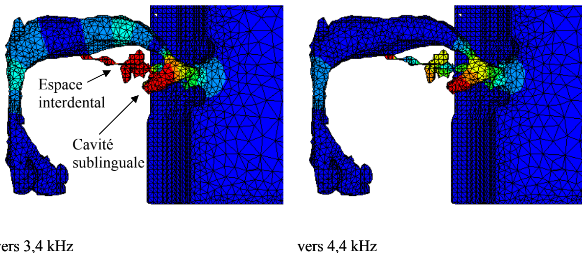
Figure 89. Distribution de pression à la fréquence des pics spectraux, à l'intérieur du conduit vocal 3D FrJ / f_{fr} construit à partir d'un maillage de 1 mm (en correspondance avec la courbe pointillée (2) de la Figure 88). Vue de l'intérieur du conduit vocal 3D coupé en deux dans le sens longitudinal. Une pression élevée est représentée en rouge ; une pression basse en bleu.
