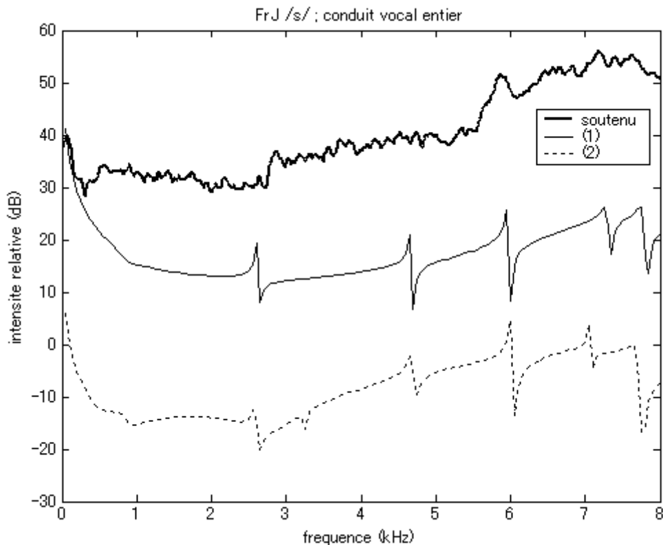
Figure 84. Spectre de bruit de friction tenu (ligne épaisse) et fonctions de transfert calculées à l'aide de la méthode des éléments finis (lignes fines) pour le /s/fr de la locutrice FrJ. (1) fonction de transfert calculée avec un conduit vocal issu d'un maillage de surface dont les segments mesuraient environ 2 mm ; (2) conduit vocal issu d'un maillage de 1 mm. Les fonctions de transfert sont décalées entre elles de 20 dB pour plus de clarté.
