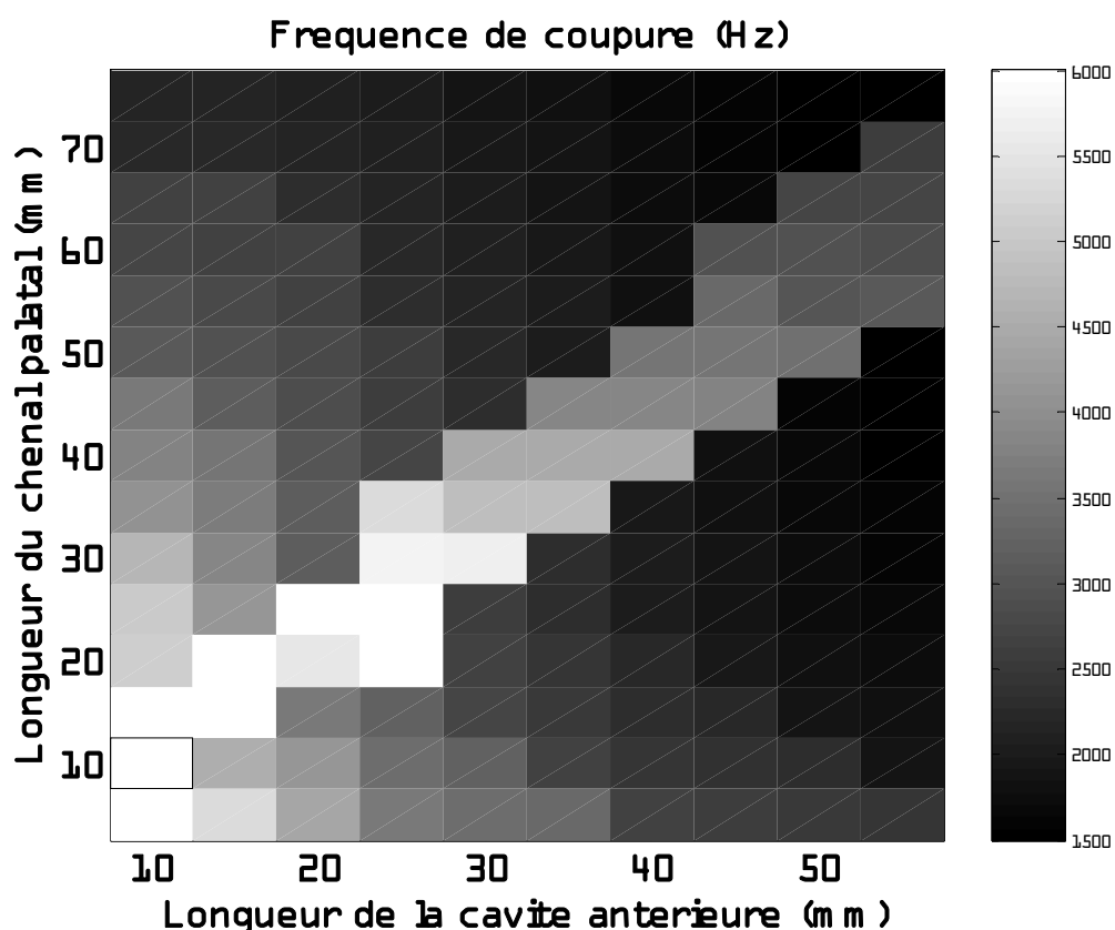
Figure 63. Fréquence de coupure (exprimée en niveaux de gris) des fonctions de transfert obtenues par simulation acoustique pour une source palatale de pression. L'axe horizontal correspond à la longueur de la cavité antérieure et l'axe vertical à la longueur du chenal palatal.
