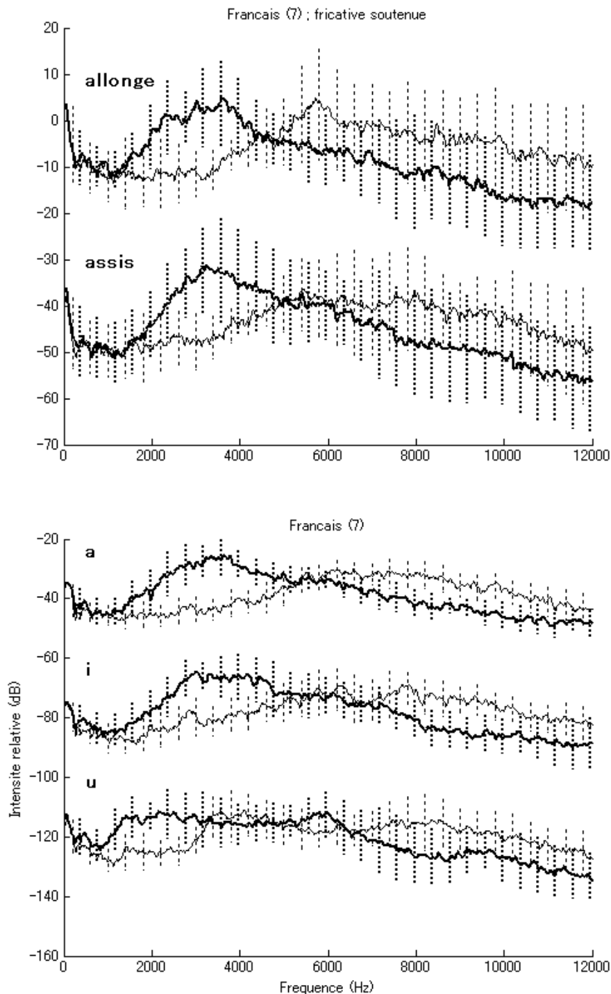
Figure 41. Spectres moyens, tous locuteurs confondus, pour le français. Les lignes épaisses correspondent à /ʃ/ et les lignes fines à /s/. Les segments hachurés correspondent à \pm 1 écart type. Le panneau du haut montre les spectres moyens de production tenue, en positions assise ou allongée. Le panneau du bas présente les spectres moyens dans différents contextes vocaliques. Les ensembles de courbes ont été décalés de 40 dB chacun pour une meilleure visibilité.
