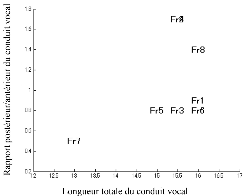
Figure 70. Configurations de la voyelle /a/ définies par leur longueur totale (axe
