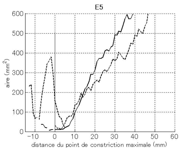
Figure 123. Fonctions d'aire de /s/ (lignes pleines) et /ʃ/ (lignes discontinues) ; mesures effectuées sur les coupes coronales perpendiculaires aux images d'origine.
