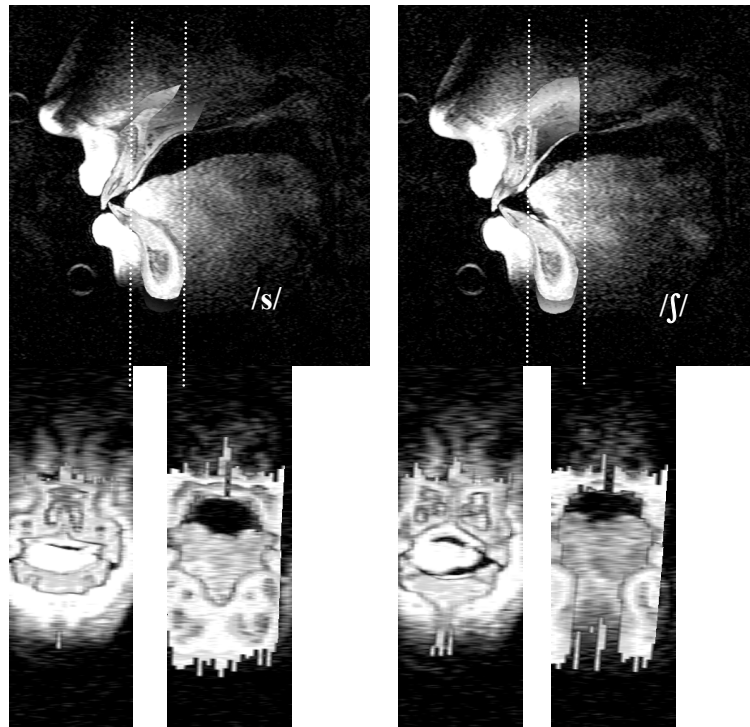
Figure 143. Coupes médio-sagittales (haut) et coronales (bas) des données IRM pour le français, produite par la locutrice bilingue FrJ, complétées des dents. A gauche, /s/ ; à droite, /sʰ/. Les lignes pointillées blanches sur les profils sagittaux indiquent l'emplacement approximatif des coupes coronales.
