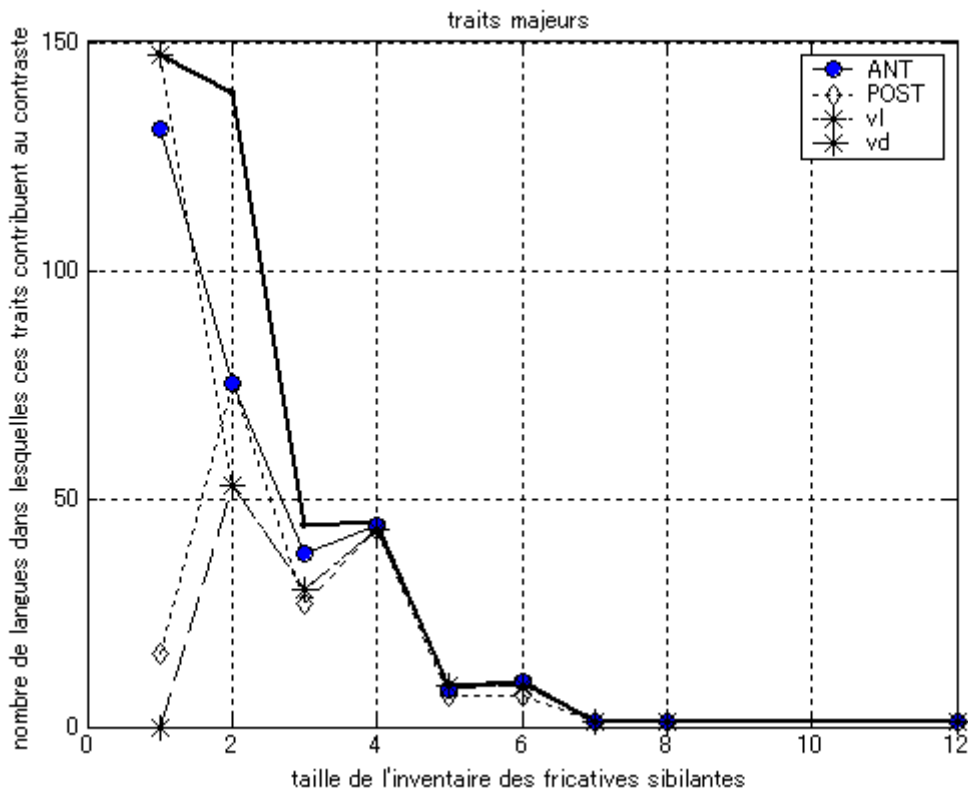
Figure 99. Nombre d'occurrences des traits distinctifs (sauf lorsque la taille de l'inventaire est égale à 1 ; dans ce cas les traits ne sont pas nécessairement distinctifs) les plus utilisés (lieux génériques et voisement) en fonction de la taille de l'inventaire des fricatives sibilantes (sourdes et sonores confondues) d'après la base de données UPSID. La courbe foncée représente le nombre total de langues pour chaque taille de l'inventaire.
