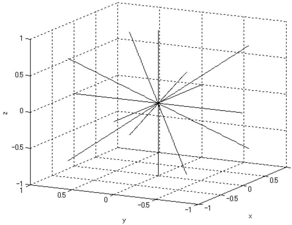
Figure 207. Axes d'orientation de la source (cf. Figure 208).
