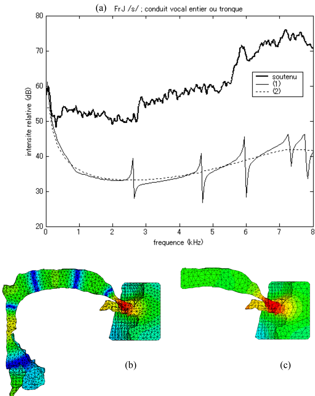
Figure 90. (a) Fonctions de transfert calculées à l'aide de la méthode des éléments finis pour /s/ fr , FJ. (1), Ligne pleine : fonction de transfert d'un conduit vocal entier illustré en (b), dérivé d'un maillage de surface de 2 mm ; et (2), en ligne pointillée, pour un conduit vocal tronqué dans la région vélaire illustré en (c). Les images (b) et (c) représentent la distribution de pression à l'intérieur des conduits vocaux 3D (coupé en deux dans le sens longitudinal), vers 7,8 kHz. Une source dipôle a été placée en arrière des incisives, dans la direction antéro-postérieure. Il est à noter que l'échelle des couleurs n'est pas nécessairement la même que la Figure 85.
