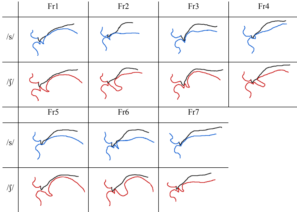
Figure 16. Profils médio-sagittaux des sept locuteurs du français
