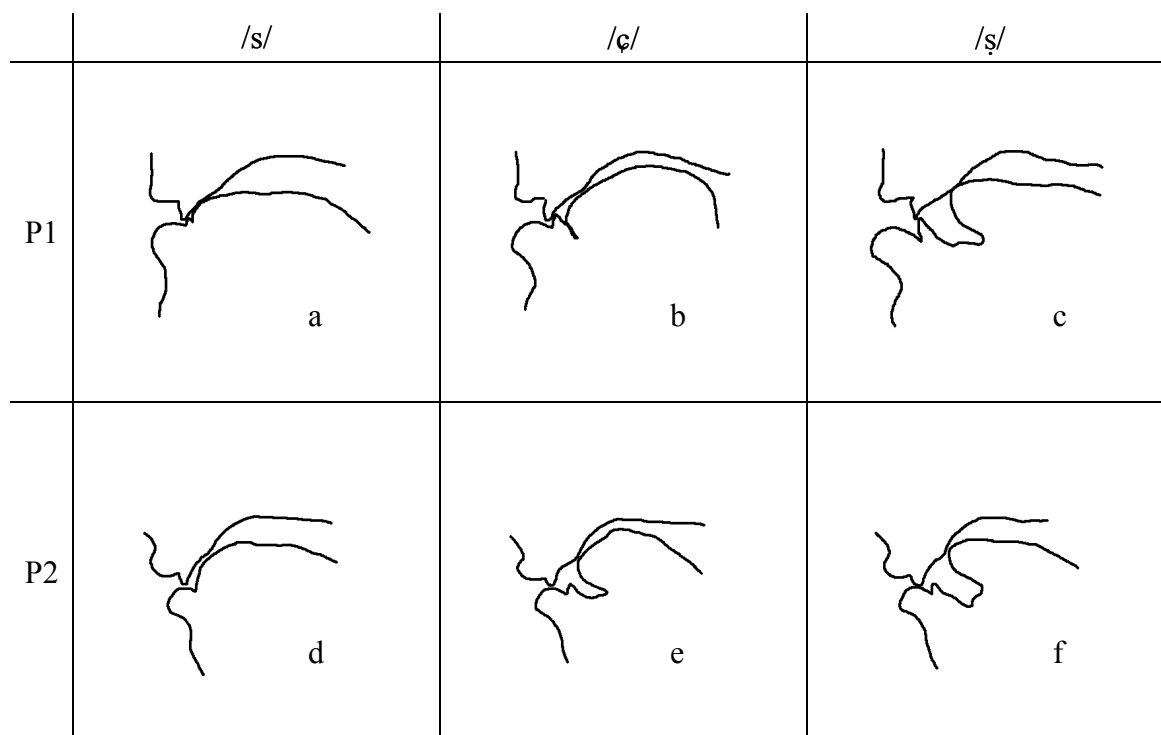
Figure 19. Contours médio-sagittaux des sibilantes du polonais.
