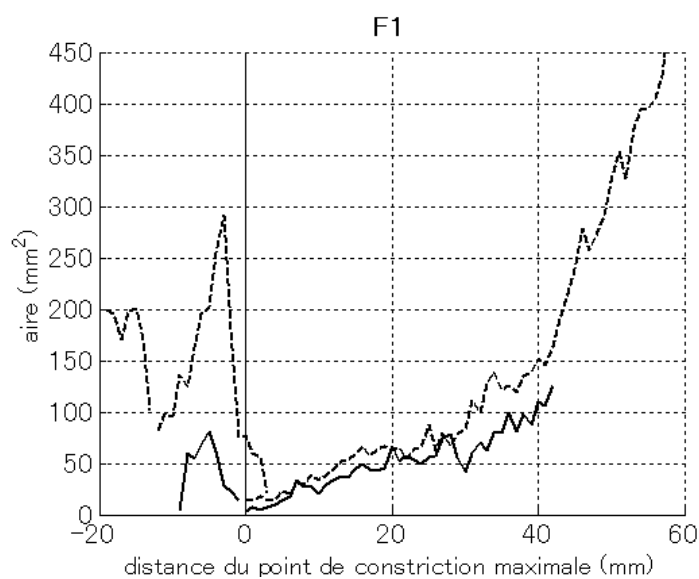
Figure 105. Fonctions d'aire de /s/ (lignes pleines) et /ʃ/ (lignes discontinues) ; mesures effectuées sur les coupes coronales perpendiculaires aux images d'origine.
