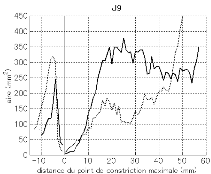
Figure 142. Fonctions d'aire de /s/ (lignes pleines) et /sʲ/ (pointillées) ; mesures effectuées sur les coupes coronales perpendiculaires aux images d'origine.
