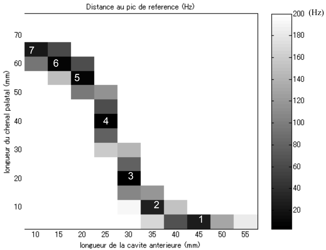
Figure 73. Distance de la fréquence de coupure des fonctions de transfert au pic de référence du locuteur Fr8 (2660 Hz) représentée en niveaux de gris. L'axe horizontal correspond à la longueur de la cavité antérieure et l'axe vertical à la longueur du chenal palatal (la configuration du conduit vocal pour / ʃ / est illustrée en Figure 68).
