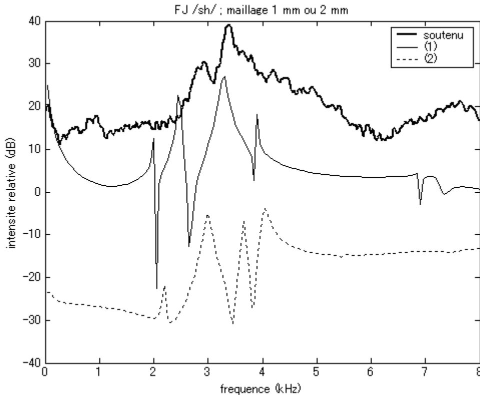
Figure 204. Spectre moyen du bruit de friction tenu (ligne foncée) et fonctions de transfert calculées à l'aide de la méthode des éléments finis. (1) Conduit vocal 3D tronqué dans la région vélaire, construit à partir d'un maillage de 1 mm ; (2) conduit vocal 3D tronqué dans la région vélaire, construit à partir d'un maillage de 2 mm. Les fonctions de transfert sont décalées entre elles de 20 dB pour une meilleure lisibilité.
