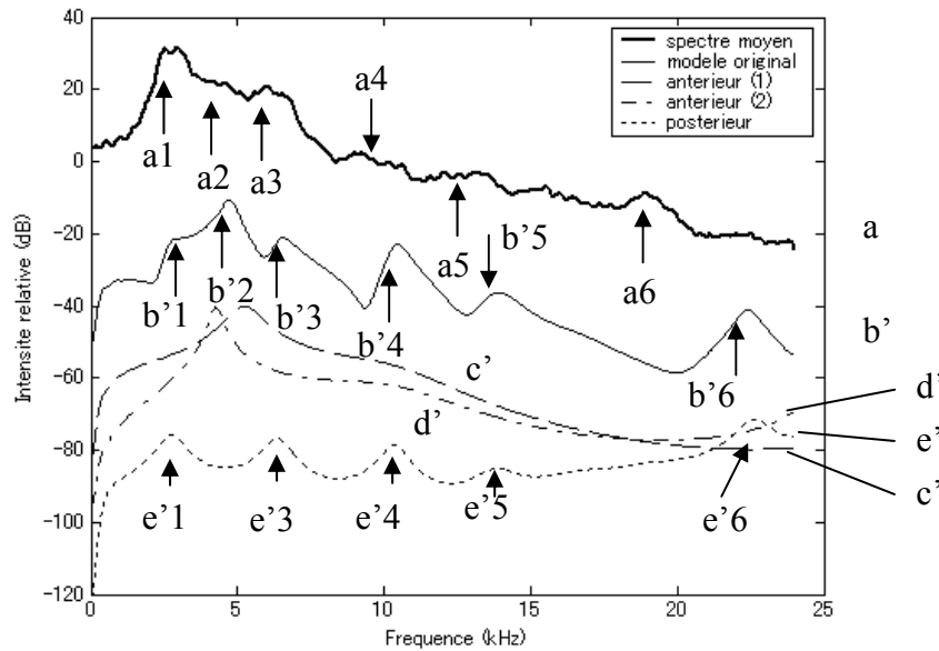
Figure 82. En haut, configurations variées du conduit vocal pour /ç/, P1. En bas, spectre moyen (ligne épaisse a) et fonctions de transfert (lignes fines b' à e'). La première fonction de transfert (b') est pour la configuration originale (de la région vélaire aux lèvres) avec une source de pression localisée dans la constriction. Les deux courbes suivantes correspondent à la cavité antérieure. La fonction de transfert c', dont le pic spectral principal a une fréquence plus élevée, a été obtenue avec une extrémité tronquée (au niveau de la constriction linguale) fermée, et la fonction de transfert d', avec une extrémité tronquée ouverte (et rallongée de 1 m). La dernière fonction de transfert correspond à la cavité postérieure (e). Dans ces trois dernières simulations, une source de pression localisée à l'extrémité arrière du conduit vocal a été utilisée. Les courbes ont été décalées de 30 dB entre elles pour une meilleure visibilité.
