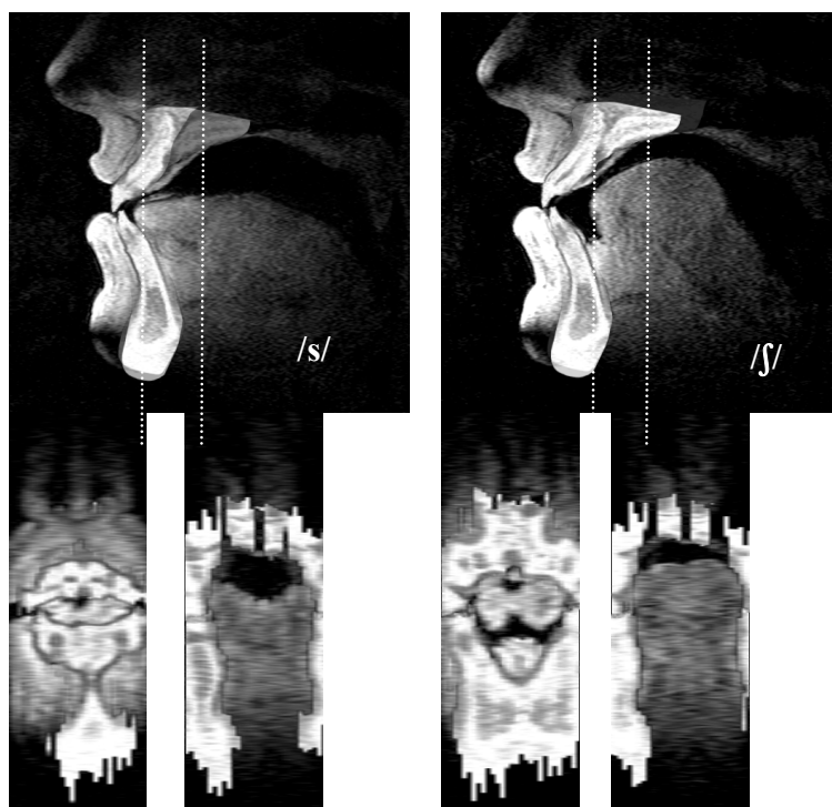
Figure 120. Coupes médio-sagittales (haut) et coronales (bas) des données IRM complétées des dents. A gauche, /s/ ; à droite, /ʃ/. Les lignes pointillées blanches sur les profils sagittaux indiquent l'emplacement approximatif des coupes coronales.
