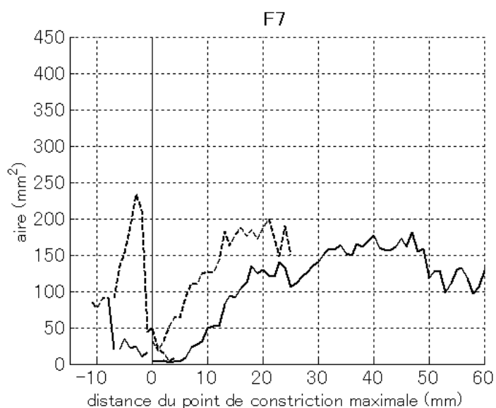
Figure 113. Fonctions d'aire de /s/ (lignes pleines) et /ʃ/ (lignes discontinues) ; mesures effectuées sur les coupes coronales perpendiculaires aux images d'origine.
