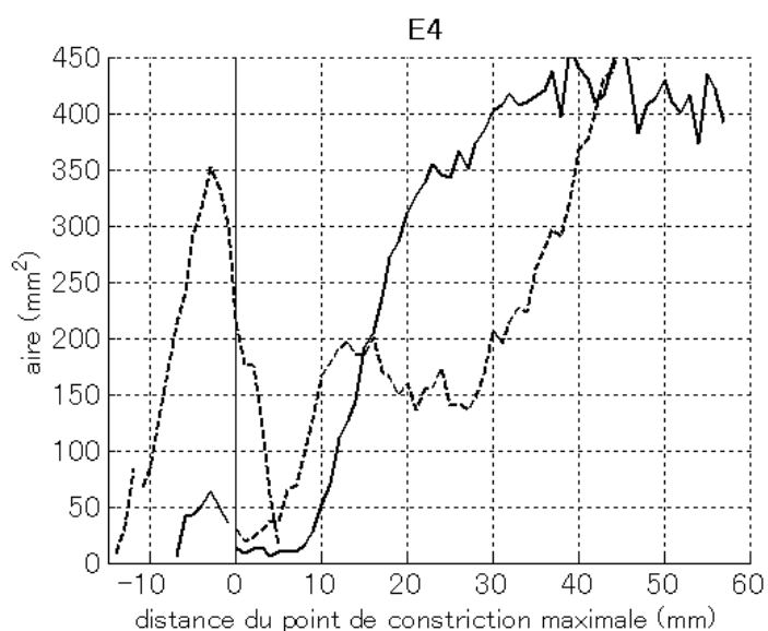
Figure 121. Fonctions d'aire de /s/ (lignes pleines) et /ʃ/ (lignes discontinues) ; mesures effectuées sur les coupes coronales perpendiculaires aux images d'origine.
