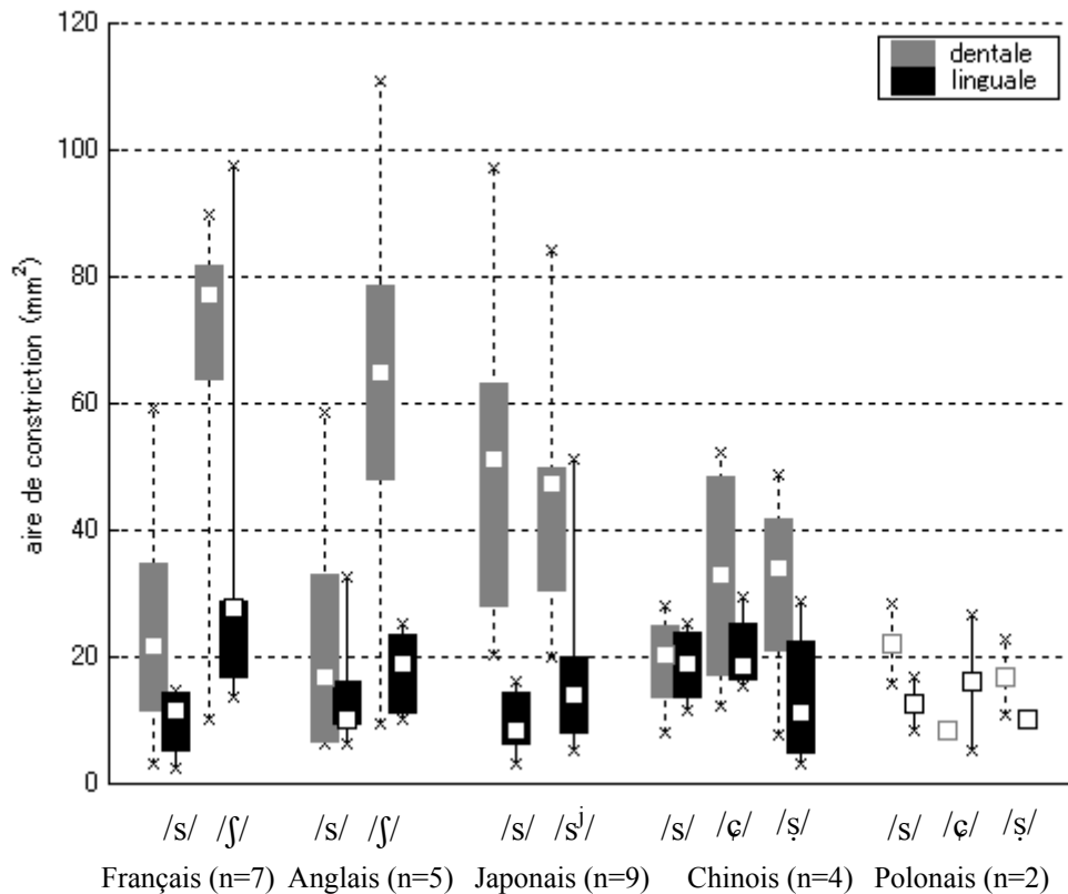
Figure 28. Taille des constrictions dentales (rectangles gris et lignes pointillées) et linguale (rectangles noirs et lignes pleines) en fonction des langues et des sibilantes. Les croix indiquent les maxima et minima, les rectangles couvrent du premier au troisième quartiles et les carrés blancs indiquent le mode (ou médiane).
