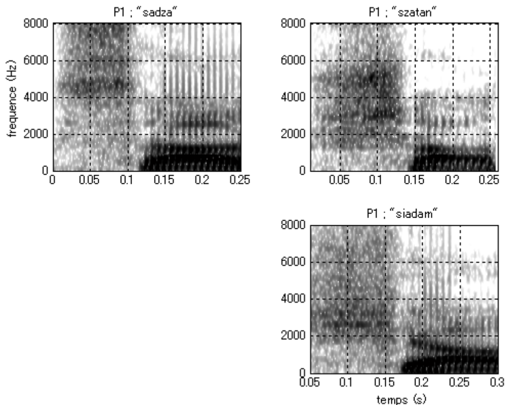
Figure 33. Spectrogrammes des séquences [sɔ] (en haut à gauche), [ʃɔ] (en haut à droite) et [cɔ] (en bas à droite) extraits respectivement des mos « sadza », « szatan » et « siadam ».
