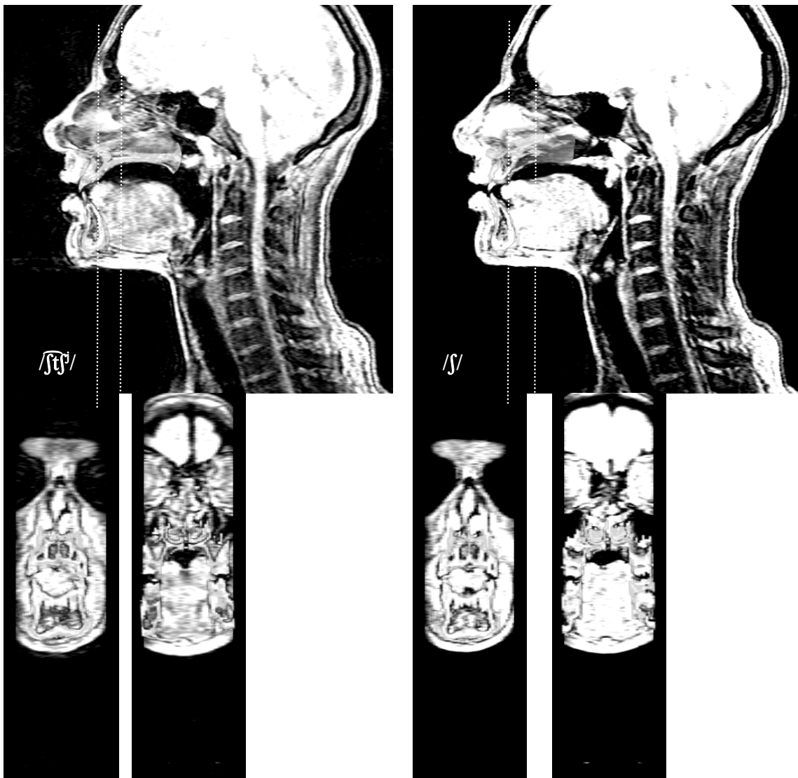
Figure 161. Coupes médio-sagittales (haut) et coronales (bas) des données IRM de la locutrice R complétées des dents. A gauche, /ʃtʃ/ ; à droite, /ʃ/. Les lignes pointillées blanches sur les profils sagittaux indiquent l'emplacement approximatif des coupes coronales.
