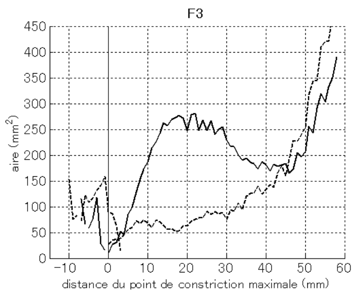
Figure 107. Fonctions d'aire de /s/ (lignes pleines) et /ʃ/ (lignes discontinues) ; mesures effectuées sur les coupes coronales perpendiculaires aux images d'origine.
