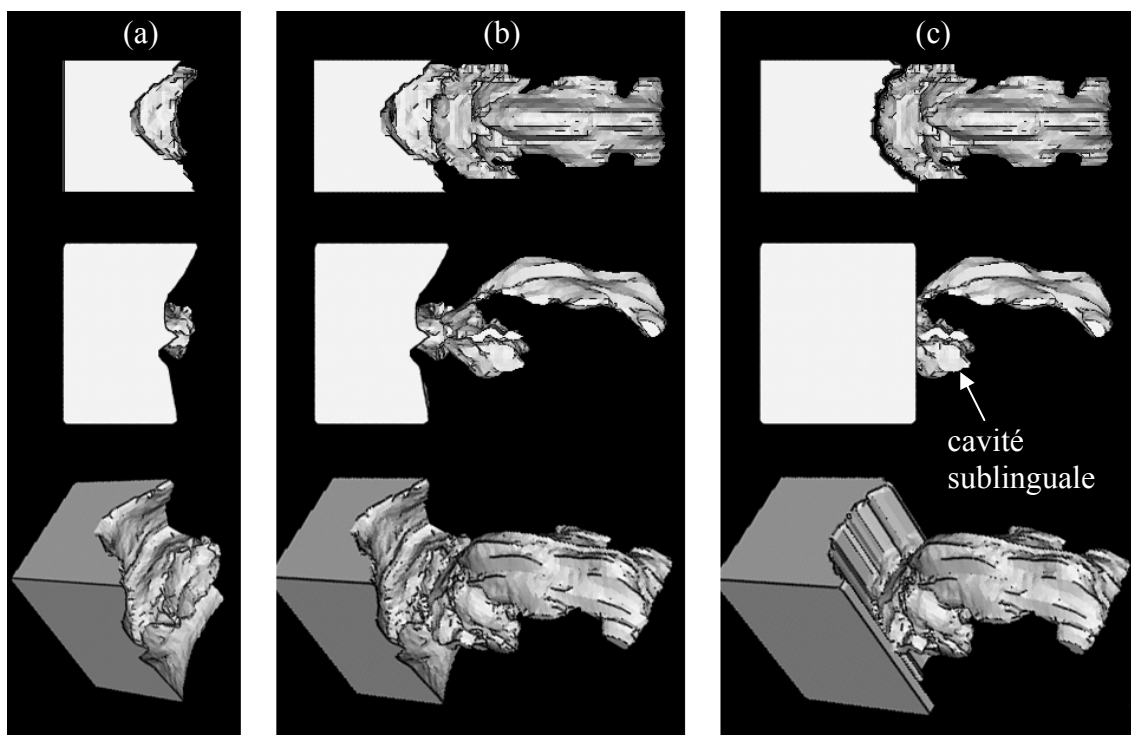
Figure 95. Conduits vocaux des sibilantes Fr1 /ʃ/ (haut) et P1 /ʒ/ (bas) ; (a) les lèvres seulement, (b) original (identiques à la Figure 92), et (c) sans les lèvres. A l'intérieur
