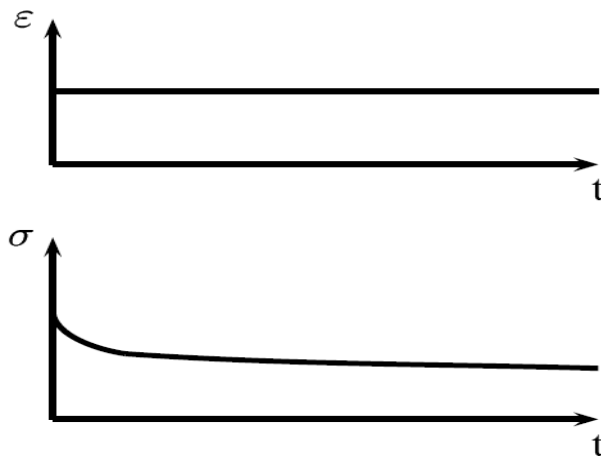
FIGURE 3.24: Déformation et contrainte lors d'un essai de relaxation.
