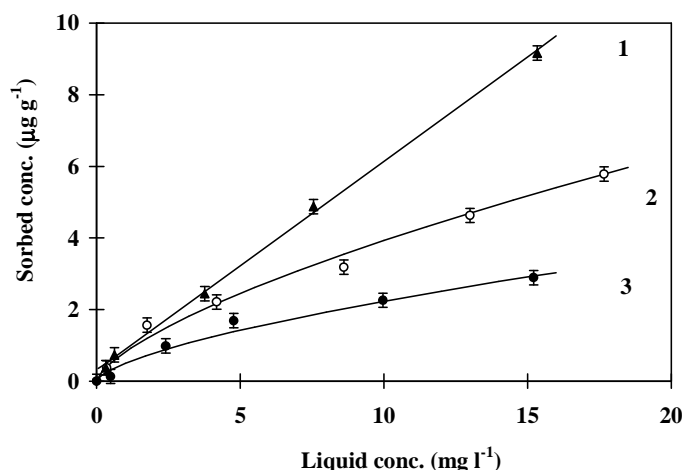
Figure 20 : Isothermes d'adsorption du dinosèbe seul (▲), en présence de 2,4 Dinitrophénol (o) ou en présence de 2,4DNP, DNOC et DNTB (●). Les isothermes sont modélisées avec l'Eq.1 (1) ou avec l'Eq. 6 (modèle de Freundlich) (2) et (3). (Martins and Mermoud 1998).
