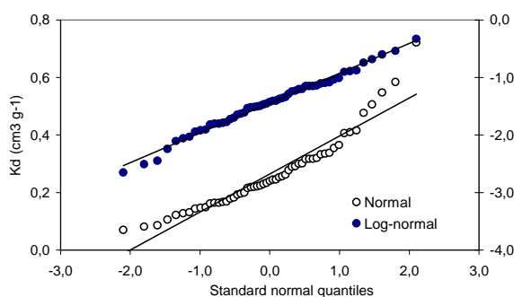
Figure 25 : Distribution statistique normale et log-normale des valeurs de K_D de l'atrazine et du dinoseb mesurées sur des échantillons de sol alluvial limoneux prélevés à différentes profondeurs et sur 3 profils de sols distants de 50cm (Zhang 2003)
