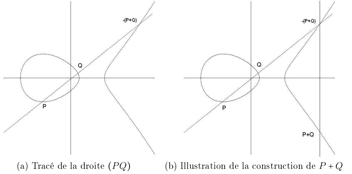
FIGURE I.2 – Loi de groupe sur les courbes elliptiques.
