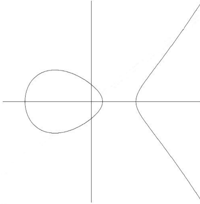
FIGURE I.1 – Exemple de courbe elliptique sur \mathbb{R} .
