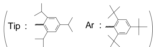
Schéma 1 : synthèse de ArP=C=Si(Ph)Tip
