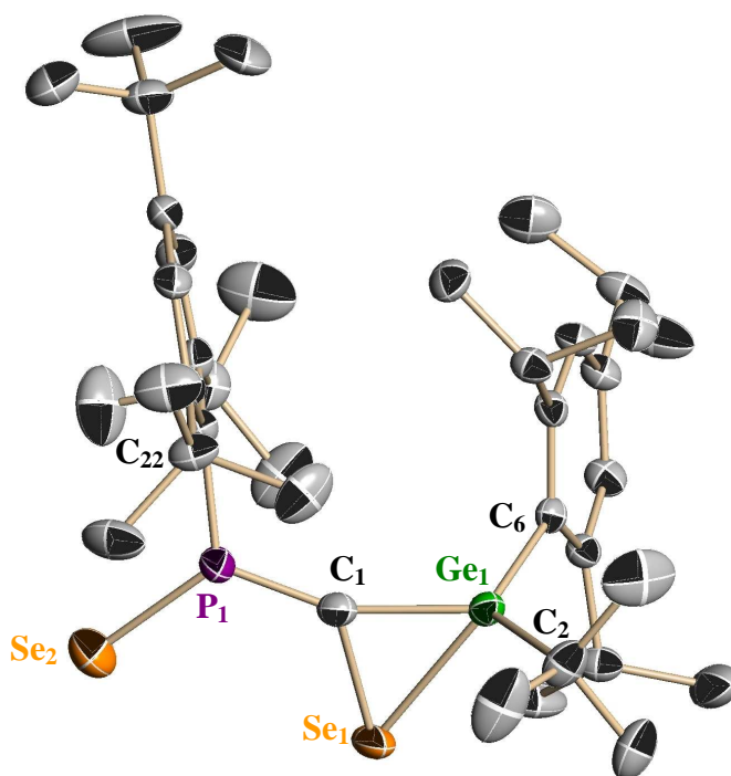
Fig 4. Structure moléculaire du méthylènesélénoxophosphorane 18 : ellipsoïdes tracés à 50% de probabilité. Les atomes d'hydrogène ont été omis pour rendre l'image plus claire.
