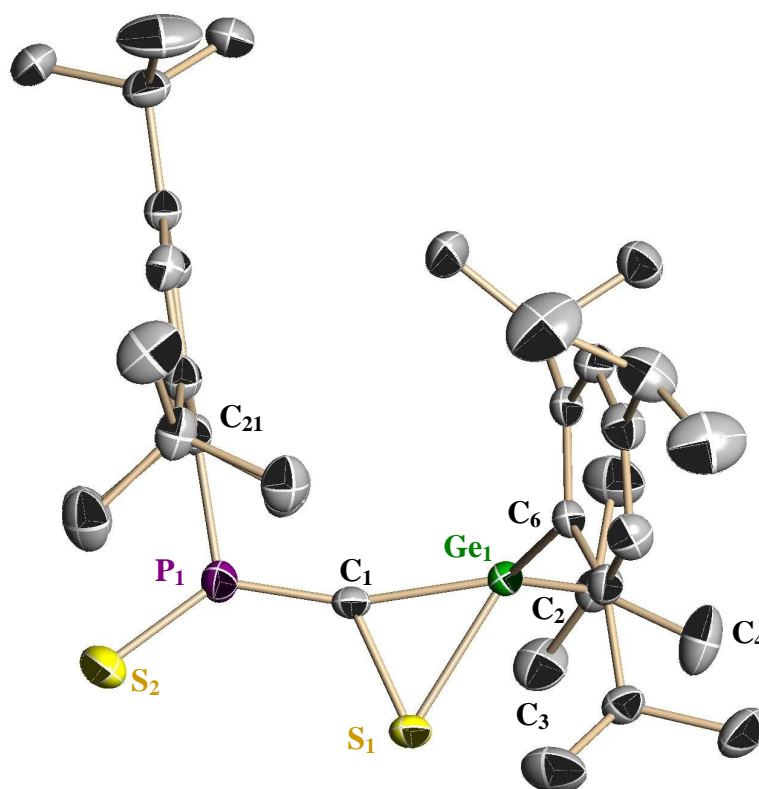
Fig 1. Méthyléthioxyphosphorane 12 : ellipsoïdes tracés à 50% de probabilité. Les atomes d'hydrogène ont été omis pour rendre l'image plus claire.
