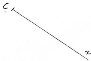
demi-droite [Cx)
