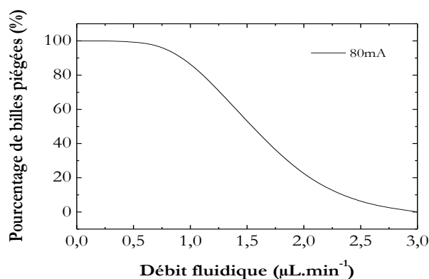
Figure 4.29 Courbe montrant l'influence de la vitesse d'écoulement du fluide sur l'efficacité de piégeage. Bobine carrée, N=5 et I=80\text{mA} .
