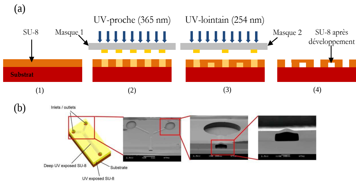
Figure 1.18 Réalisation de structures microfluidiques à l'aide d'une méthode à double insolation de la couche de SU-8 : (a) déroulement du protocole et (b) quelques exemples de réalisations.
