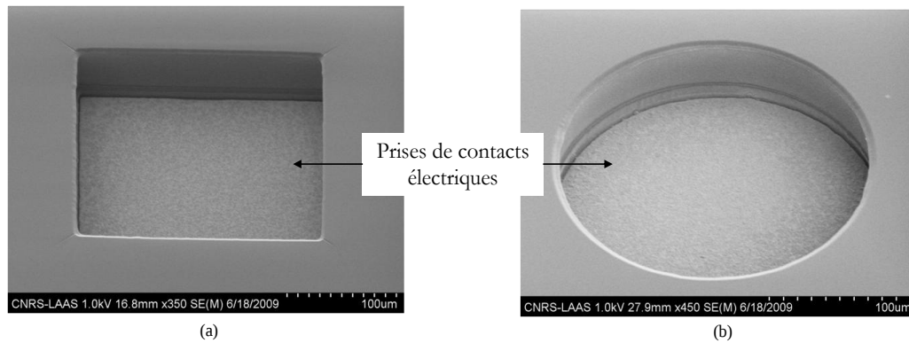
Figure 3.38 Photos montrant les fonds des ouvertures des contacts électriques après planarisation et encapsulation du microactionneur magnétique. (a) Prise de contact carrée et (b) prise de contact circulaire.
