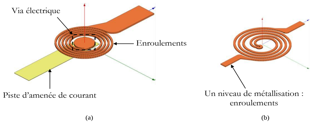
Figure 3.22 Deux approches technologiques différentes: (a) microbobine de type spirale et (b) microbobine de type méandre.
