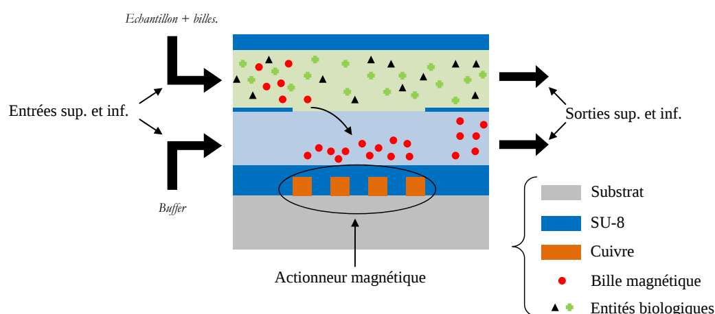
Figure 4.38 Schéma de principe d'un système magnéto-fluidique tridimensionnel pour la manipulation de billes magnétiques.
