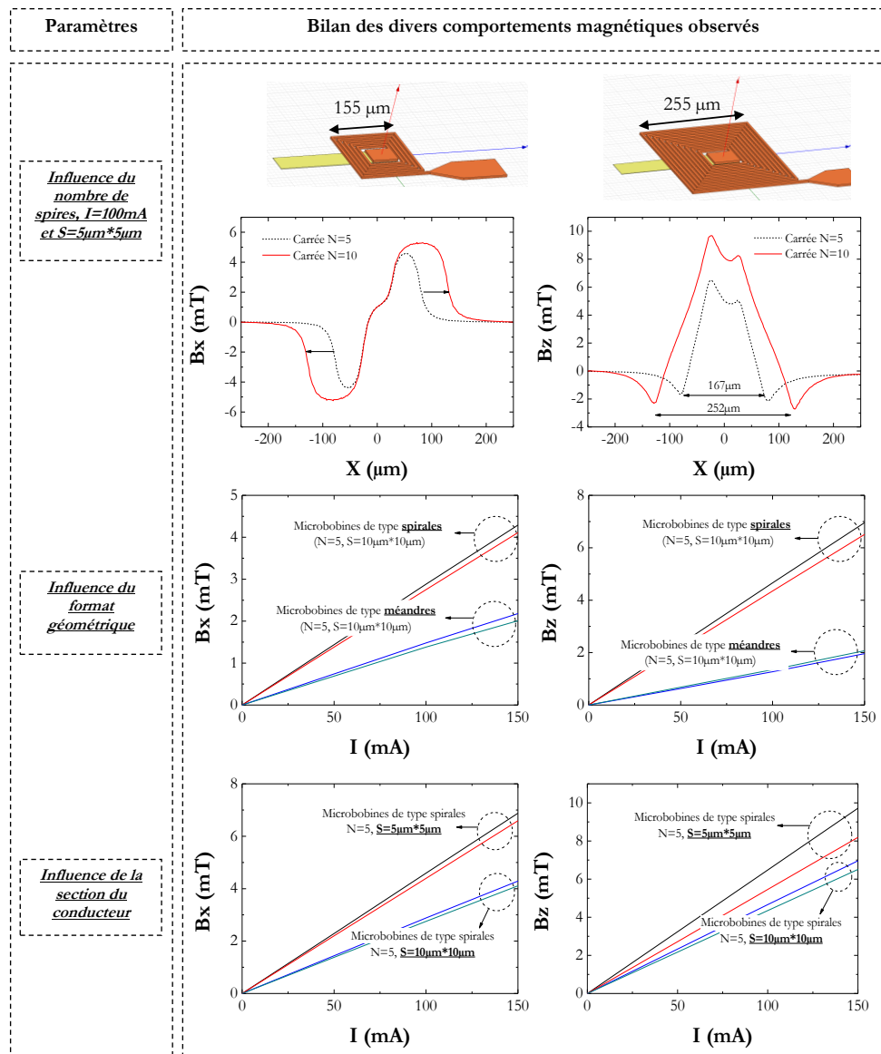
Figure 2.12 Bilan des divers comportements magnétiques observés.
