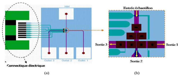
Figure 4.31 Réalisation d'un microsystème fluidique intégrant un réseau de microactionneurs magnétiques pour l'aiguillage de billes magnétiques : (a) vue globale du microsystème ; (b) observation détaillée des microbobines.
