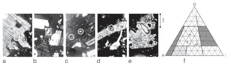
Figura 2. Fotografía de las secciones delgadas en nicoles cruzados (NX). Objetivo 0:0,12x. Ocular: 12,5x para las secciones FCT-1 al FCT 5 (a-e); f: diagrama ternario para la clasificación de rocas volcánicas según Streckeisen (1979), elaborado en Matlab y modificado de Middleton (1999). Ver Tabla I.
