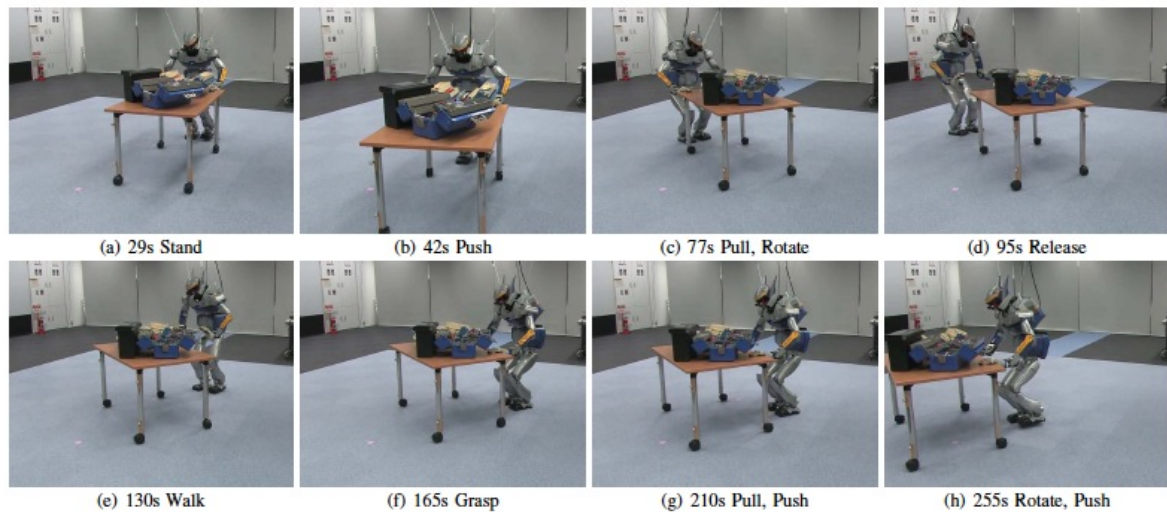
FIGURE 2.26 – de [Stilman et al. 2008] Images d'une seule et même expérimentation de télé-opération. Nous pouvons y voir diverses manipulations d'une table sur roulette recouverte de 55kg de matériel.
