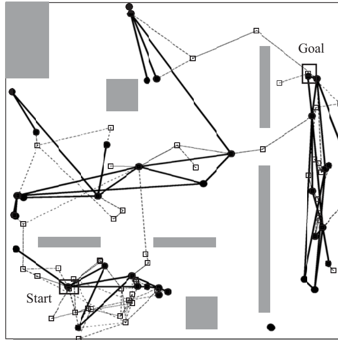
FIGURE 5.8 – Graphe de manipulation généré par la méthode proposée. Les fines lignes avec des cercles dérivent du graphe \mathcal{G}_{obj} initial de l'objet. Les fines lignes avec des carrés ont été additionnées par la méthode de planification par diffusion RRT.
