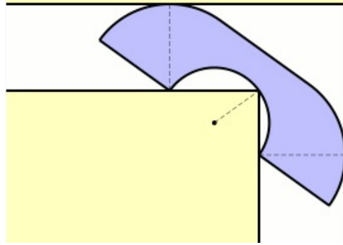
FIGURE 2.1 – de [Stewart 2004] Exemple de solution proposée J. Hammersley au problème du sofa formulé par L. Moser
