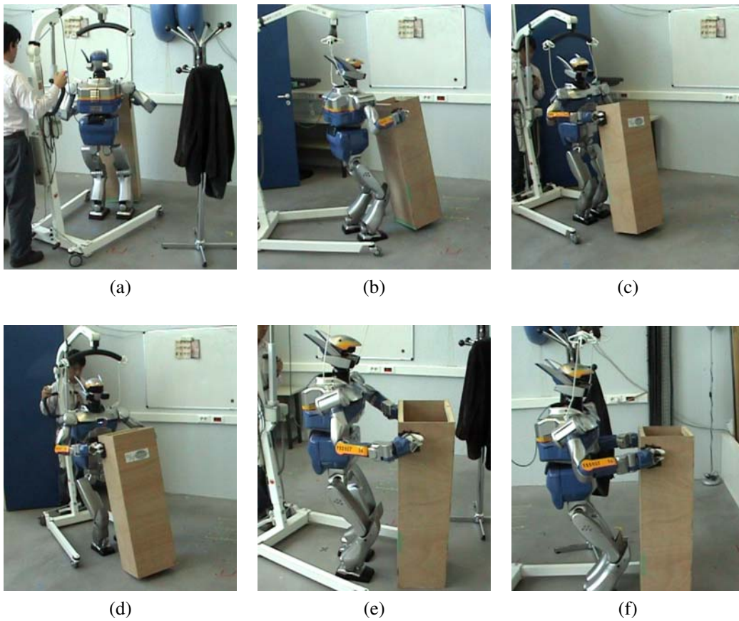
FIGURE 4.21 – Résultats d’expérimentations. départ de la position initiale de l’objet (a) avec l’obstacle sur le côté droit. le robot manipule l’objet à reculons depuis le mur (b). Après un changement de direction vers l’avant (c), le robot continue de manipuler l’objet vers sa position finale tout en évitant l’obstacle (d-f).
