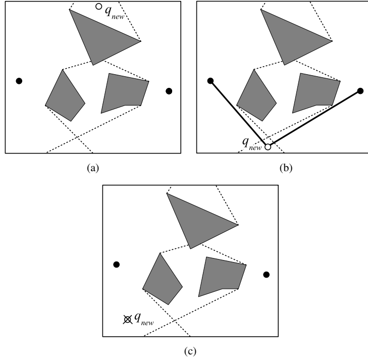
FIGURE 5.3 – Trois cas de la construction d'un graphe de PRM de visibilité.
