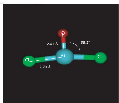
AtOCl 2 - (symétrie C 2v )
