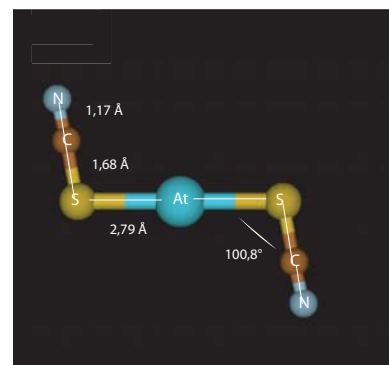
AtSCN 2 (symétrie C 2h )
