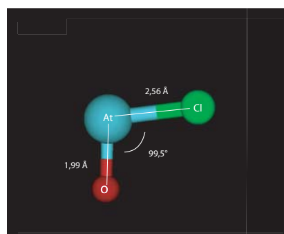
AtOCl (symétrie C s )
