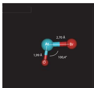
AtOBr (symétrie C s )
