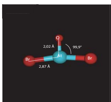
AtOBr 2 - (symétrie C 2v )
