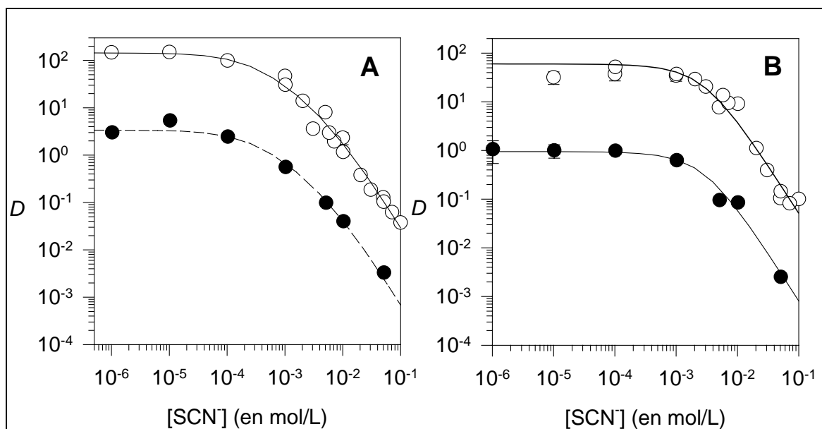
Figure 2: Variation du coefficient de partage D de \text{At}^+ (A) et \text{AtO}^+ (B) entre une phase aqueuse et organique (toluène \circ et hexane \bullet ) en fonction de la concentration en ion \text{SCN}^- .
