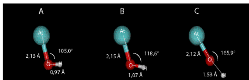
Figure 4: Evolution de la géométrie de \text{AtOH} de la phase gaz à la phase aqueuse au cours de calculs pseudo-relativistes B3LYP/mAVDZ utilisant le modèle de solvatation CPCM couplé aux cavités UAKS. La structure A est celle de l'espèce en phase gaz, la structure B représente une des premières étapes de l'optimisation de géométrie dans le modèle de solvant et la structure C est la géométrie optimum prévue par le calcul pour \text{At}(\text{OH}) en phase aqueuse.
