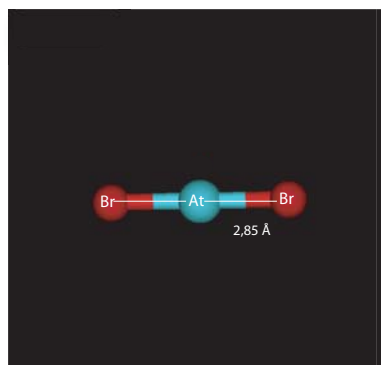
AtBr 2 (symétrie D ∞h )
