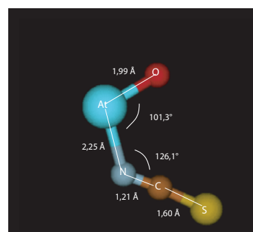
AtOSCN (symétrie C 1 )
