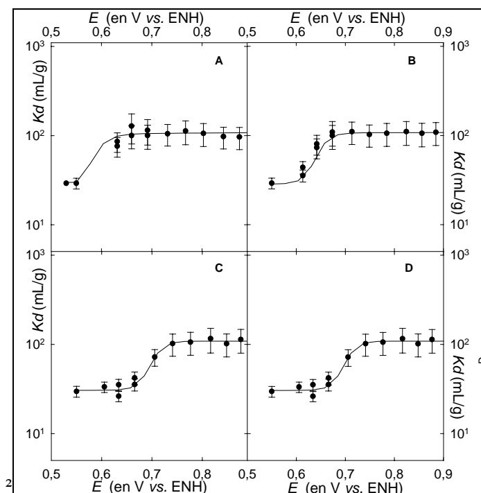
Figure 5: Etude du passage de l'espèce II vers l'espèce III dans le système aqueux/Dowex 50WX8. Le changement de potentiel est imposé par le couple redox \text{Fe}^{3+}/\text{Fe}^{2+} ( [\text{Fe}^{\text{n+}}]_{\text{total}} = 0,1 \text{ mol/L} ). A: [\text{HClO}_4] = 0,01 \text{ mol/L} , B: [\text{HClO}_4] = 0,013 \text{ mol/L} , C: [\text{HClO}_4] = 0,1 \text{ mol/L} , D: [\text{HClO}_4] = 0,3 \text{ mol/L} .
