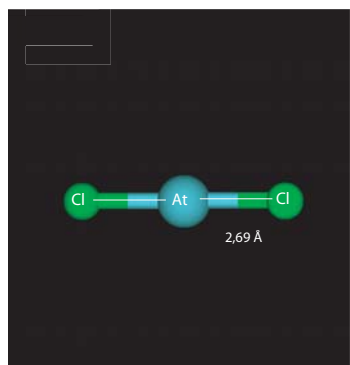
AtCl 2 (symétrie D ∞h )
