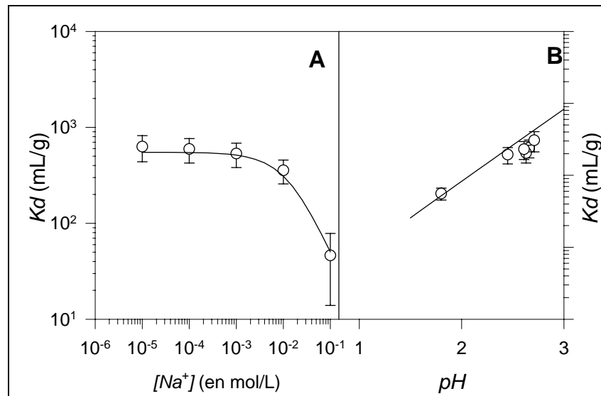
Figure 1: Variation du coefficient de partage K_d de \text{Na}^+ sur la résine Dowex-50WX8 en fonction de la concentration en \text{Na}^+ ( \text{pH} = 1,8 et m/V = 5 g/L) (A) et du \text{pH} (avec [\text{NaCl}] = 1 \cdot 10^{-3} mol/L et m/V = 5 g/L) (B).
