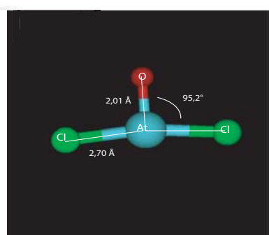
AtOCl 2 - (symétrie C 2v )
