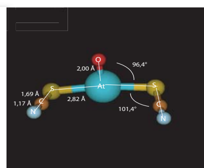
AtO(SCN) 2 - (symétrie C s )
