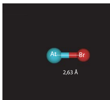
AtBr (symétrie C_{\infty v} )
