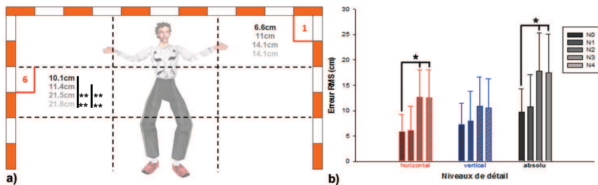
Fig. 3.11 - Erreurs RMS (en horizontal, vertical et absolu) entre la trajectoire du centre de masse de l'avant-bras pour le niveau N0 et cette même trajectoire pour les niveaux N1, N2, N3 et N4 (* : p < 0.05 ; ** : p < 0.01 ). Seules les erreurs en absolu sont représentées dans le but de handball.
