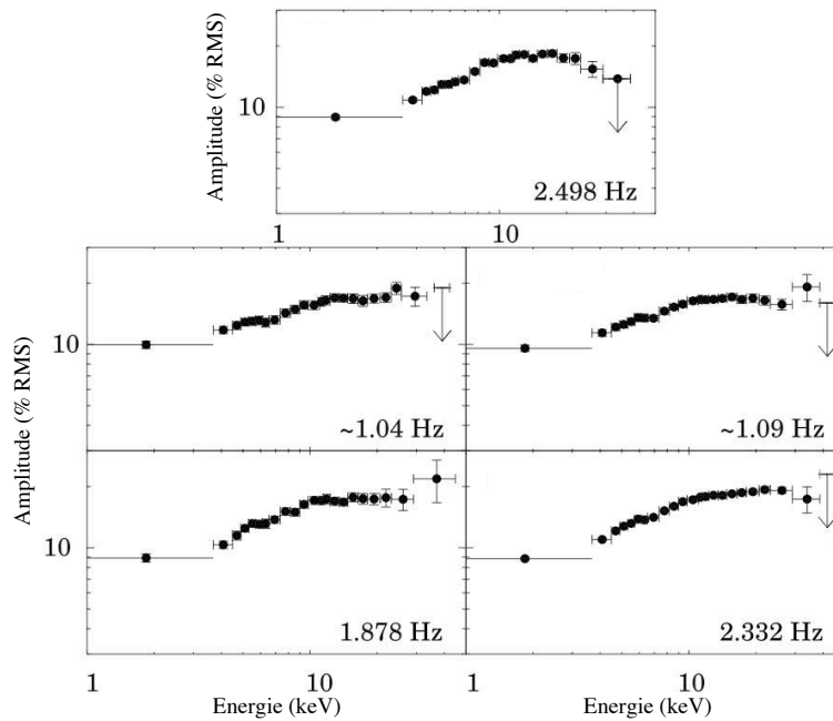
FIG. 12.2 – Spectres en énergie des 5 QPO de fréquences différentes obtenus lors des observations de classe \chi de la première année de notre suivis simultanée avec INTEGRAL . Adapté de Rodriguez et al. (2004a).
