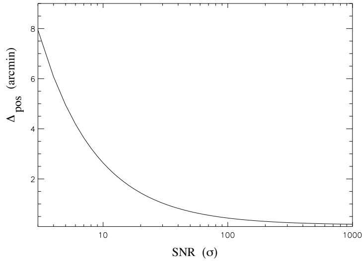
FIG. 2.2 – Dépendance de la précision de localisation d'IBIS en fonction du rapport signal à bruit de la détection, obtenue à partir d'un ajustement des données (Gros et al. 2003).
