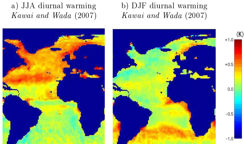
FIG. 2.12 – Amplitude moyenne du réchauffement diurne pour a) l'été (juin - août) et b) l'hiver boréal (décembre - février). Tiré de Kawai and Wada (2007)
