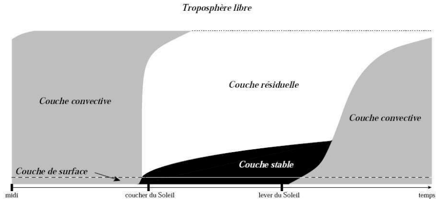
FIG. 1.6 – Evolution schématisée de la couche limite par temps calme et non perturbé. Cette figure est tirée de l'ouvrage de Stull (1988)
